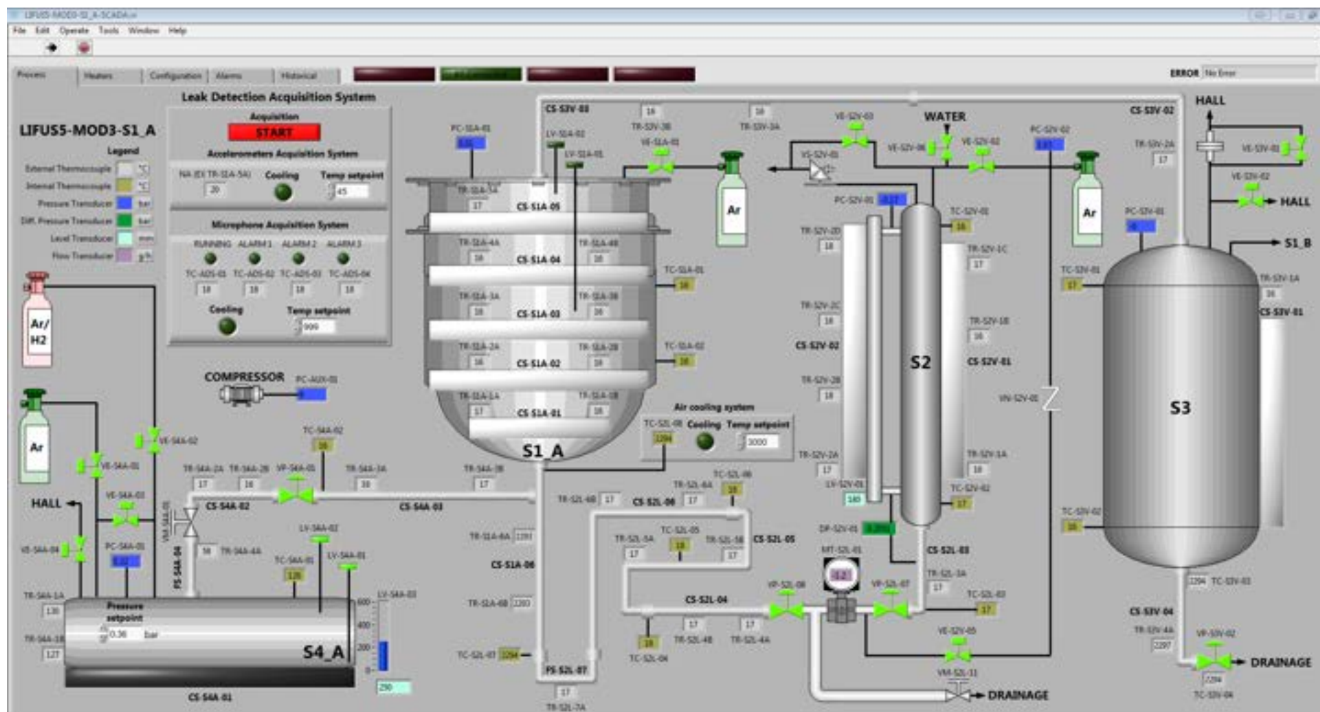
Fig. 2—11 – LIFUS5/Mod3 synoptic.
