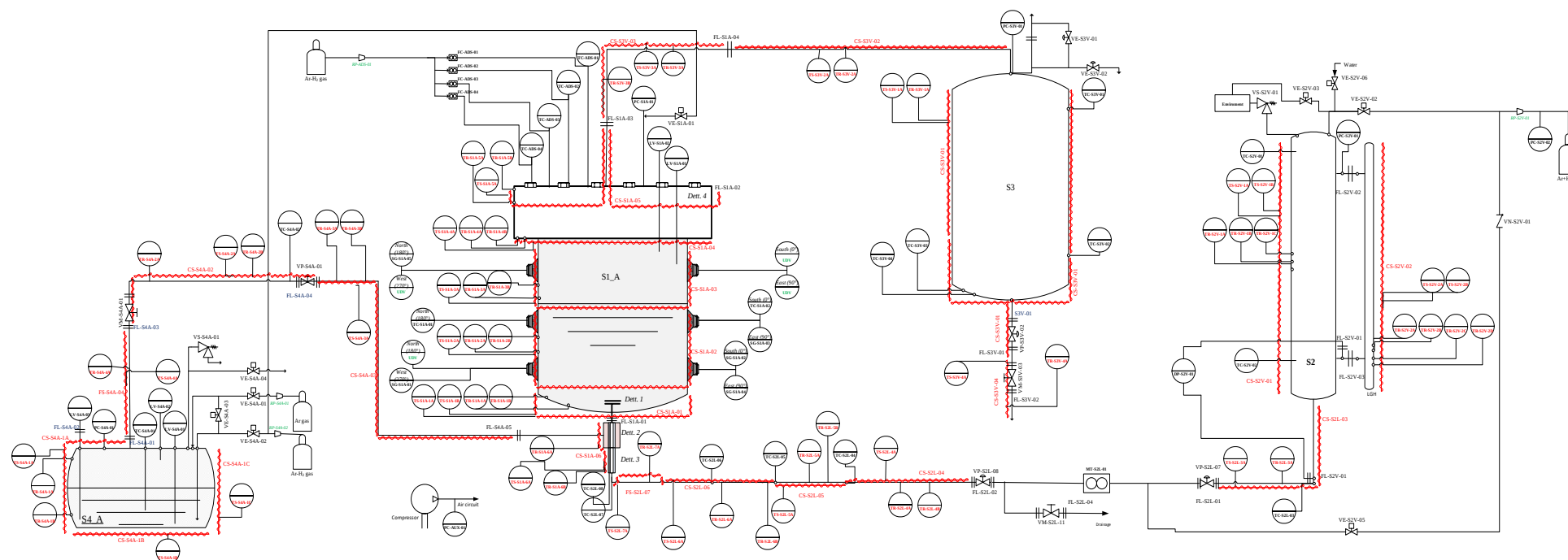
Fig. 2—10 – LIFUS5/Mod3 facility
