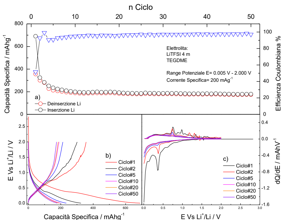
Figura 21 Comportamento elettrochimico della cella Sn/RGO_ENEA alla corrente specifica di 200 mA g -1 con elettrolita a base LiTFSI - TEGDME
