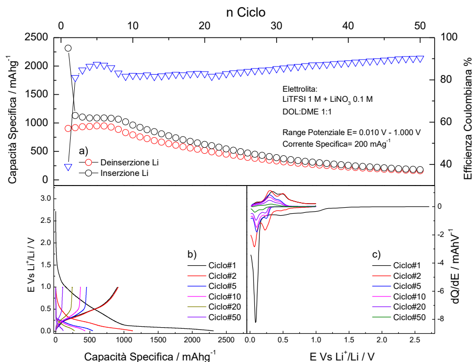
Figura 14. Comportamento elettrochimico della cella Si/RGO con elettrolita LiTFSI+LiNO 3 – DOL:DME alla corrente specifica di 200 \text{ mA} \text{ g}^{-1} .
