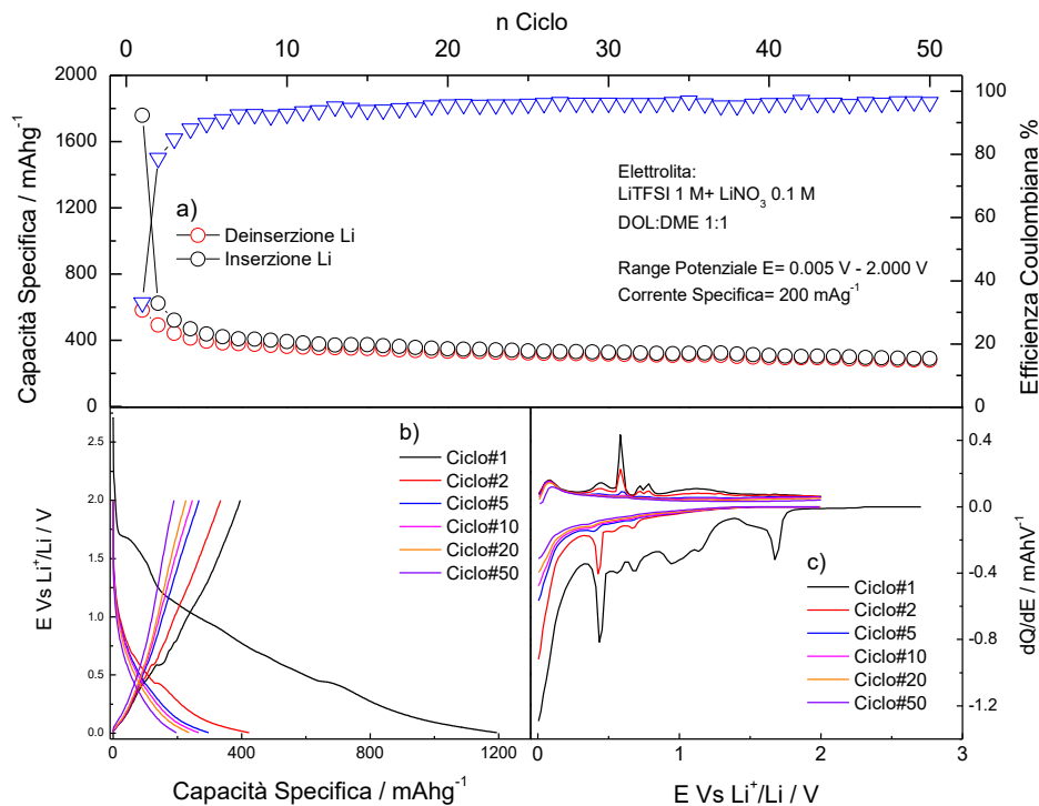
Figura 25 Comportamento elettrochimico della cella Sn/RGO_ENEA alla corrente specifica di 200 \text{ mA g}^{-1} con elettrolita a base LiTFSI 1 M + \text{LiNO}_3 0.1 M – DOL:DME
