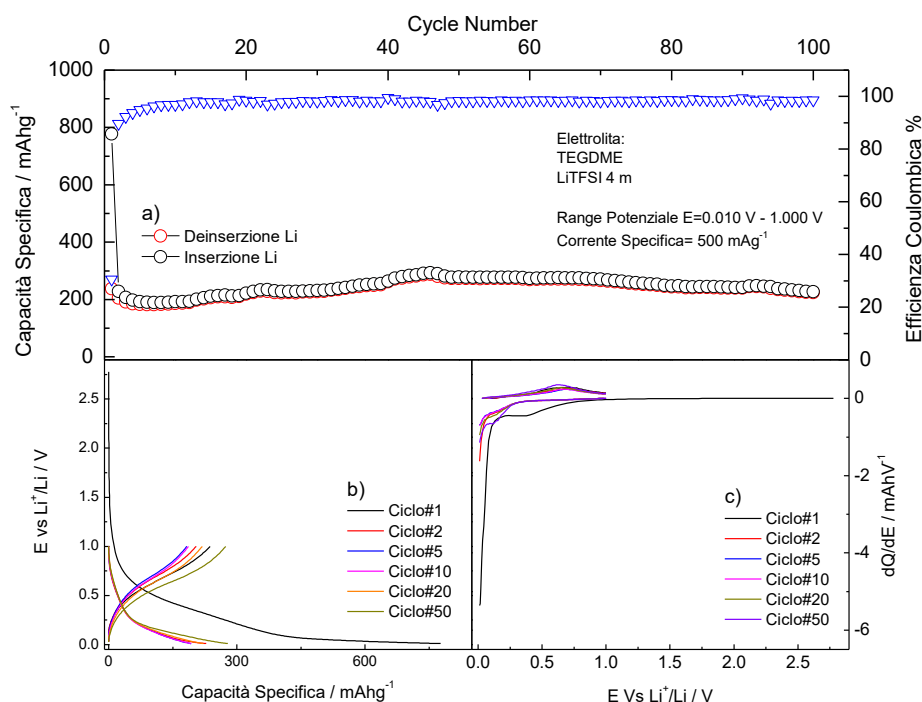
Figura 7. Comportamento elettrochimico della cella Si/RGO con elettrolita LiTFSI-TEGDME alla corrente specifica di 500 \text{ mA g}^{-1} .
