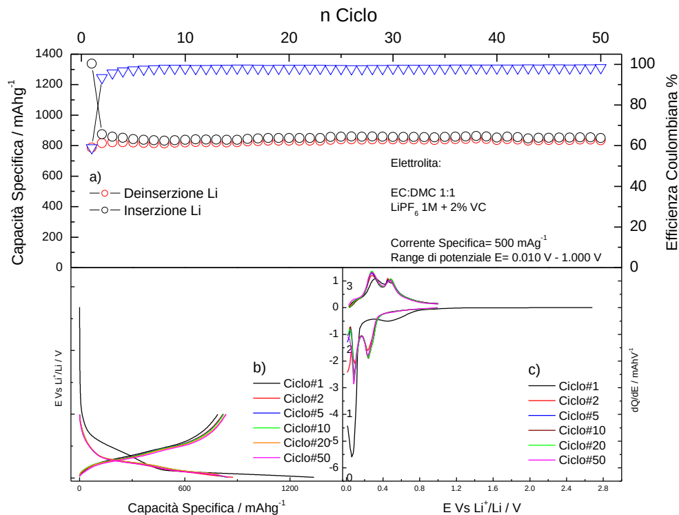
Figura 5. Comportamento elettrochimico della cella Si/RGO alla corrente specifica di 500 mA g -1 con elettrolita LiPF 6 /VC in EC:DMC 1:1
