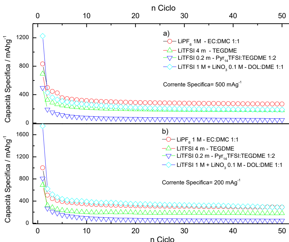
Figura 27 Confronto prestazioni elettrochimiche di elettrodi Sn/RGO con differenti elettroliti: a) Corrente Specifica 500 mA g -1 b) Corrente Specifica 200 mA g -1
