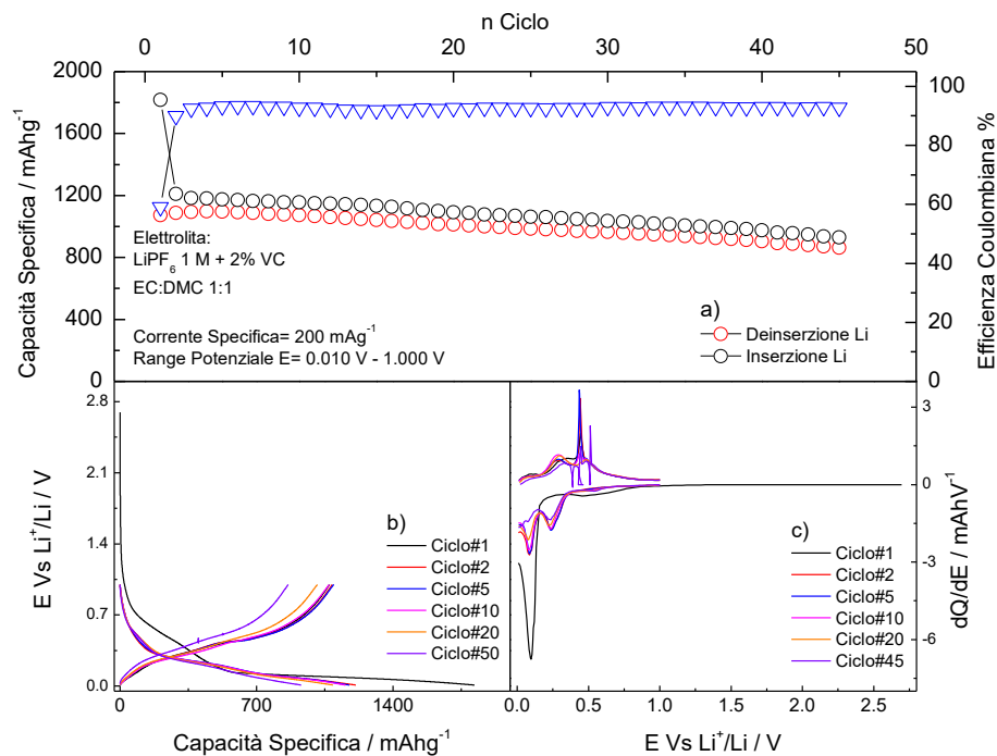
Figura 6. Comportamento elettrochimico della cella Si/RGO alla corrente specifica di 500 mA g -1 con elettrolita LiPF 6 /VC in EC:DMC 1:1
