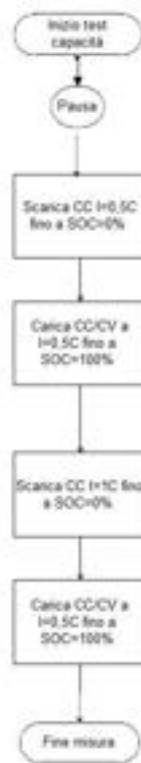
Figura 7:Flowchart del test di capacità
