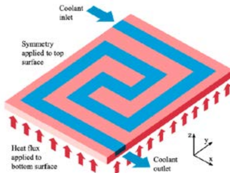
Figura 30. Piastra con liquido di raffreddamento
