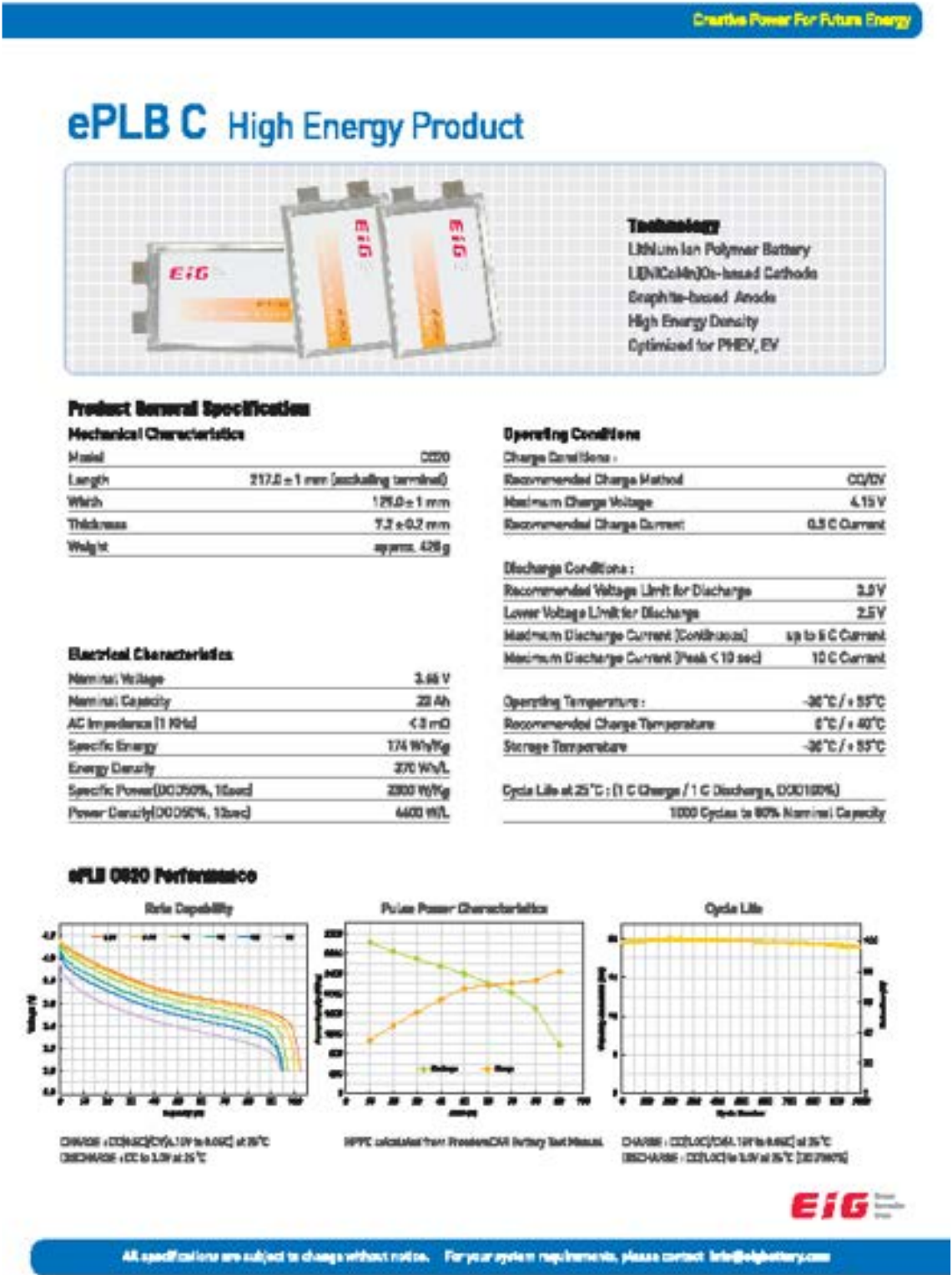
Figura 18. Caratteristiche delle celle EIG 20 Ah
