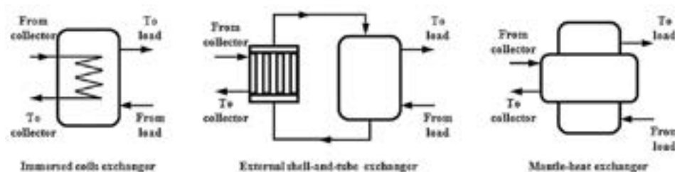
Fig. 3. Tipiche configurazioni per scambiatori di calore accoppiati a serbatoio di accumulo termico ad acqua (Han et al. [10]).
