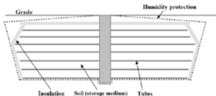
Fig. 8. Sistema di accumulo termico stagionale a tubi orizzontali dell'impianto Vulturno.
