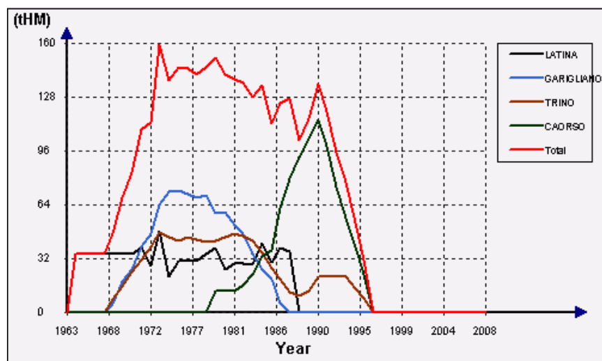
Figura 25: SF inventory in piscina prima del reprocessamento
