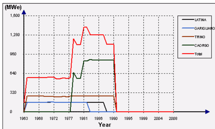
Figura 19: Capacità nucleare installata in Italia nel periodo 1963-1990
