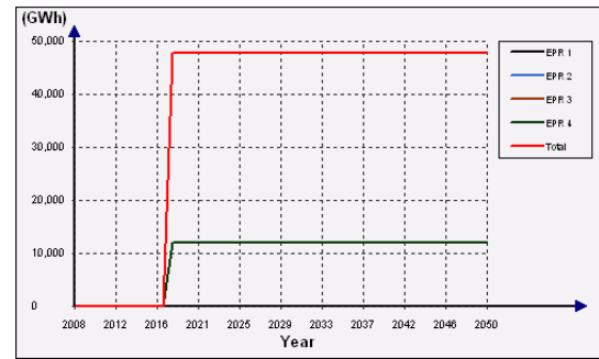
Figura 29: Elettricità prodotta annualmente scenario ONE
