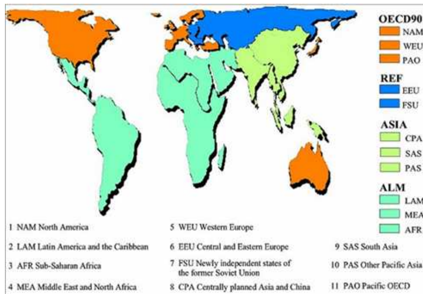
Figura 2: Suddivisione del mondo in 11 regioni (IIASA), raggruppate poi nelle 4 macro-regioni considerate dall'IPCC [1]
