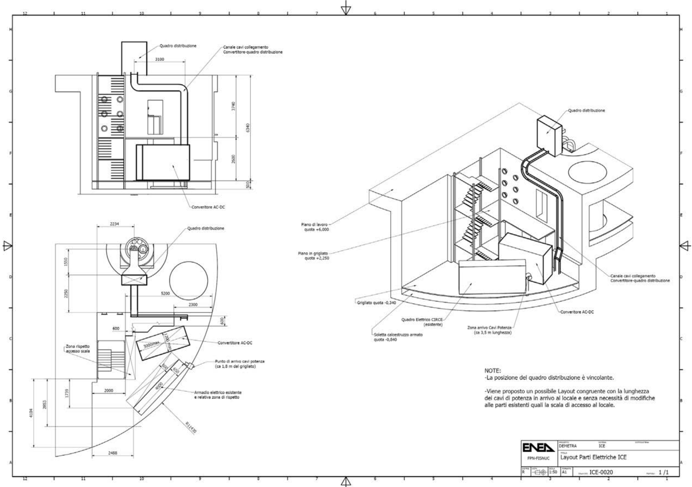
Allegato 1: ICE-0020 Layout Parti Elettriche ICE
