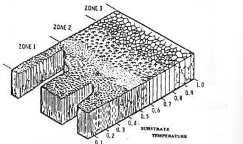
Figura 2.4 - Modello structure zone di crescita di un film (da rif. 13)
