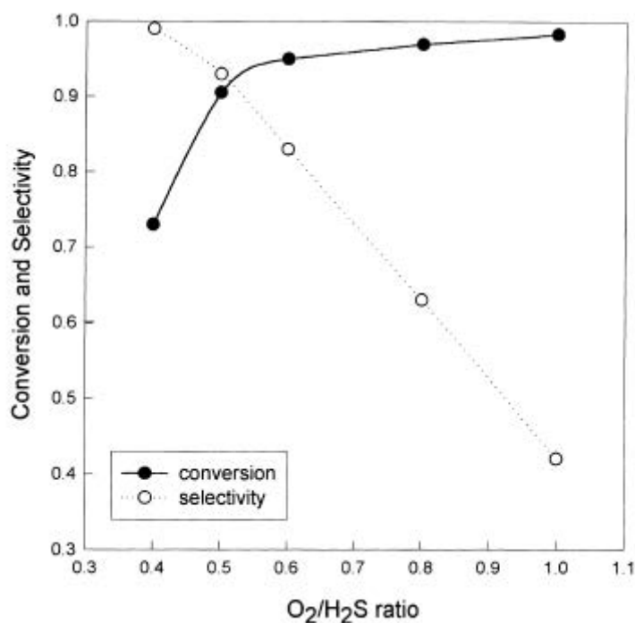
Fig. 1: Effetto di \text{O}_2/\text{H}_2\text{S} sulla conversione di \text{H}_2\text{S} e selettività a zolfo.
