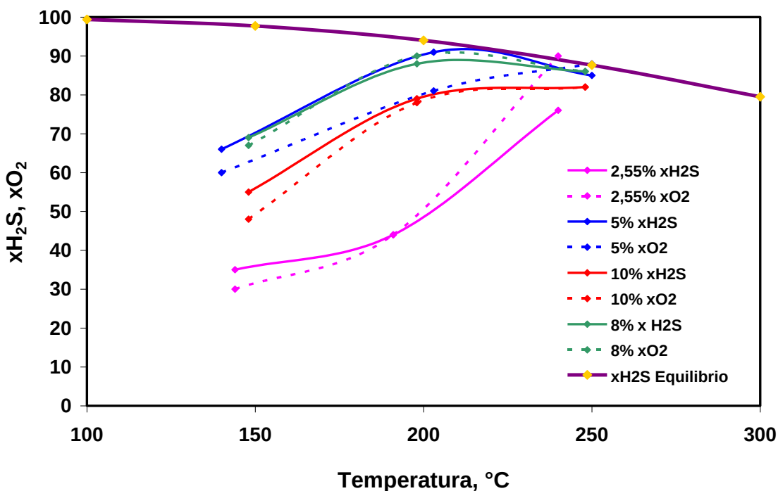
Fig. 18: Andamento della conversione di \text{H}_2\text{S} e \text{O}_2 nell'intervallo T=150-250^\circ\text{C} in funzione del carico di vanadio.
