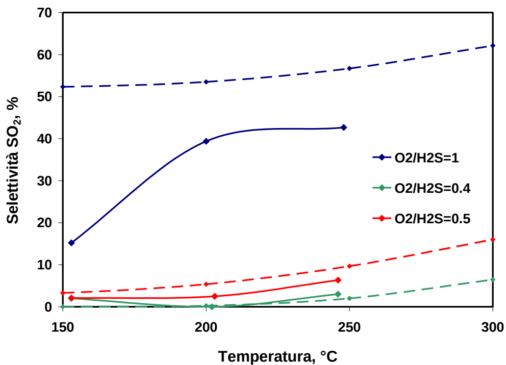
Fig. 22: Andamento della selettività ad \text{SO}_2 al variare della temperatura e in funzione di \text{O}_2/\text{H}_2\text{S} .
