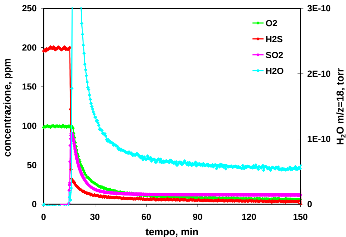
Fig. 32 Prova di attività condotta sul monolite catalizzato a base di V_2O_5 (campione 2) T=205^\circ\text{C} .
