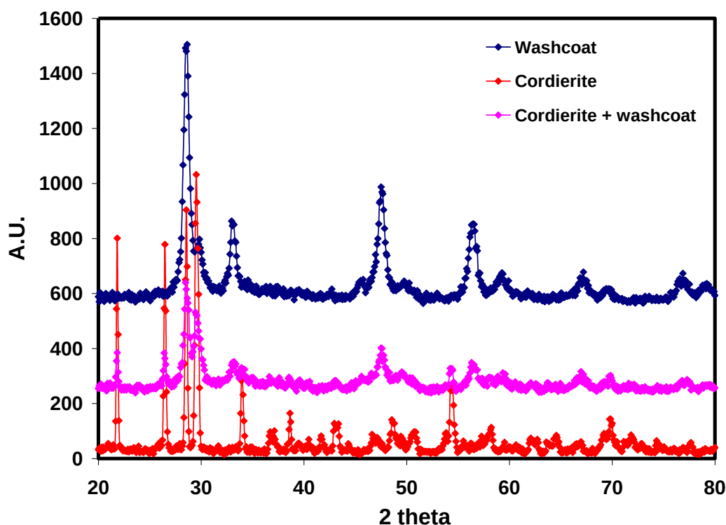
Fig. 26: XRD della cordierite, washcoat e cordierite con washcoat.
