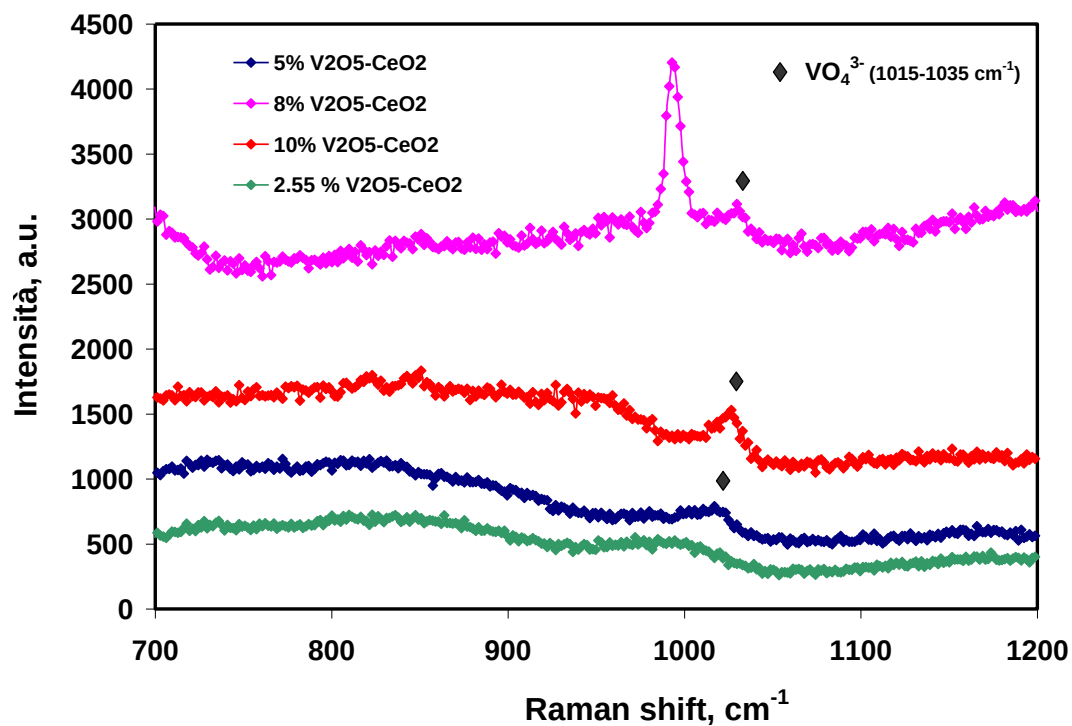
Fig. 16: Spettri Raman del supporto e dei catalizzatori V-Ce nell'intervallo 700-1200 \text{cm}^{-1} .
