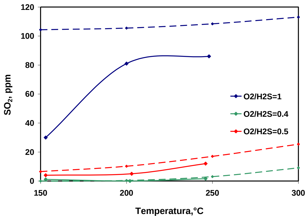
Fig. 21: Andamento della concentrazione di \text{SO}_2 al variare della temperatura e in funzione del rapporto \text{O}_2/\text{H}_2\text{S} .
