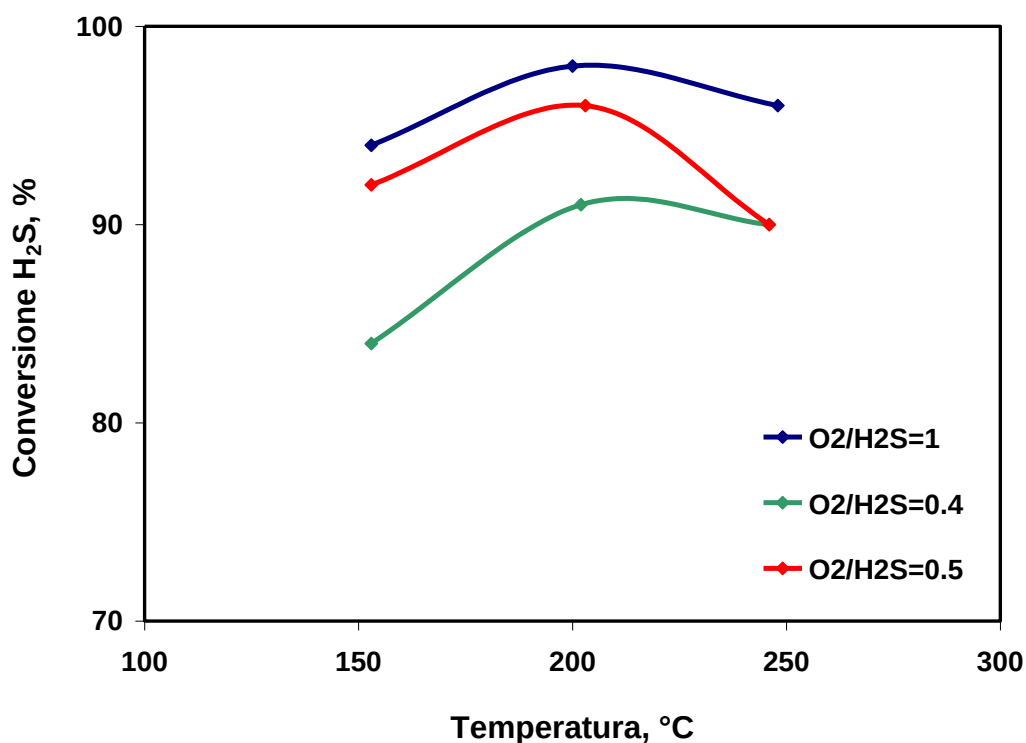
Fig. 20: Conversione di H 2 S al variare della temperatura e in funzione del rapporto O 2 /H 2 S.
