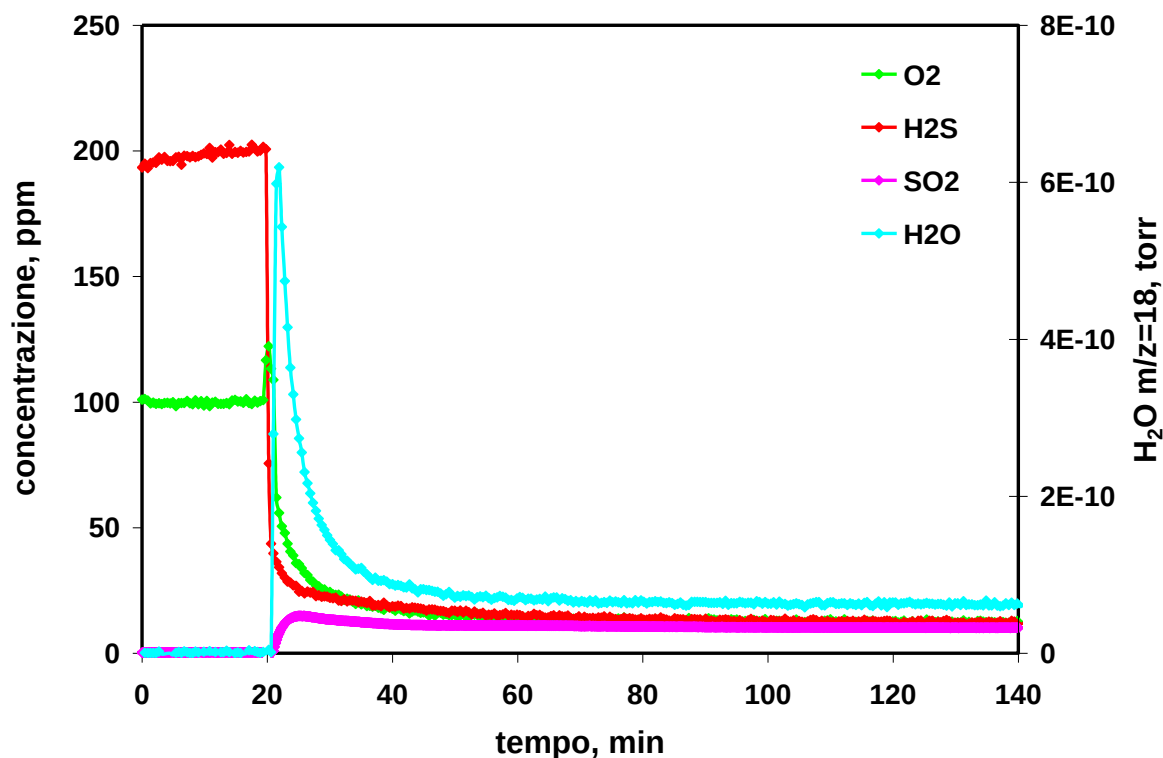
Fig. 31: Prova di attività condotta sul monolite catalizzato a base di \text{V}_2\text{O}_5 (campione 1) a T=205^{\circ}\text{C} .
