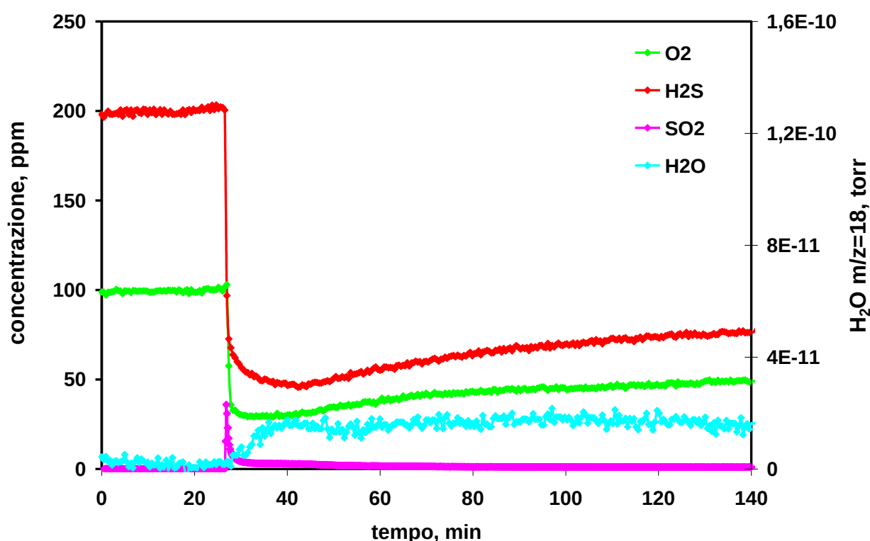
Fig. 30: Prova di attività condotta sul monolite catalizzato a base di \text{V}_2\text{O}_5 (campione 1) a T=160^\circ\text{C} .
