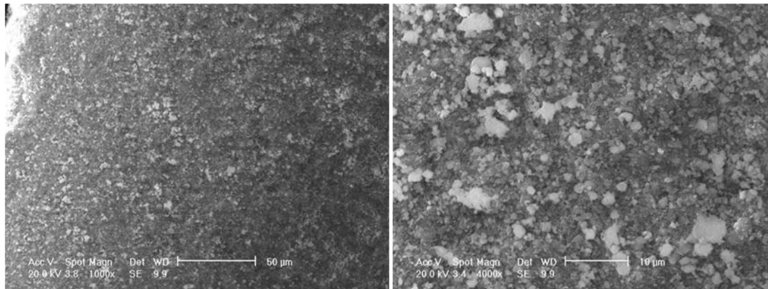
Figura 4A Superficie esterna HT a base di calcio promossa con \text{K}_2\text{CO}_3 post trattamento termico
