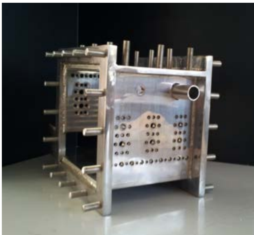
Figura 2: Prototipo TVC.
