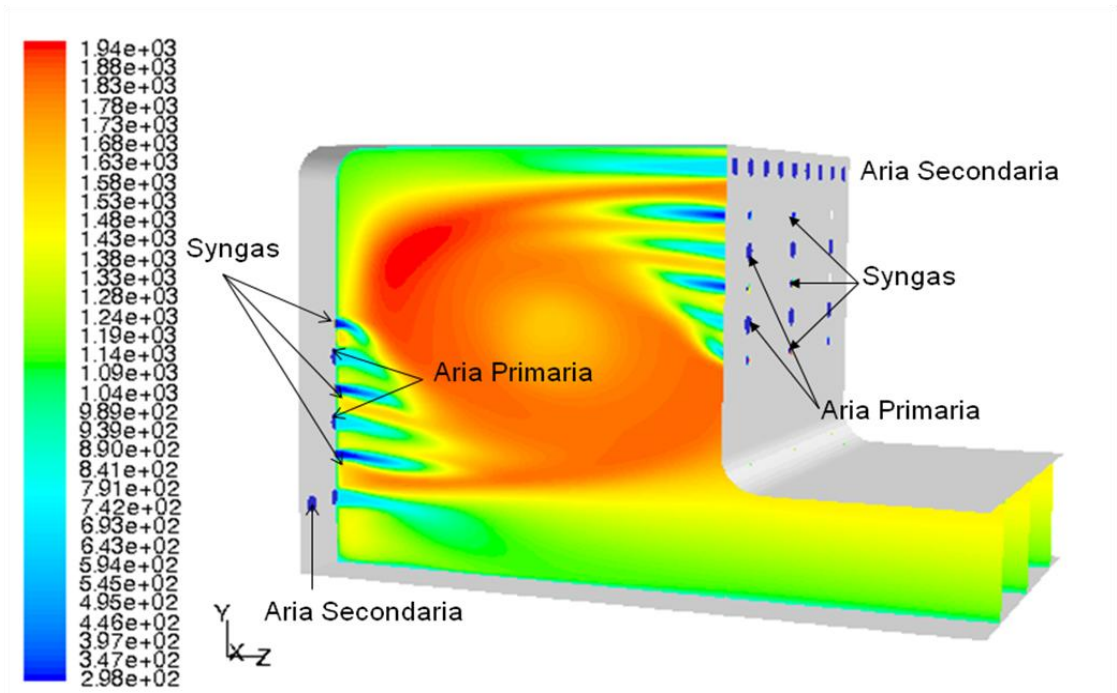
Figura 1: Prototipo TVC e campo di temperature [1].
