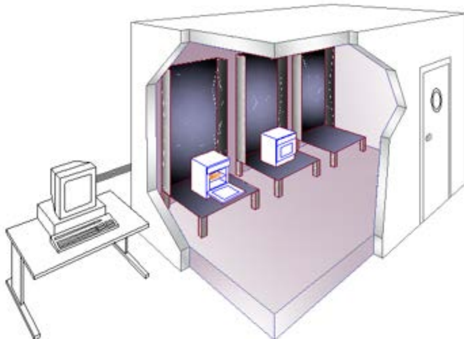
Figura 4: Schema della camera climatica per la prove sui forni elettrici domestici (FIRELAB).
