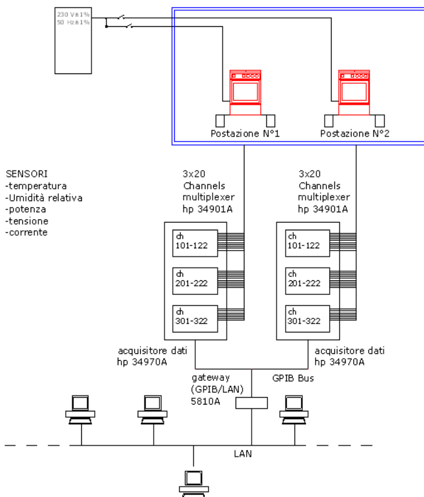
Figura 7: Schema del sistema di acquisizione dati del laboratorio FIRELAB.
