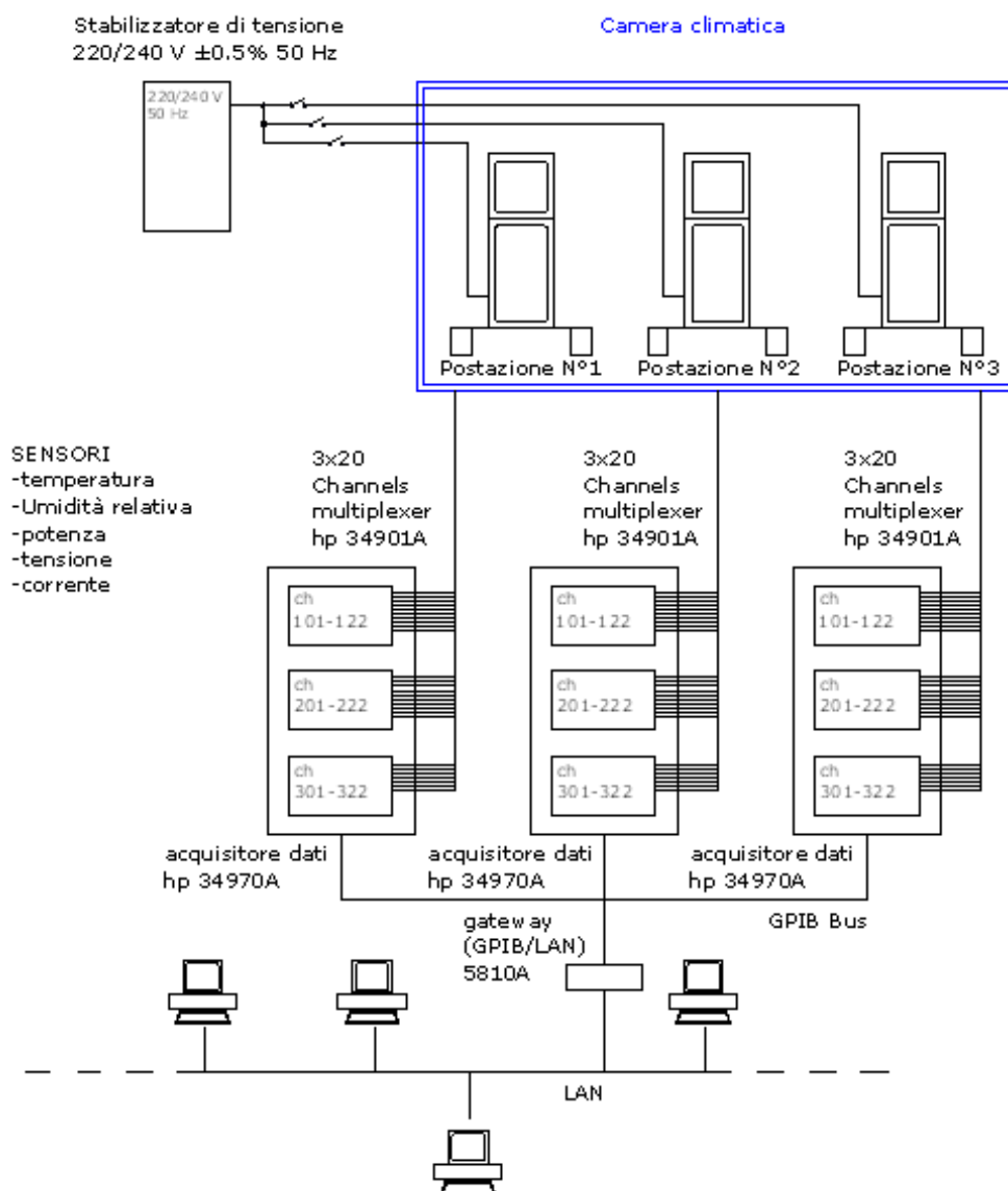
Figura 11: Schema del sistema di acquisizione dati del laboratorio ICELAB
