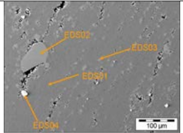
10-morfologia -SEM- BSE – 20 kV- 250X
