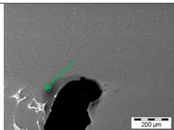
14 - IQ- SEM - BSE - 20 kV -125X
