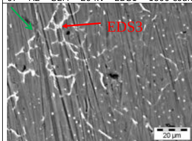
09 - A2- SEM - BSE - 20 kV - 1000X
