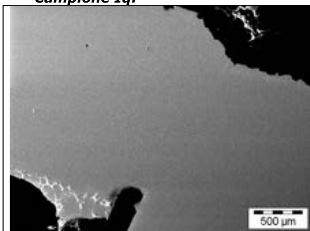
13 - IQ- SEM - BSE - 20 kV -40X
