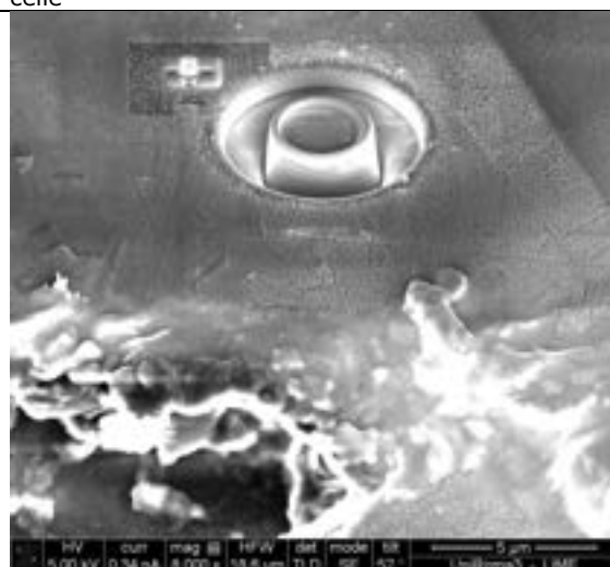
04 – immagine di dettaglio di una delle prove realizzate
