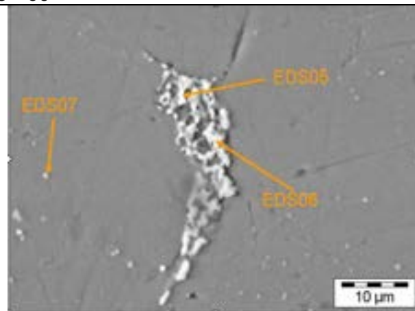
24- schiuma pannello AFS - SEM- BSE - 20 kV- 2000X
