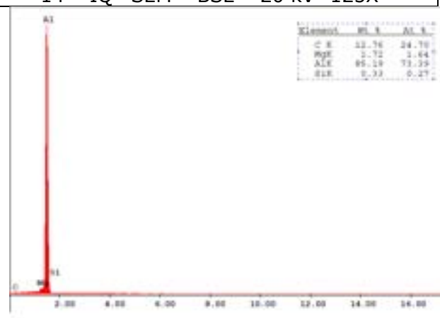
16- IQ - SEM - 20 kV - EDS6 - 1800 count
