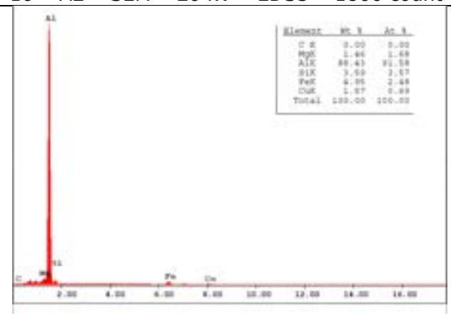
11- A2 - SEM - 20 kV - EDS4 - 1800 count
