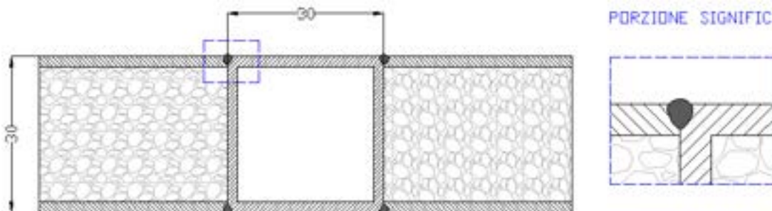
Figura 8: schema di prelievo dei campioni per microanalisi e durezza
