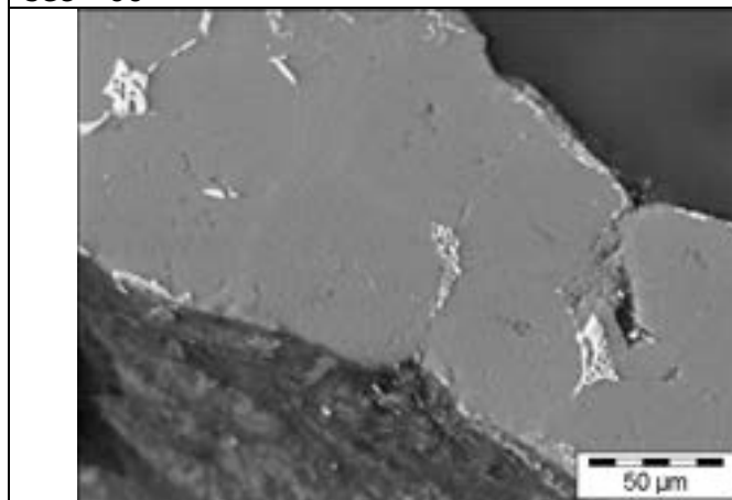
23- schiuma pannello AFS - SEM- BSE - 20 kV- 500X
