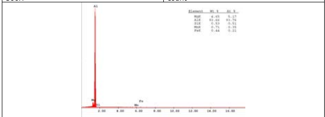
27- A8 - SEM - 20 kV - EDS13 - 1800 count
