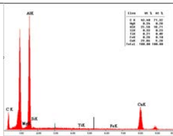
22-EDS 04 - SEM - 20kV - count 1900 - sec= 60
