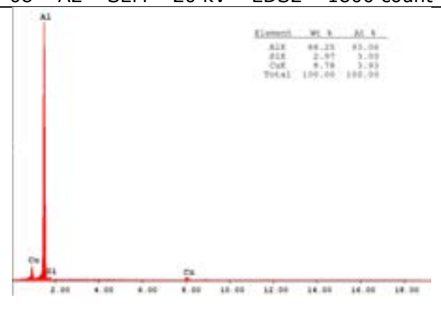
10 - A2 - SEM - 20 kV - EDS3 - 1800 count
