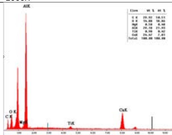
26-EDS 06 - SEM - 20kV - count 1900 - sec= 60
