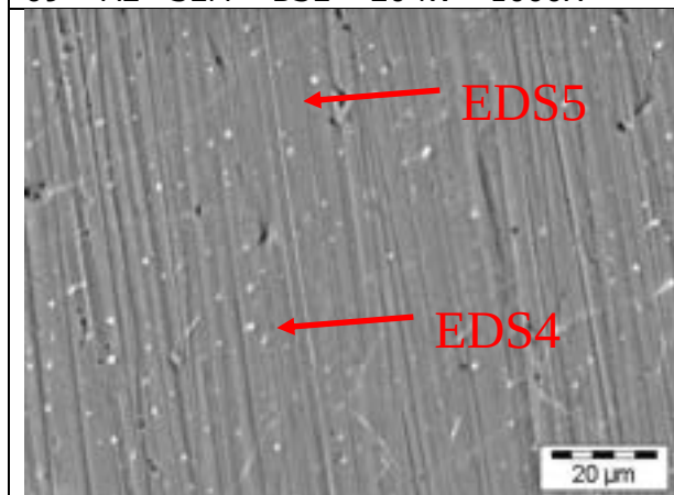
11 - A2- SEM - BSE - 20 kV - 1000X
