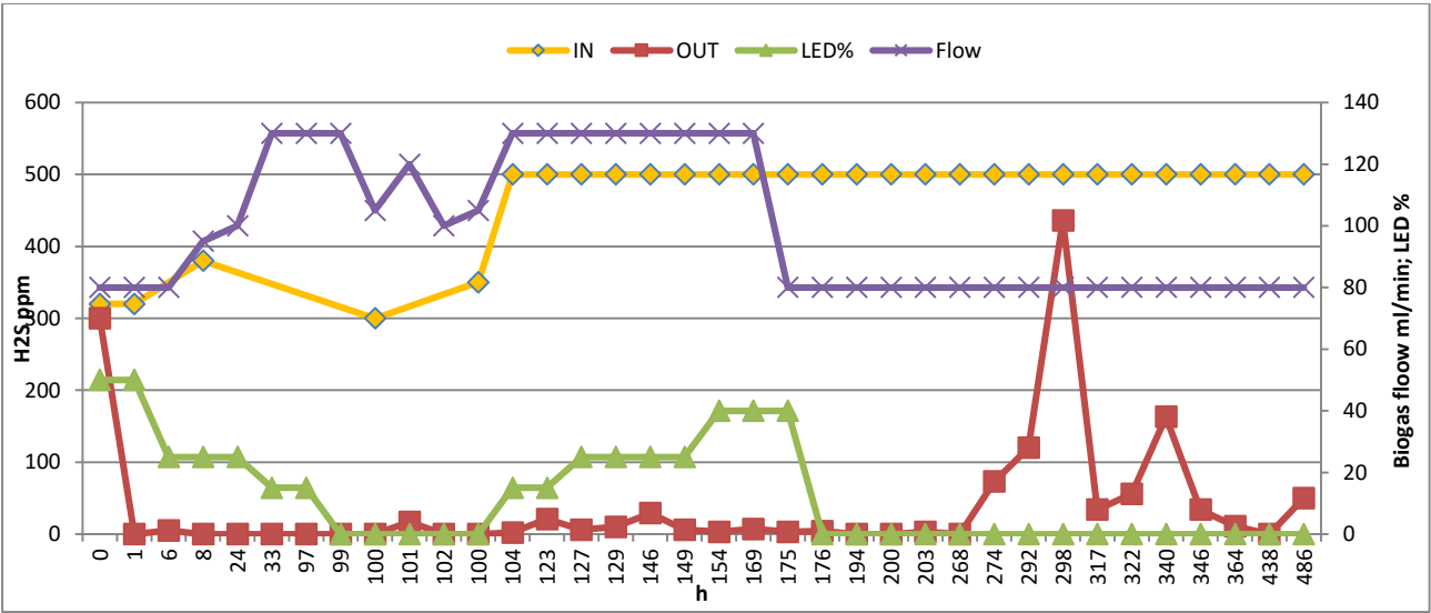
Figura 5. Dati relativi al FBR nel secondo esperimento. Concentrazione dell' H_2S (ppm) del biogas in entrata nel FBR (IN), concentrazione dell' H_2S (ppm) del biogas in uscita nel FBR (OUT), % di utilizzo dei LED e flusso( mlmin^{-1} ) di biogas trattato(Flow)
