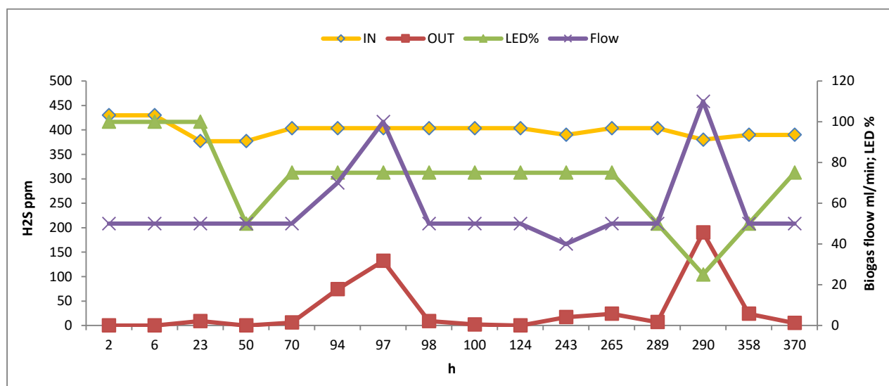
Figura 3. Dati relativi al FBR nel primo esperimento. Concentrazione dell’ H_2S (ppm) del biogas in entrata nel FBR (IN), concentrazione dell’ H_2S (ppm) del biogas in uscita nel FBR (OUT), % di utilizzo dei LED e flusso (mlmin -1 ) di biogas trattato (Flow)
