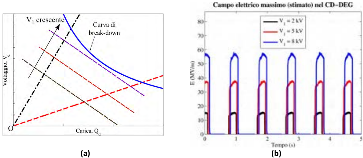
Figura 10. (a) Effetto dell'aumento di V_I sui cicli di controllo del DEG; (b) Stima del campo elettrico al tip del CD-DEG ottenuta dai valori misurati di V_d e dalla stima dello spessore al tip per il caso di onde regolari. I dati sono relativi alla sola fase in cui h > 0 a causa dei limiti dell'apparecchiatura.
