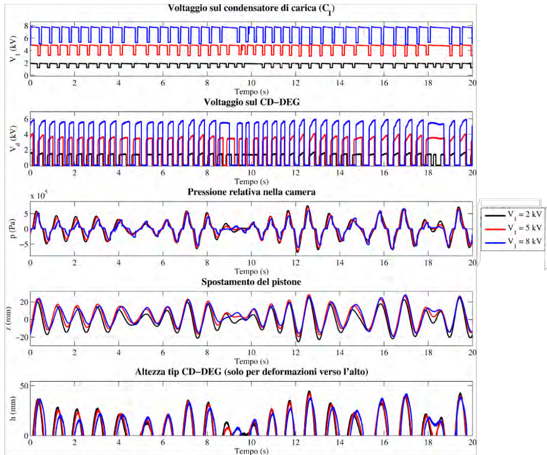
Figura 11. Profili temporali delle principali grandezze misurate ( V_1 , V_d , p , z ed h ) ottenuti con un'onda irregolare ( T_e = 0.91 s e H_s = 4.55 cm) e per tre diversi valori del voltaggio V_1 imposto. I dati relativi all'altezza del tip, h (lettura del sensore CCD), sono relativi alle sole fasi in cui la membrana è espansa verso l'alto.
