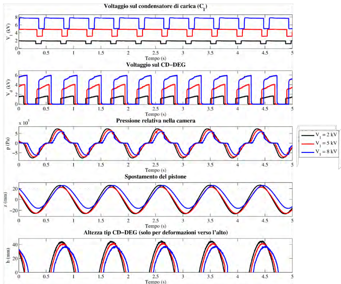
Figura 9. Profili temporali delle principali grandezze misurate ( V_1 , V_d , p , z ed h ) ottenuti con un'onda regolare ( T = 0.91 s e H = 3.2 cm) e per tre diversi valori del voltaggio V_1 imposto. I dati relativi all'altezza del tip, h (lettura del sensore CCD), sono relativi alle sole fasi in cui la membrana è espansa verso l'alto.
