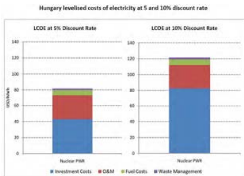
Figura 1: costo del kWh da fonte nucleare per due diversi tassi di sconto in Ungheria [1].
