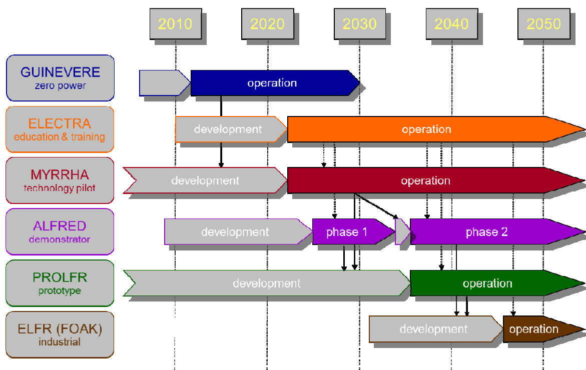
Figura 2: Roadmap sviluppo dei sistemi LFR
