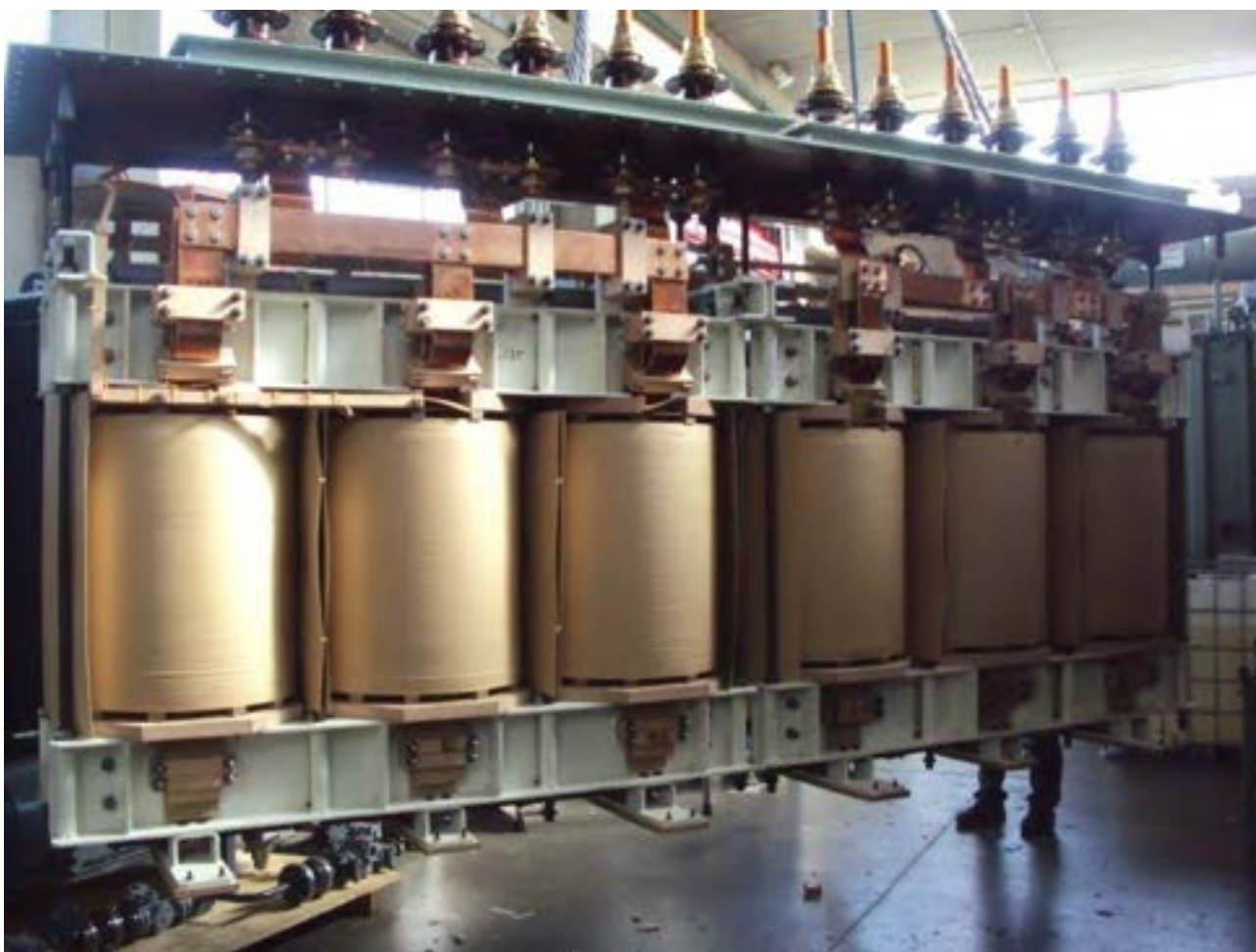
Figura 3 - Costruzione del trasformatore CS3.
