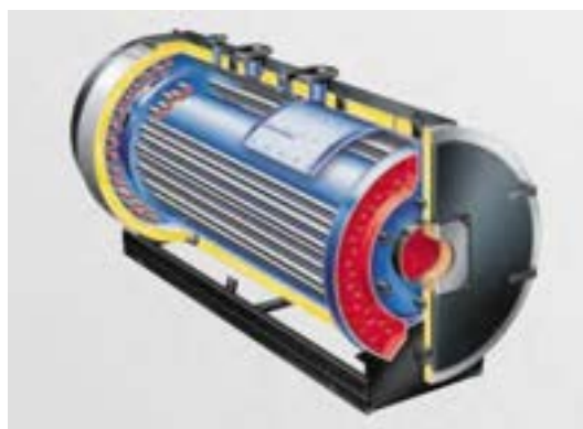
Figura 9 - Sezione di caldaia Vitomax 200
