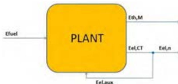
Figura 20 - Flussi energetici entranti/uscenti dall'impianto
