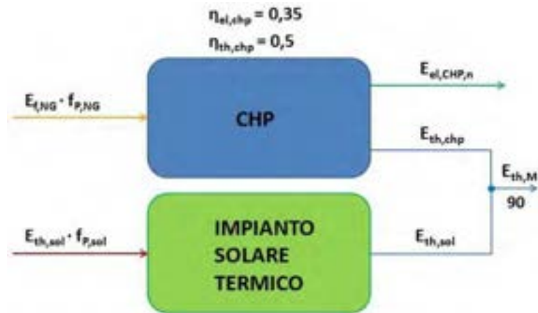
Figura 29 - Generazione tramite CHP e solare termico
