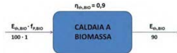
Figura 27 - Generazione tramite caldaia a biomassa
