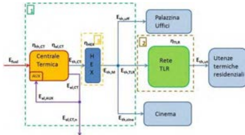
Figura 33 - Schema semplificato di impianto
