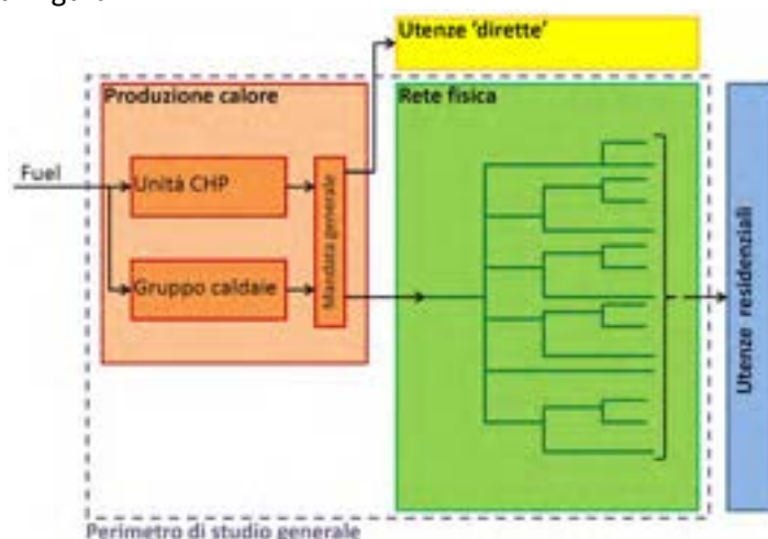
Figura 4 – schema a blocchi dell'intero impianto con annessa rete di teleriscaldamento
