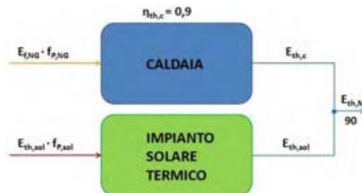
Figura 28 - Generazione tramite caldaia e solare termico
