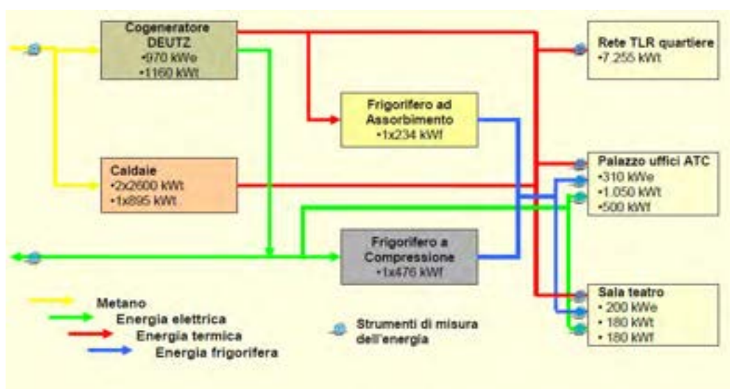
Figura 5 - Schema della Centrale Termica
