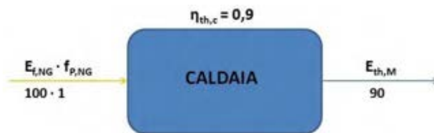
Figura 21 - Generazione con caldaia a gas naturale
