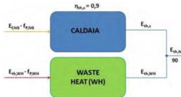
Figura 24 - generazione tramite caldaia a gas e sfruttamento calore di scarto
