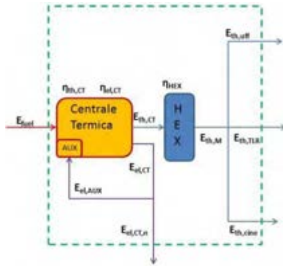
Figura 35 - Volume di controllo 1
