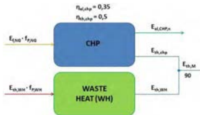
Figura 25 - generazione tramite cogenerazione e sfruttamento calore di scarto
