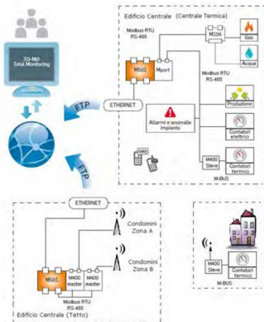
Figura 40 - Architettura sistema di monitoraggio
