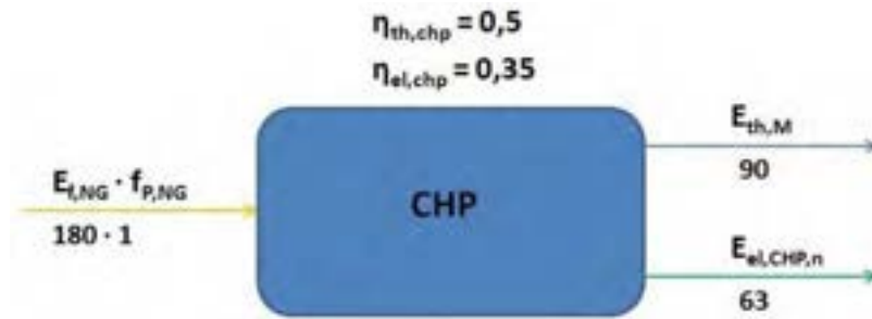
Figura 22 - Generazione tramite CHP
