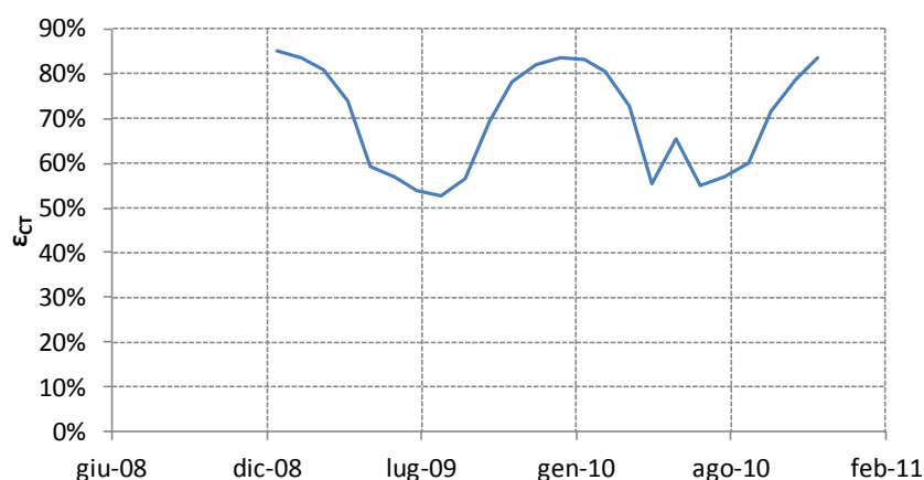
Figura 36 - Efficienza primaria centrale termica
