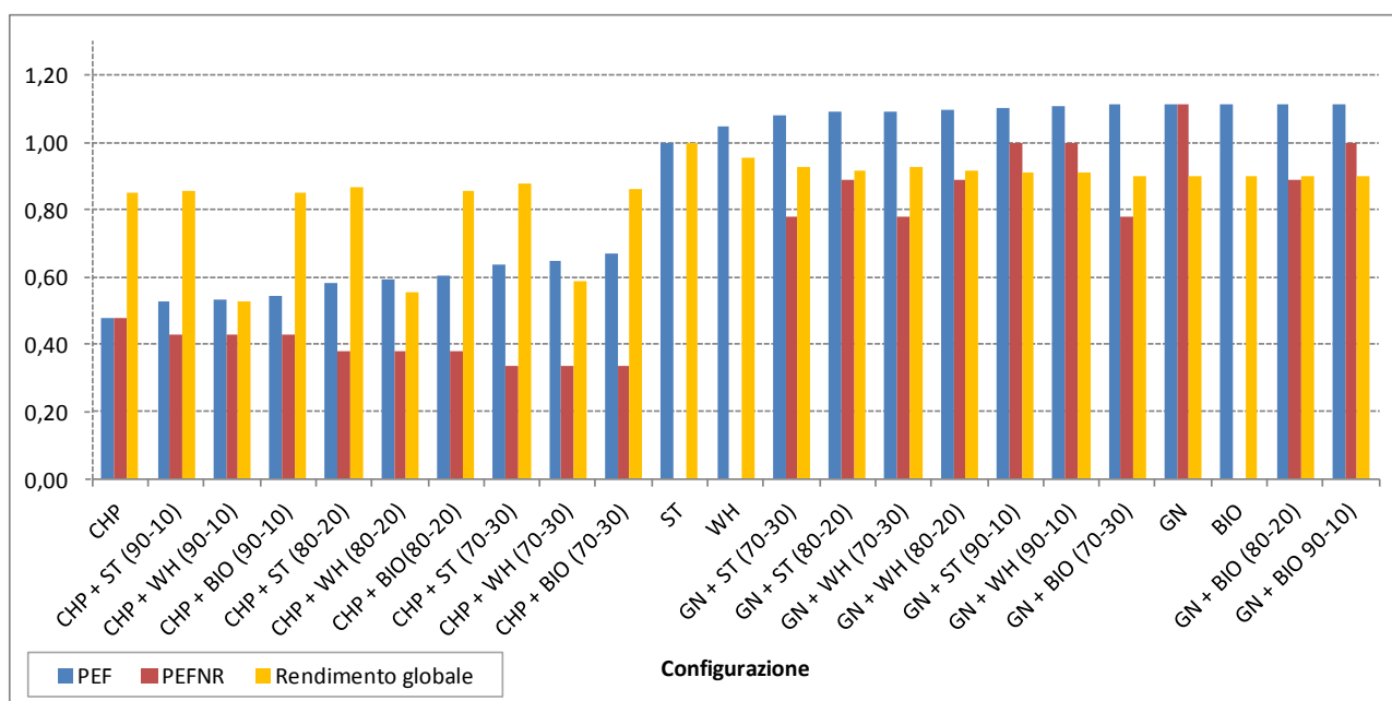
Figura 32 - Ranking in base al PEF delle configurazioni analizzate
