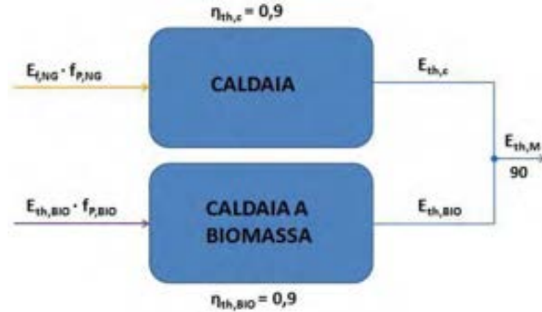
Figura 30 - Generazione tramite caldaia a gas e a biomassa
