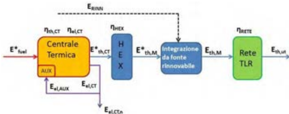
Figura 38 - Schema semplificato impianto di TLR, con adduzione da fonte rinnovabile
