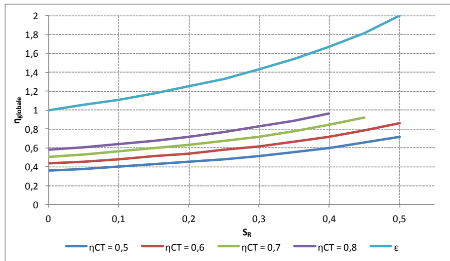
Figura 39 - Rendimento globale impianto
