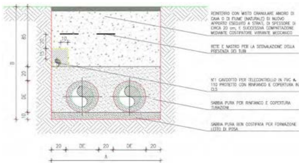
Figura 2 - Sezione di posa tipica
