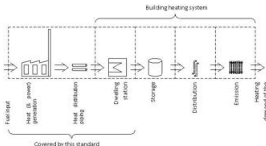
Figura 19 - Schema concettuale suddivisione impianto teleriscaldamento (fonte UNI EN 15316-4-5:2007)
