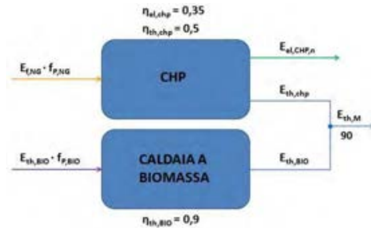
Figura 31 - Generazione tramite CHP e caldaia a biomassa
