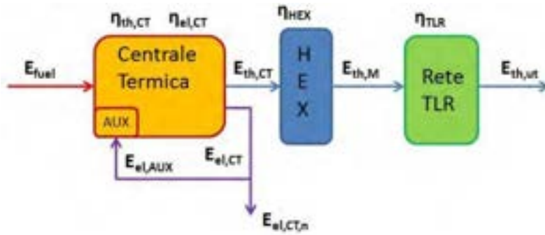
Figura 37 - Schema semplificato impianto teleriscaldamento ad alimentazione esclusivamente fossile
