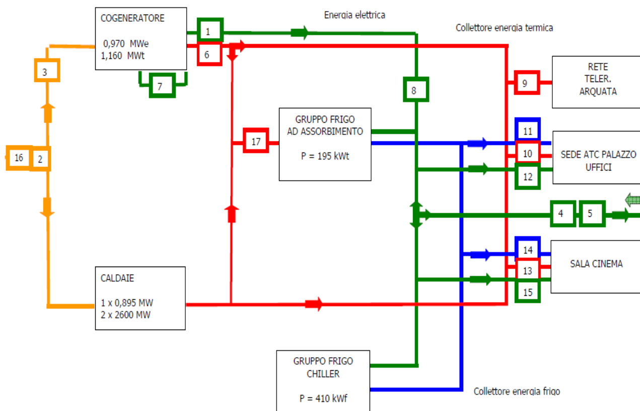
Figura 10 - Schema sensori dell'impianto
