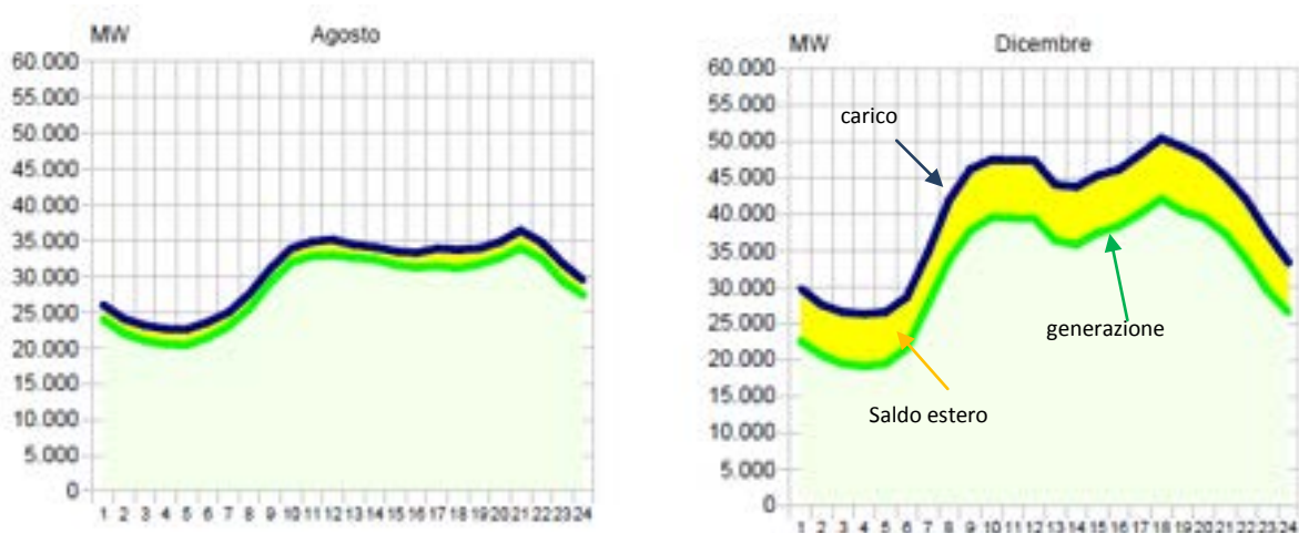
Figura 7 – Carico rete elettrica nazionale 2014- dati Terna [ 13]
