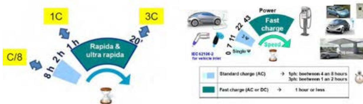
Figura 28 – Variazione della ricarica tra standard e veloce al variare della corrente di ricarica, riferita alla capacità C della batteria
