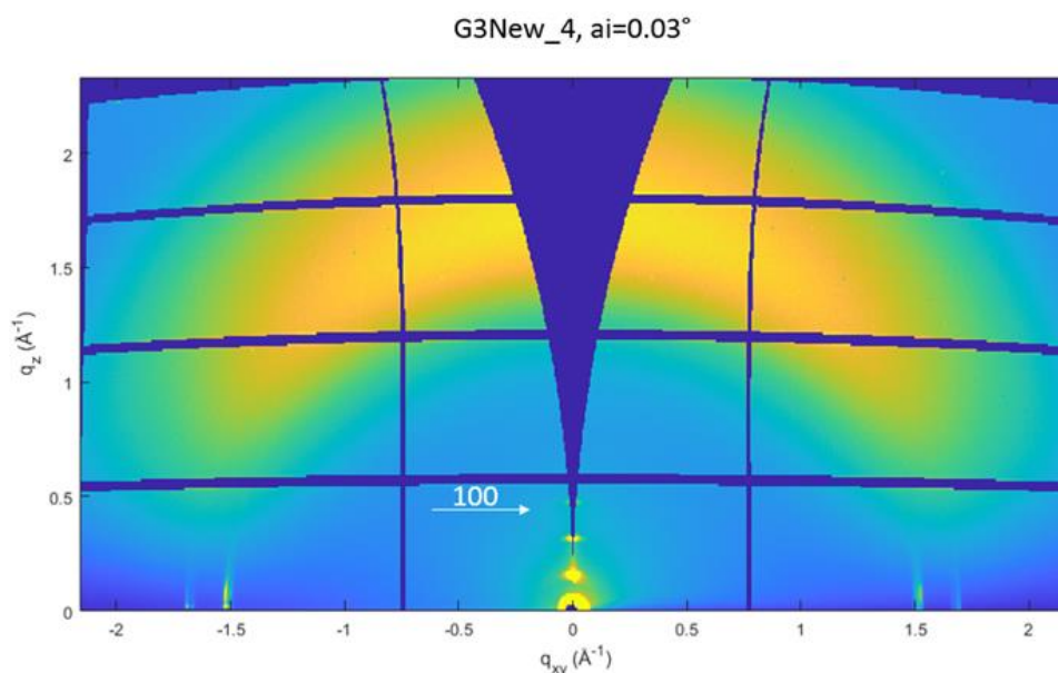
Figura 2: Diffrattogramma GIWAX del campione di PEDOT:ToS:Pridina con un angolo di incidenza di 0.03 °
