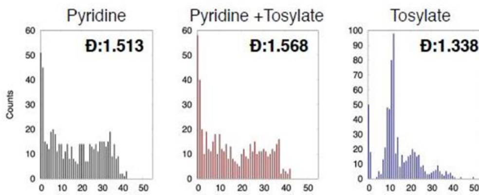
Figura 3: Distribuzione delle lunghezze di catena generata dalla reazione di polimerizzazione in presenza di basi diverse come determinata con tecniche di dinamica molecolare (MD).
