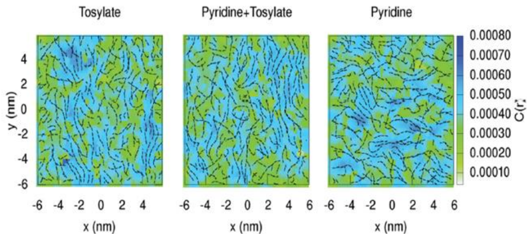
Figura 4: Mappe di correlazione strutturale (cristallinità). Le catene di PEDOT sono rappresentate da linee nere
