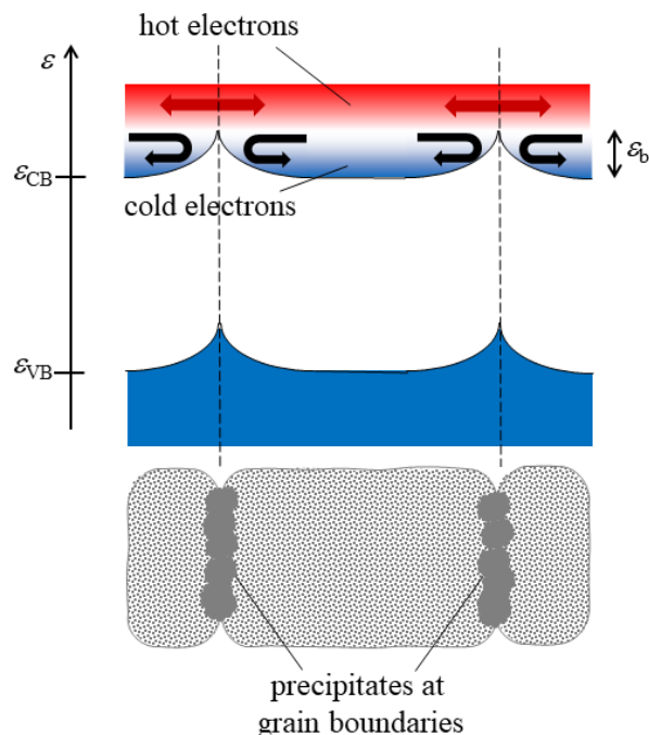
Figura 7: Meccanismo di energy filtering di elettroni [7]. Le barriere di potenziale generate dai precipitati ai bordi di grano selezionano i portatori di carica, localizzando i portatori freddi e consentendo solo a quelli con energia cinetica superiore a \epsilon_b di diffondere nel materiale. La riduzione della densità dei portatori comporta un incremento di \alpha mentre la riduzione della densità è compensata all'aumento della mobilità, sostanzialmente conservando i valori di conducibilità elettrica.
