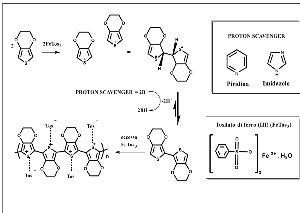
Figura 1: Meccanismo di polimerizzazione ossidativo del PEDOT. Gli scavenger sono responsabili della eliminazione dei protoni.
