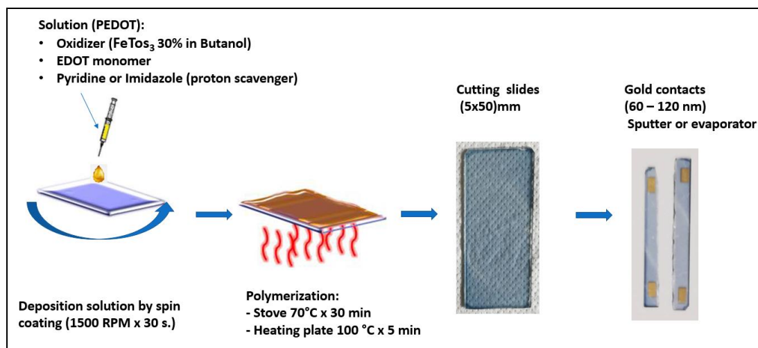
Figura 5: Schema della procedura di reazione.
