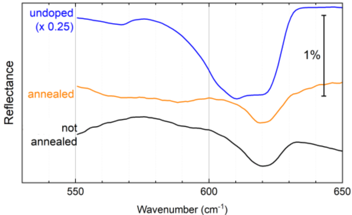
Figura 6: Spettri IR in riflettanza di campioni di silicio nanocristallino non impiantati e impiantati, prima e dopo il trattamento termico.
