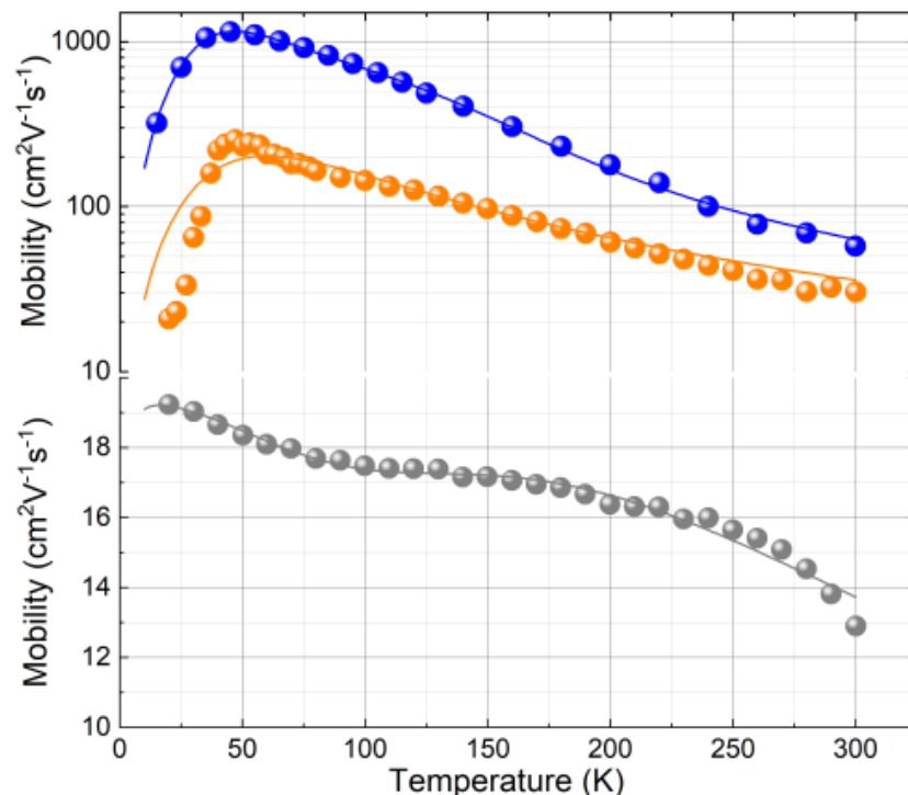
Figura 8: Mobilità Hall delle lacune in funzione della temperatura nei film di silicio nanocristallino non trattati termicamente (grigio) e dopo il trattamento termico a 1000 °C, 2 ore prima (arancione) e dopo (blu) invecchiamento.
