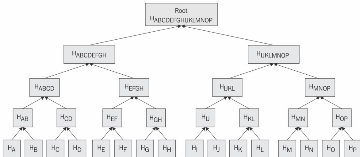
Figure 3: La struttura di un Merkle Tree.
