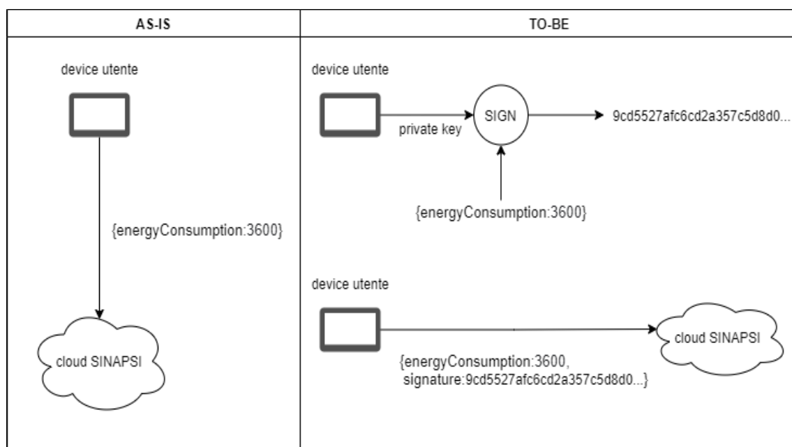
Figure 4: Segmento device utente-cloud SINAPSI nelle configurazioni AS-IS e TO-BE.
