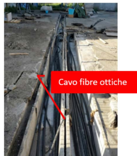
Fasi di realizzazione e strumentazione del campo geotermico presso il C.R. ENEA Casaccia
