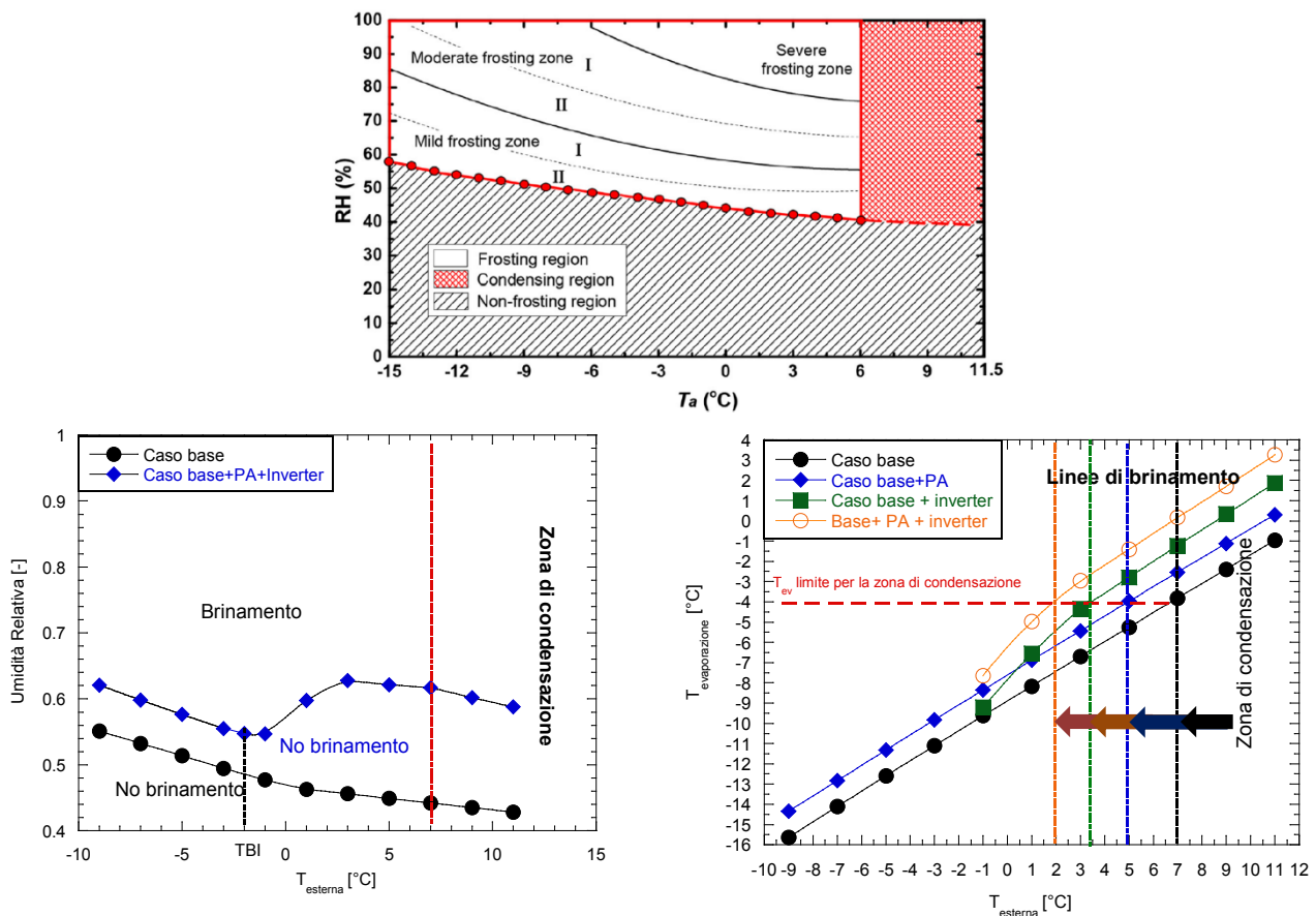
Studi teorici sulla riduzione dell'area di brinamento al variare della temperatura dell'aria e dell'umidità
