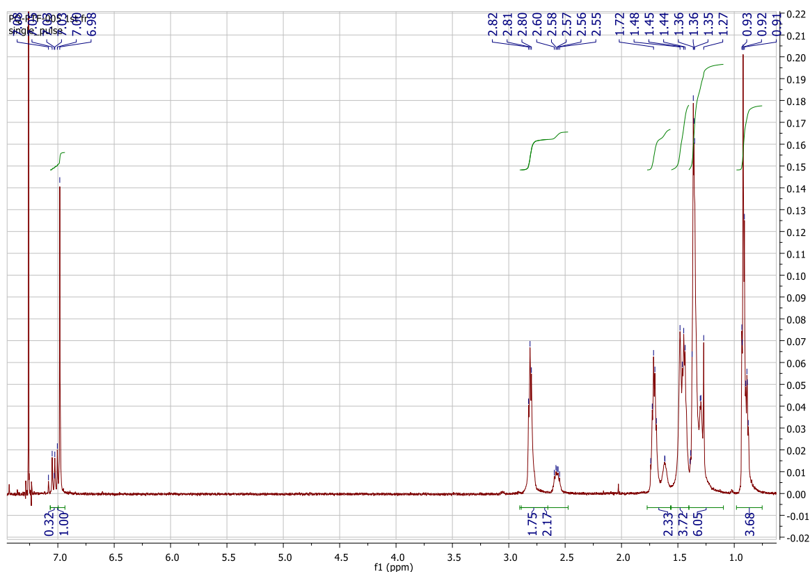
Figura 10. ^1\text{H-NMR} del composto P3HT-005.
