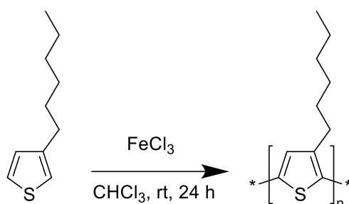
Figura 3. Metodo ossidativo di sintesi di poli(3-esiltiofeni), mediante l'uso di \text{FeCl}_3 .
