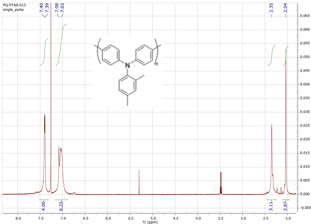
Figura 17. ^1\text{H-NMR} del composto PTAA-013.
