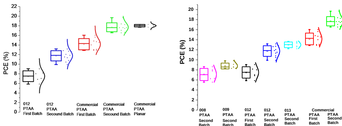
Figura 9. Grafici di efficienza fotovoltaica ottenuti con due differenti procedure sulle 4 PTAA sintetizzate, a confronto con una PTAA commerciale.
