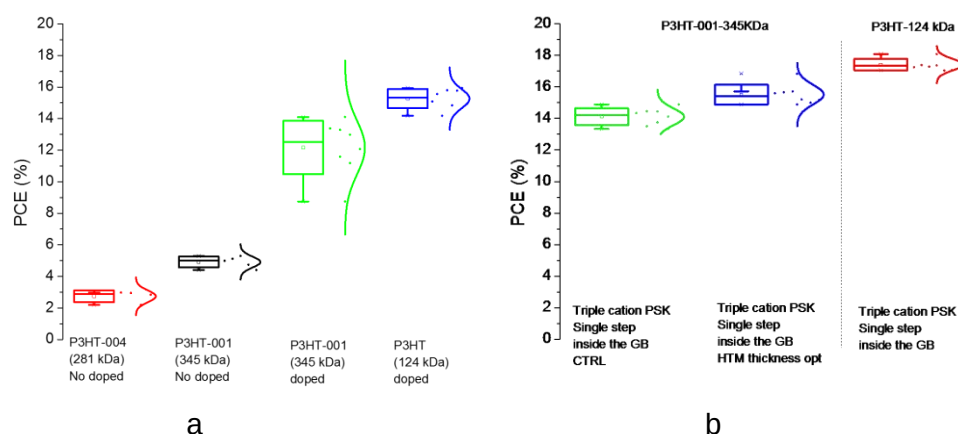
Figura 7. Grafici di efficienza fotovoltaica ottenuti con due differenti perovskiti con alcuni dei polimeri preparati dal gruppo di ricerca MOF dell'Università di Torino. Sono riportati i limiti di variazione delle misure e i singoli punti, corredati della distribuzione della media dei dati: a) confronto tra P3HT-001, P3HT-004 in stato dopato e non dopato e standard P3HT-124kDa (dopato); b) confronto tra deposizione ordinaria (CTRL) e di spessore ottimizzato per P3HT-001, e lo standard P3HT-124kDa, in stato dopato.
