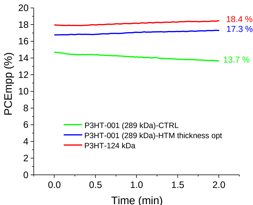
Figura 8. Caratterizzazione di celle PSC tramite MPP (Maximum Power Point tracking) basate su P3HT-001-289 kDa (dopato) e P3HT-124 kDa (dopato), come materiale HTM.
