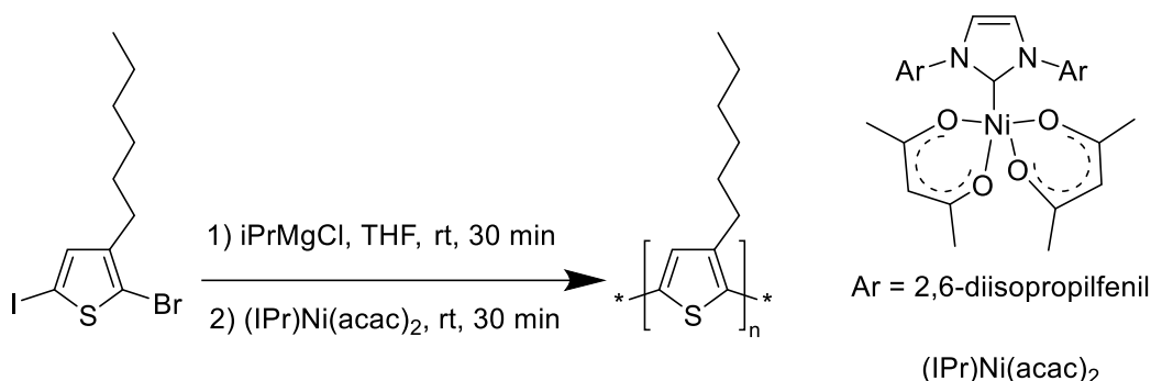
Figura 4. Metodo GRIM di sintesi di poli(3-esilpolitiofeni).
