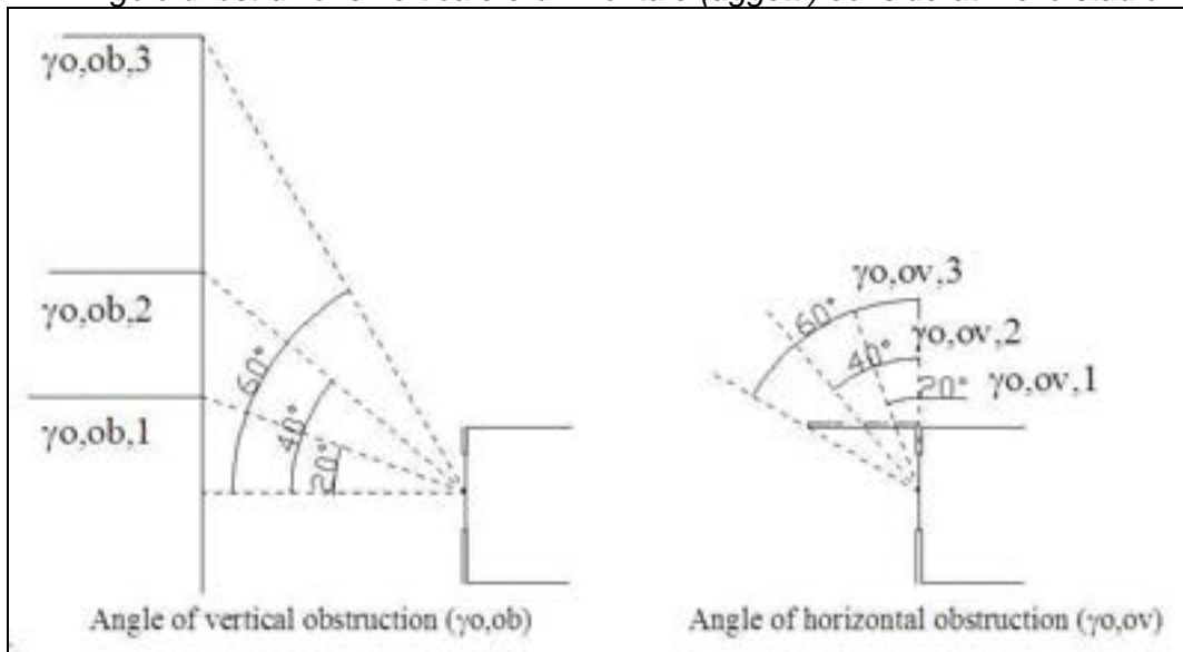
Figure 2.7 – Angolo di ostruzione verticale e orizzontale (aggetti) considerati nello studio
