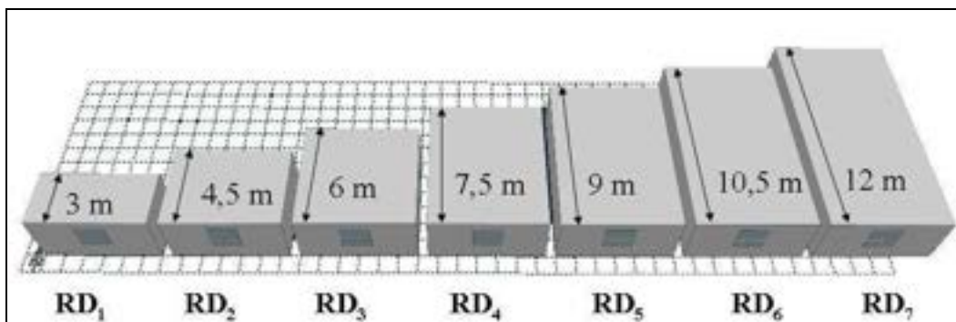
Figure 2.6 – Profondità della zona di riferimento assunte nel calcolo
