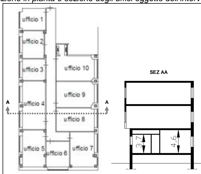
Figura 3.7 – Individuazione in pianta e sezione degli uffici oggetto dell'intervento pilota
