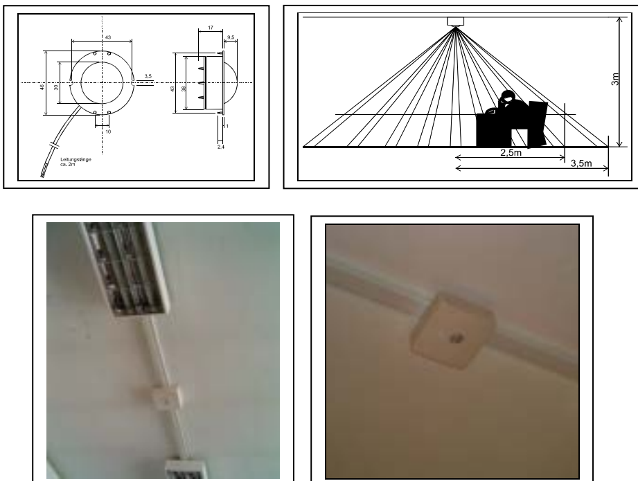
Figura 3.4 – Sensore misto: dimensioni, campo di lettura e collocazione in ambiente
