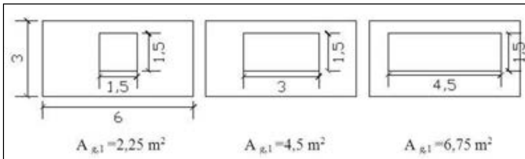
Figure 2.5. Dimensioni delle superfici vetrate assunte nel calcolo
