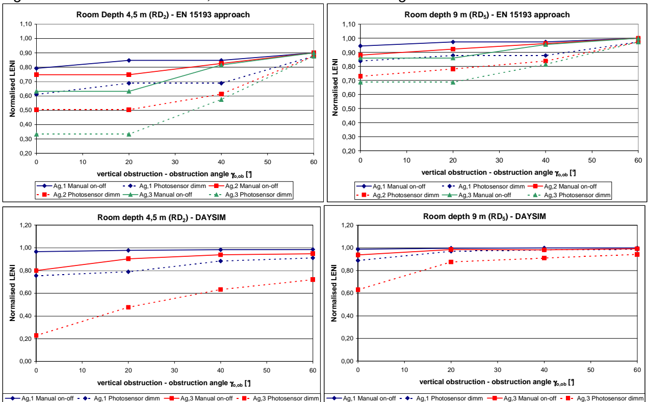
Figura 2.9 – LENI normalizzato, calcolato in funzione dell'angolo di ostruzione verticale
