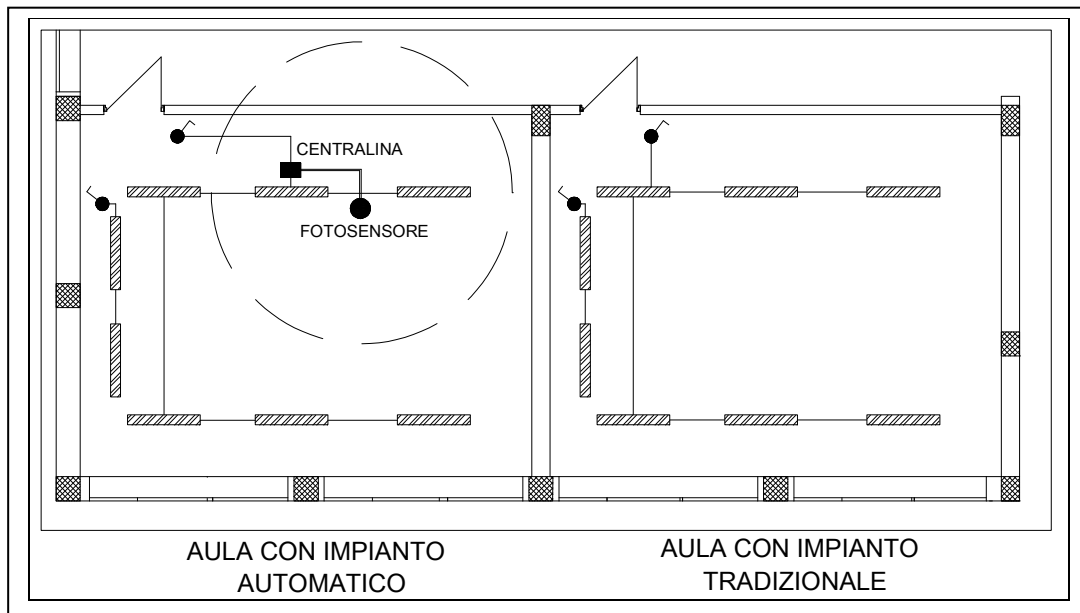
Figura 3.3 - Cablaggio elettrico e di segnale delle due aule
