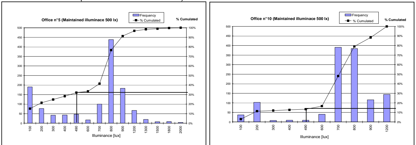
Figure 3.17: Controllo automatico & manuale. Distribuzione di frequenza e frequenza cumulata dell'illuminamento (dal 16/01/08 al 14/03/08)
