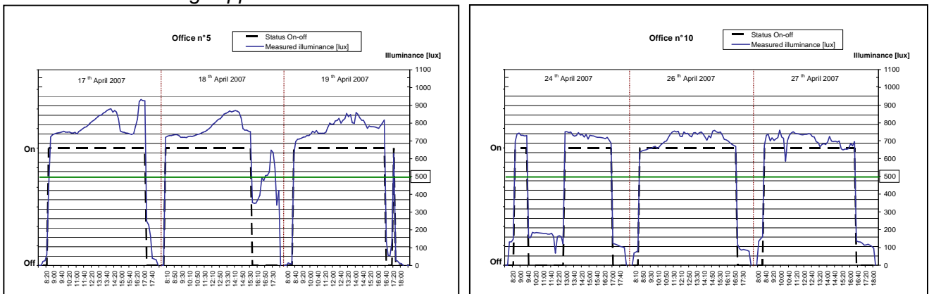
Figura 3.18: Controllo manuale. Illuminamento interno misurati sulla scrivania rapportato allo stato di funzionamento degli apparecchi
