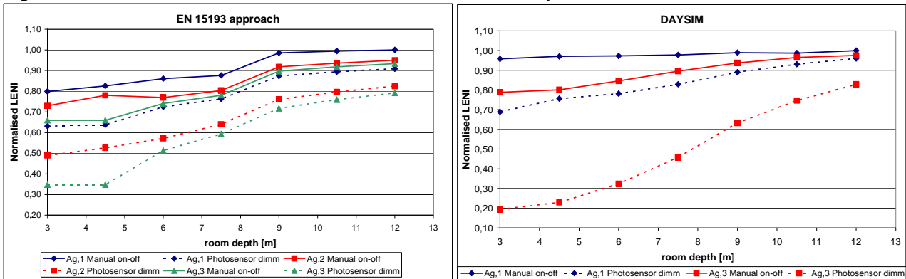
Figura 2.8 – LENI normalizzato, calcolato in funzione della profondità della zona
