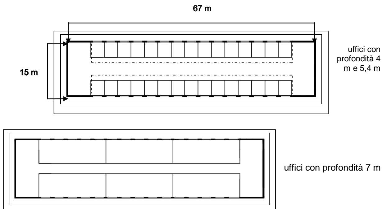
Figura 2.2 – Rappresentazione delle tre configurazioni di finestra ipotizzate per l'edificio tipo
