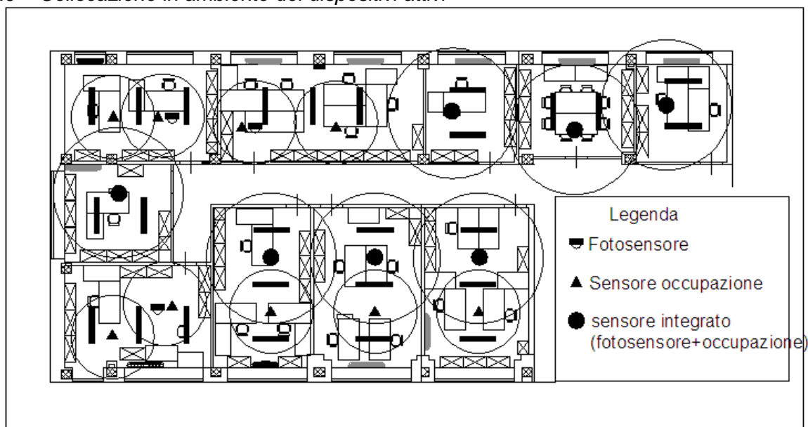
Figura 3.9 – Collocazione in ambiente dei dispositivi attivi
