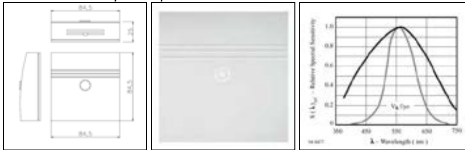
Figura 3.10 – Dimensioni e risposta spettrale del fotosensore LRA1
