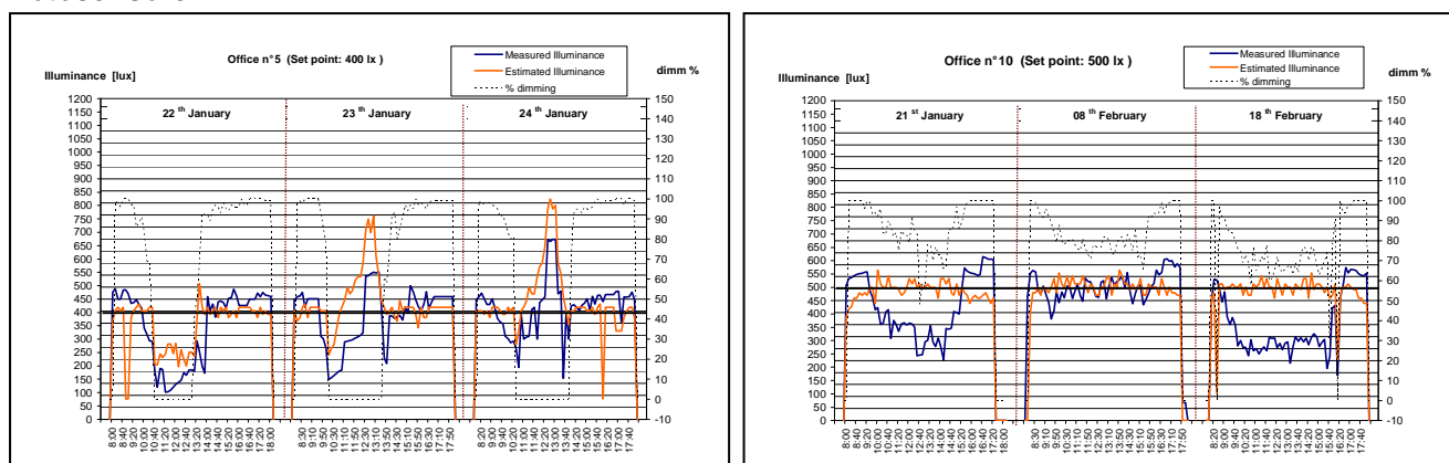
Figura 3.19: Controllo automatico & manuale. Illuminamento interno misurati sulla scrivania rapportato allo stato degli apparecchi (% di regolazione) e all'illuminamento secondo la lettura del fotosensore
