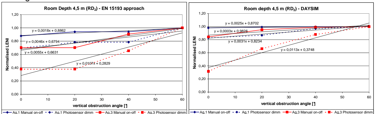
Figure 2.12. Linee di tendenza e corrispondenti equazioni ottenute dai dati relativi alla variazione dell'angolo di ostruzione esterna verticale
