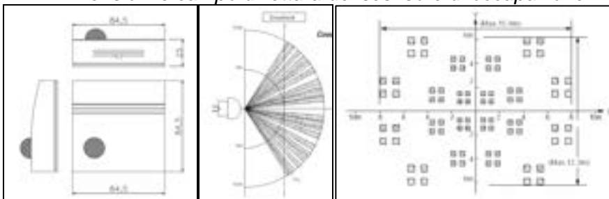
Figura 3.11 – Dimensioni e campo di lettura del sensore di occupazione WRF 041
