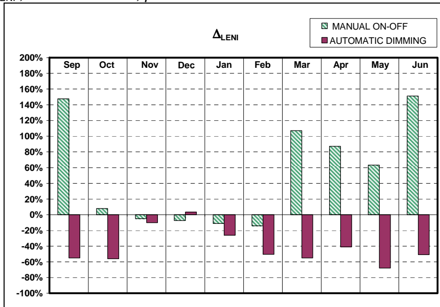
Figura 2.5 - \Delta_{LENI} , su base mensile, per le due aule caratterizzate dal diverso sistema di controllo
