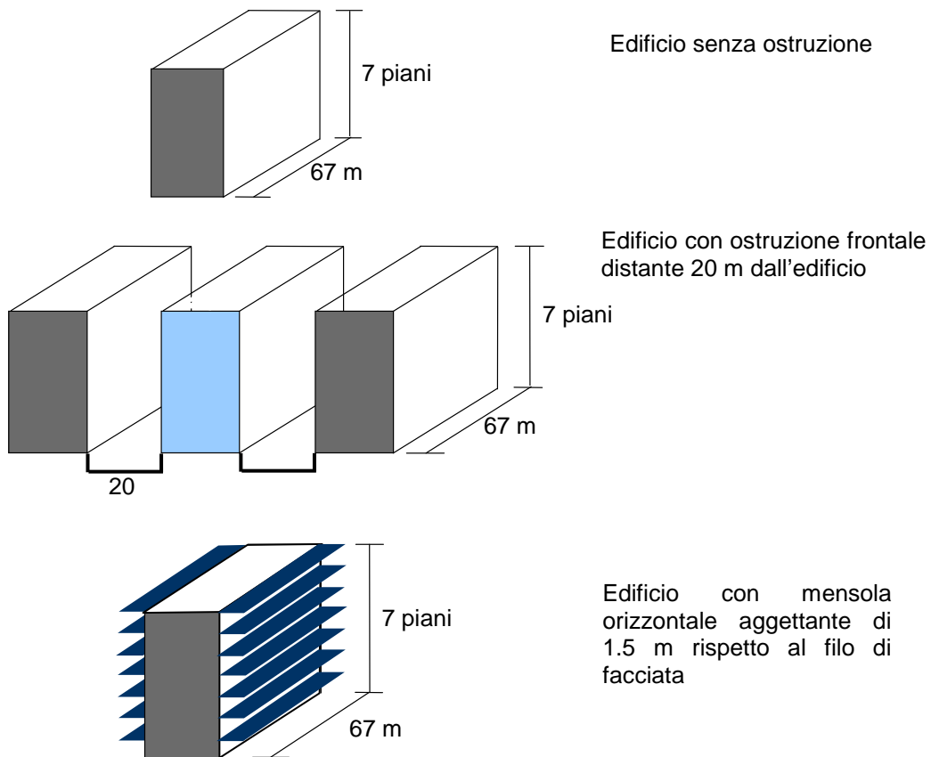
Figura 2.3 – Rappresentazione schematica delle ostruzioni esterne considerate per l'edificio tipo
