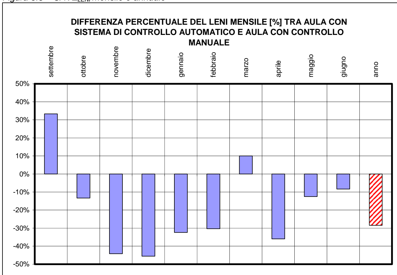
Figura 3.5 – SAVE_{LENI} mensile e annuale
