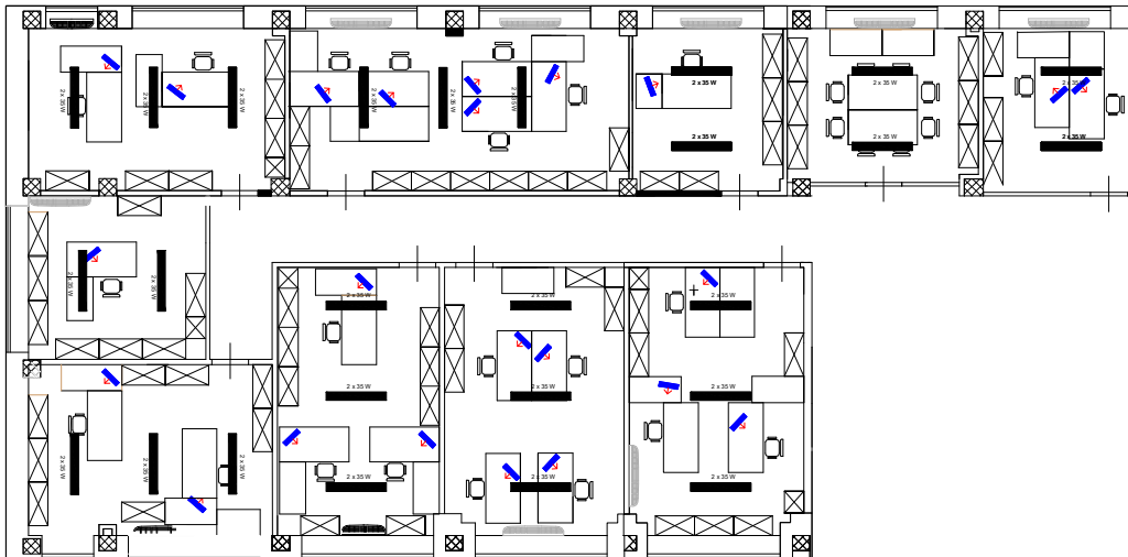
Figura 3.8 – Allestimento degli uffici e layout degli apparecchi di illuminazione
