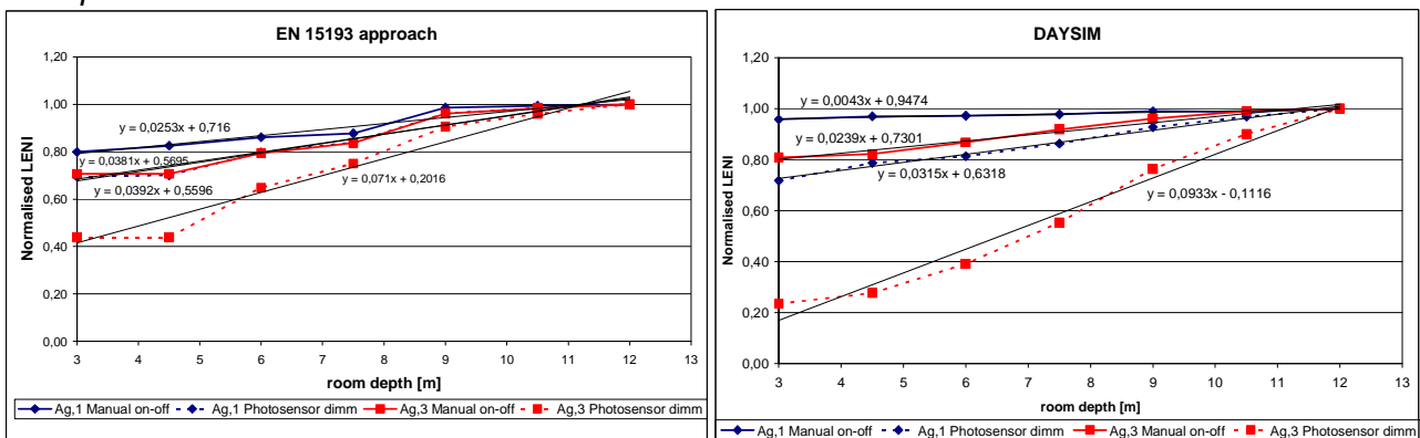
Figure 2.11. Linee di tendenza e corrispondenti equazioni ottenute dai dati relativi alla variazione della profondità della zona
