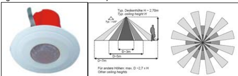
Figura 3.12 – Dimensioni e campo di lettura del sensore di misto MDS
