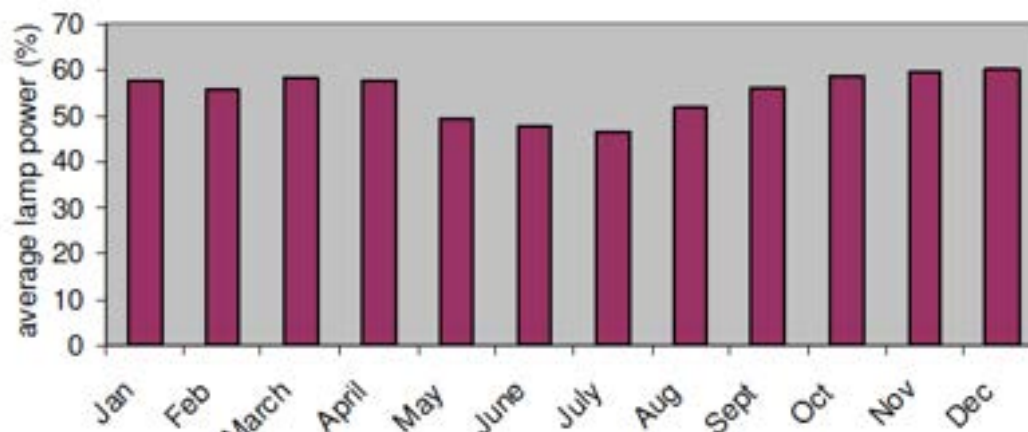
Figura 66 Percentuale della potenza media mensile rispetto a quella nominale per l'impianto Ring III. Nel corso dell'intero anno, le lampade hanno funzionato mediamente al 55% della loro potenza nominale.
