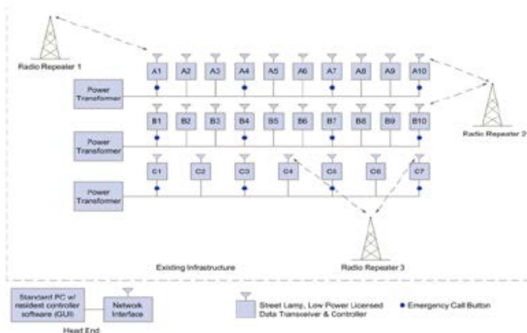
Figura 84 Architettura del sistema di controllo Relume Sentinel
