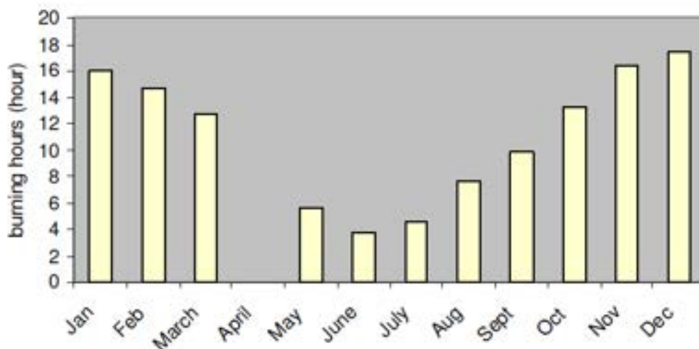
Figura 67 Distribuzione del numero di ore di funzionamento giornaliere medie mensili per l'impianto VT7. In Giugno il numero medio di ore di funzionamento giornaliero è pari a 4h, mentre d Dicembre è pari a circa 17h. Il numero totale di ore di funzionamento si aggira intorno alle 3850 h annue.
