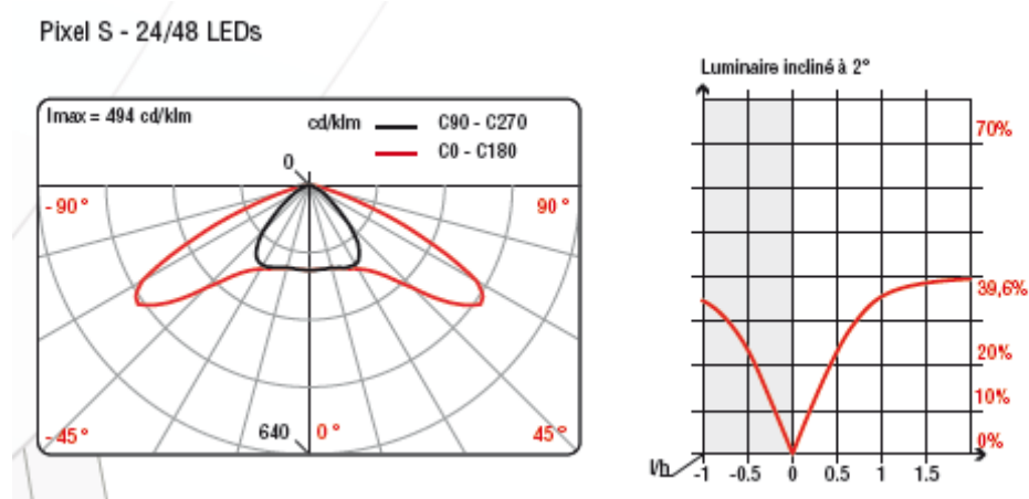
Figura 40 Apparecchio Eclatec Pixel S 24/48 LED. Indicatrici di emissione e fattore di utilizzazione
