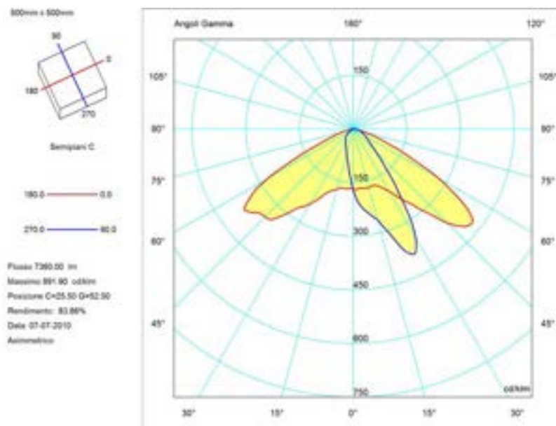
Figura 51 Risultato della simulazione di Ray tracing, che tiene conto sia della coppa di chiusura, sia degli effetti di schermatura. (Cortesia FRAEN)
