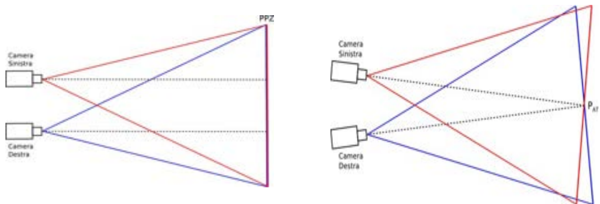
Fig.3 Modalità "asymmetric frustum" (a sinistra) e "toe-in" (a destra)
