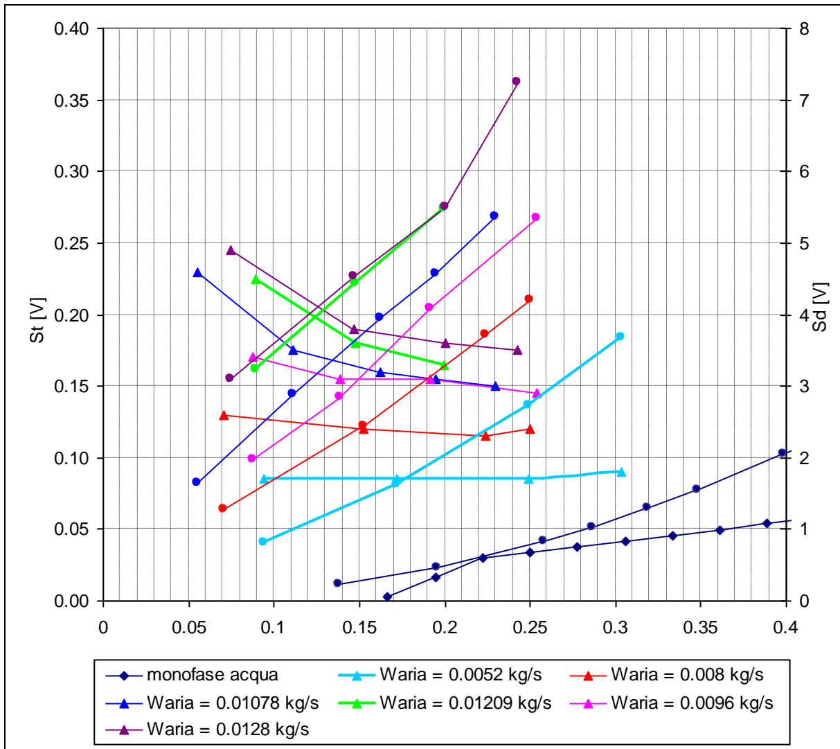
Fig. 38: Mappa SP. Asse x : W_{acqua} [kg/s], Simboli: Segnale Turbina = ▲. Segnale Drag = ●.
