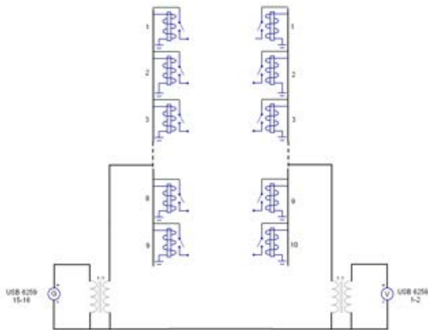
Fig. 3: Schema elettrico Sonda capacitiva
