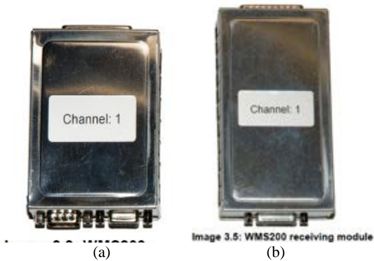
Fig. 2: Modulo Trasmettitore (a) e Modulo ricevitore (b)
