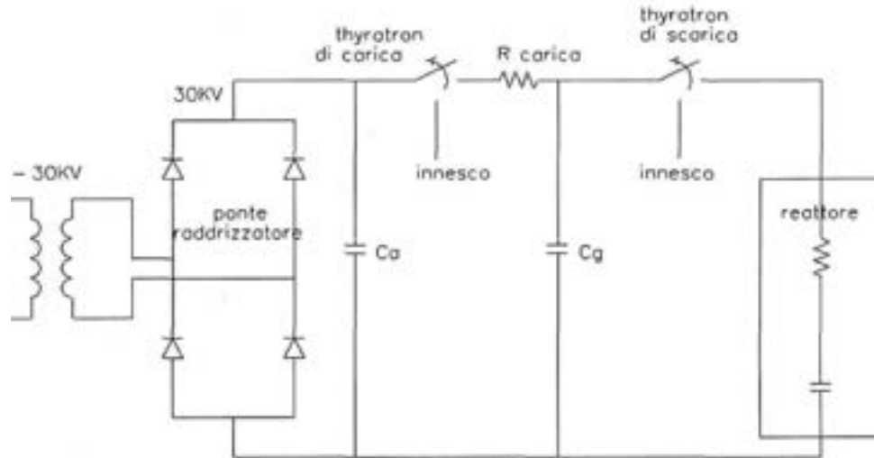
Fig. 8: Schema del circuito di scarica del reattore corona
