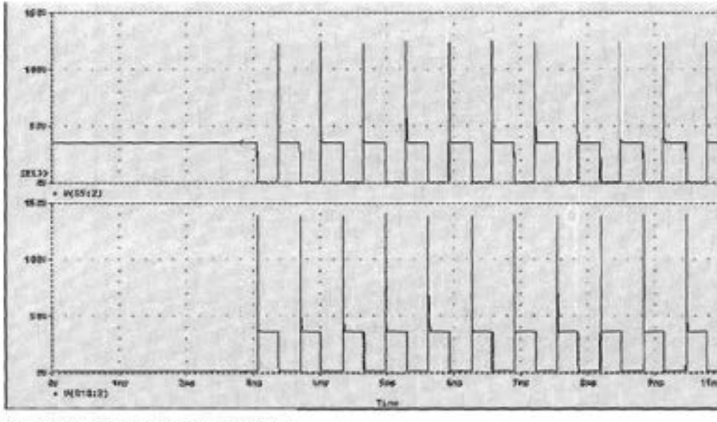
Fig. 10: Impulsi di innesco dei thyatron.
