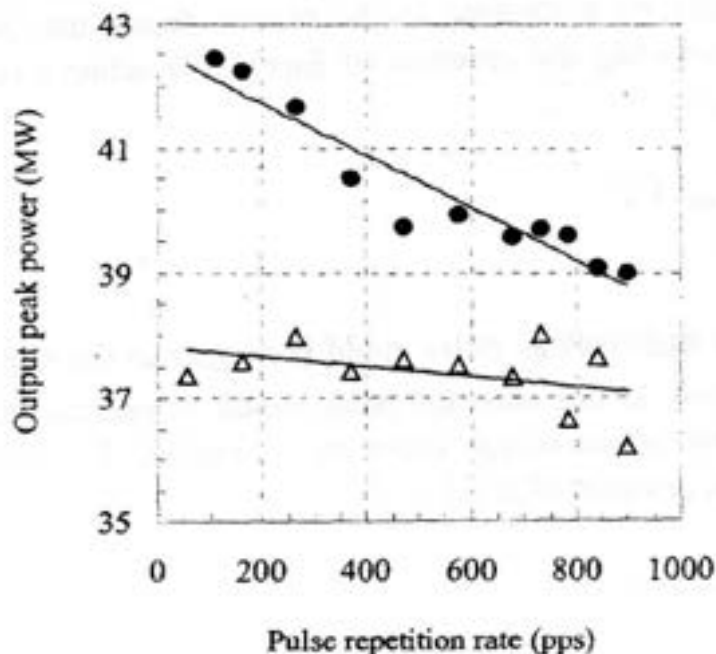
Fig. 6: Effetti del layout costruttivo sulla potenza in uscita con un carico resistivo ●: piccola taglia; Δ: grande taglia
