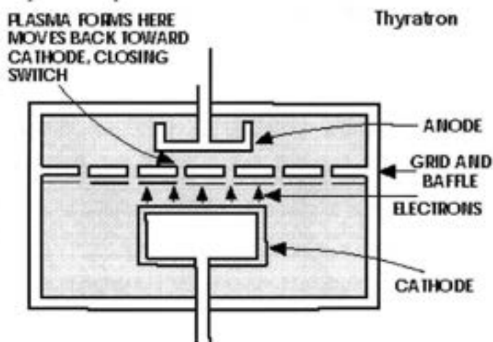
Fig. 7: Rappresentazione schematica di un thyatron.
