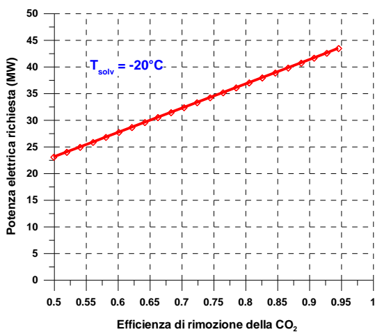
Figura 2.3.35 Potenza elettrica richiesta in funzione della efficienza di rimozione della CO 2 .
