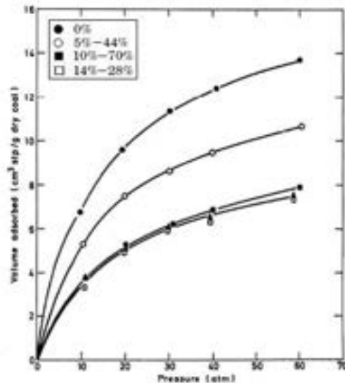
Figura 2.12. : Capacità di assorbimento in funzione dell'umidità (Carbosulcis, 2009).
