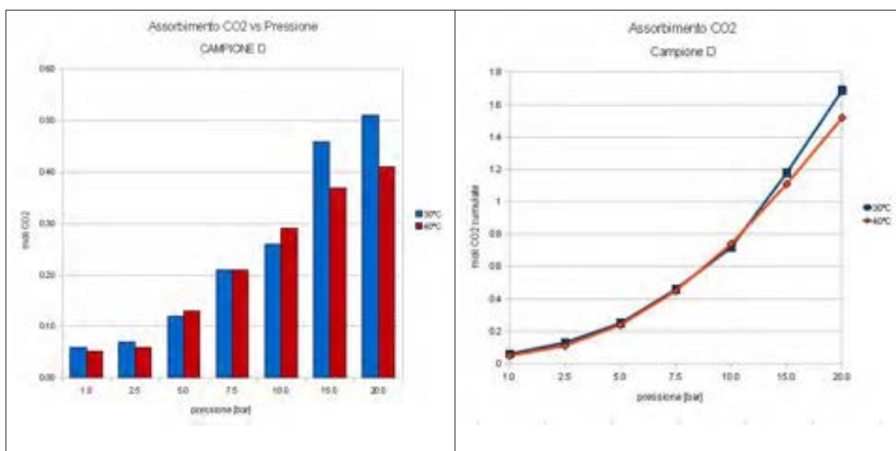
Figura 3.3.: Capacità di assorbimento del Campione D in funzione della temperatura.
