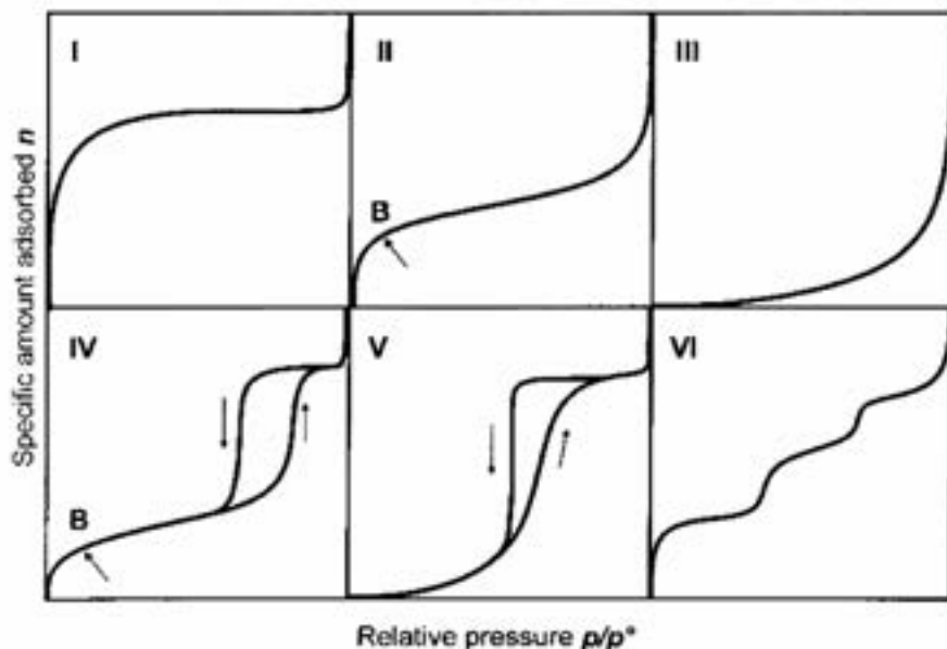
Figura 6.1. : Tipologia di isoterme di assorbimento (Sing K.S.W., e al.).
