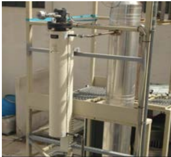
Figura 2.3.2.1: Scambiatore elettrico preriscaldamento ammine
