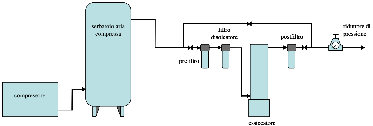
Figura 2.2.1: Sistema di trattamento aria processo
