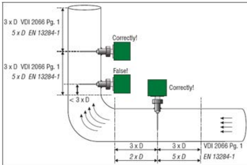
Figura 2.5.3.4: Schema di montaggio della sonda in accordo con diverse normative di riferimento
