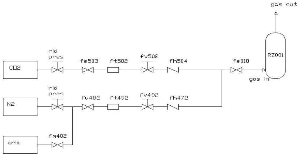
Figura 2.3.1.1: Schema del circuito di circolazione gas
