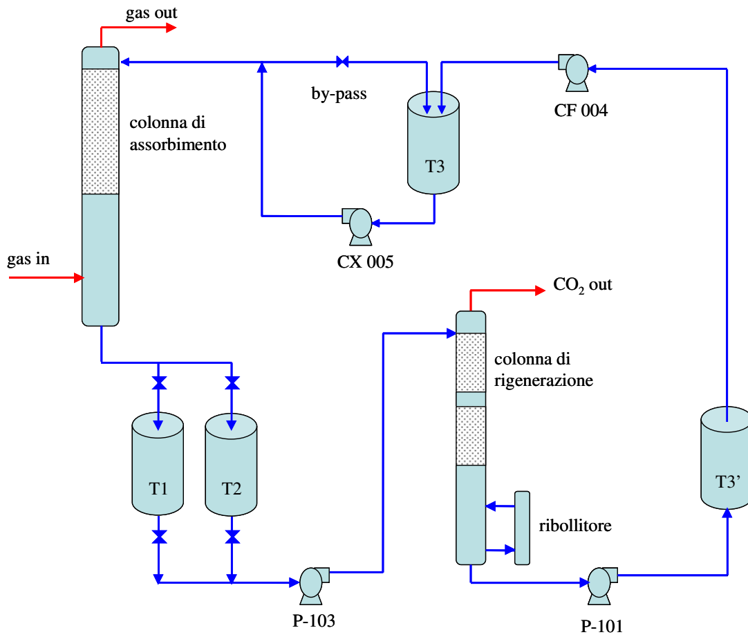
Figura 2.3.1.2: Schema del circuito di circolazione ammine
