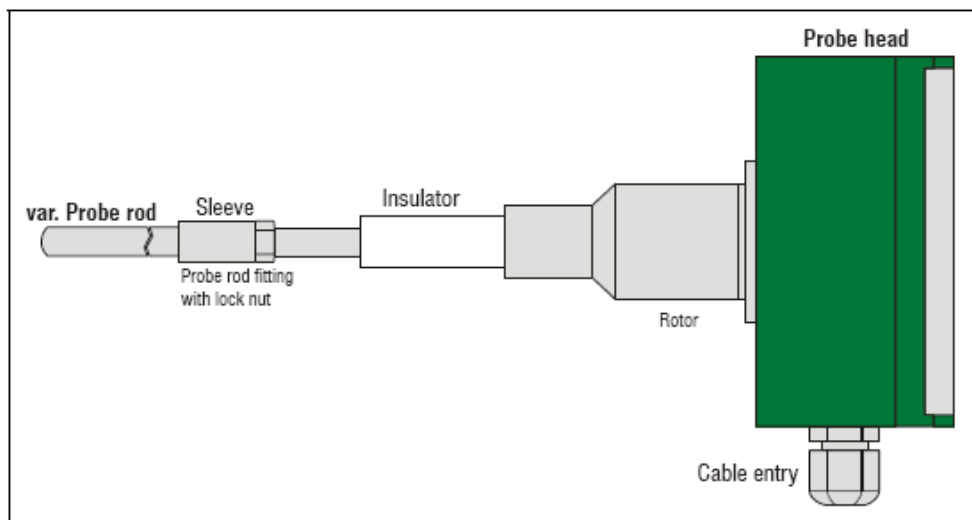
Figura 2.5.3.2: Sonda del sistema di rilevazione polveri
