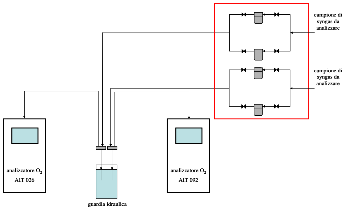
Figura 2.5.2.1: Sistema di campionamento degli analizzatori O 2
