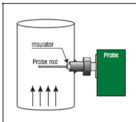
Figura 2.5.3.3: Schema di montaggio della sonda di rilevazione polveri
