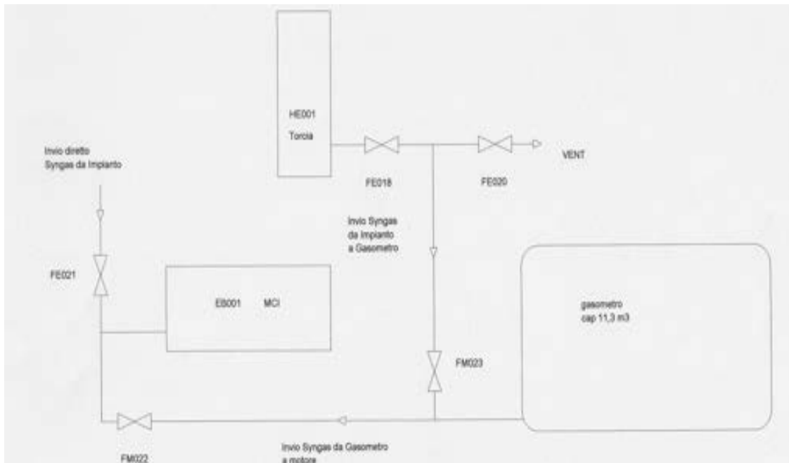
Figura 2.4.1.3: Schema di inserimento del gasometro nell'impianto pilota
