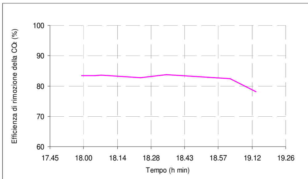
Figura 7.6. Andamento dell'efficienza di rimozione della CO 2 .
