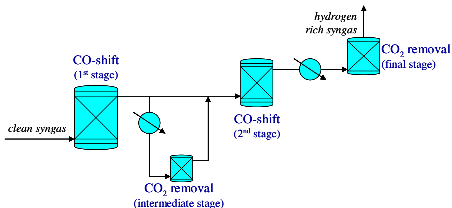
Figura 2.2. Schema di flusso del sistema integrato di CO-shift e assorbimento della \text{CO}_2 .
