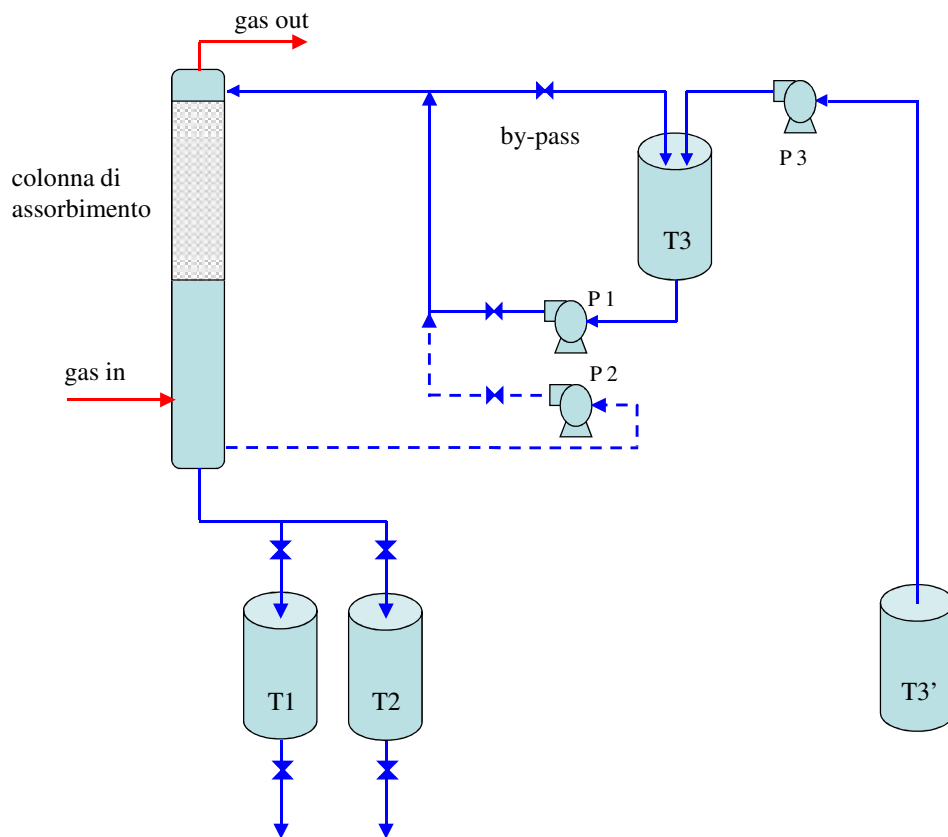
Figura 2.8. Schema di funzionamento a ciclo aperto del II stadio di desolforazione.
