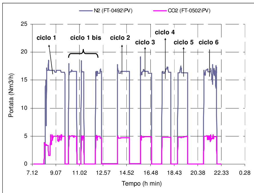
Figura 7.7. Andamento delle portate di N_2 e CO_2 inviate nella colonna di assorbimento.
