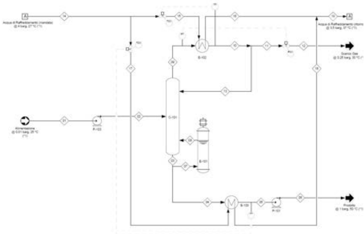
Figura 2.4. Schema semplificato del sistema di rigenerazione delle ammine.
