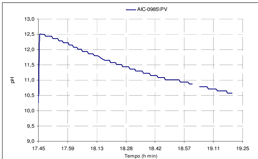
Figura 7.4. Andamento del pH all'interno del II stadio di desolfurazione a freddo.
