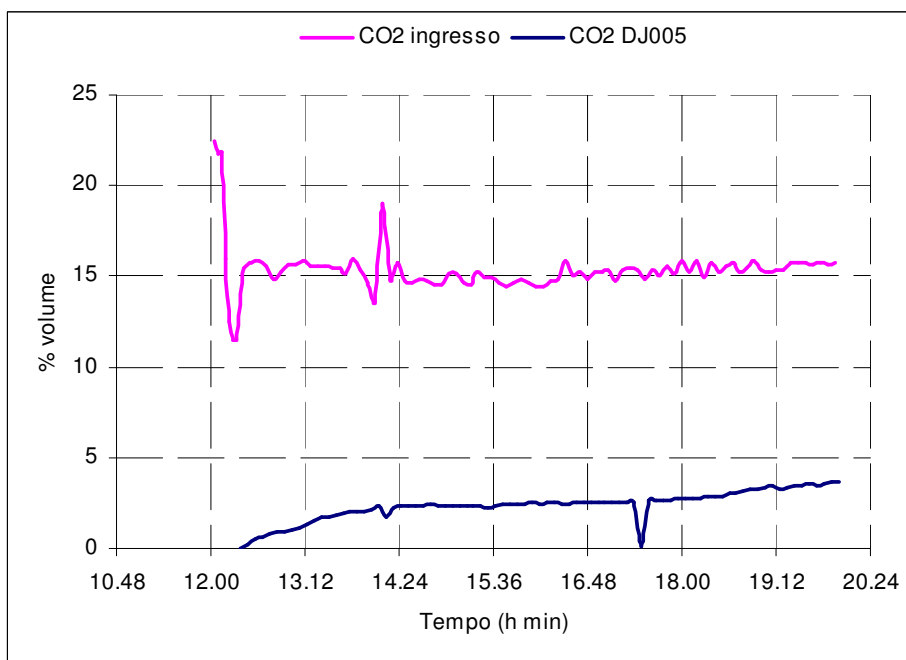
Figura 7.2. Andamento della concentrazione di CO 2 rilevata dalle prese di campionamento in ingresso e in uscita dall'assorbitore.
