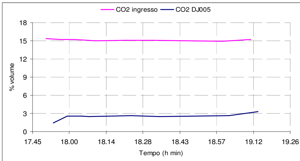
Figura 7.5. Andamento della concentrazione di CO 2 rilevata dalle prese di campionamento In ingresso e in uscita dall'assorbitore.
