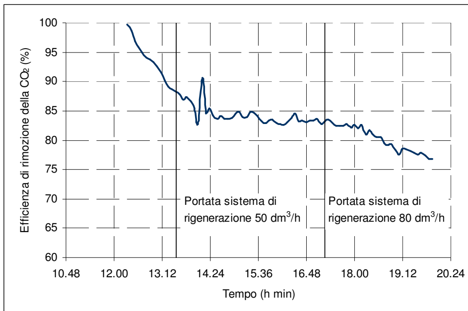
Figura 7.3. Andamento dell'efficienza di rimozione della \text{CO}_2 .
