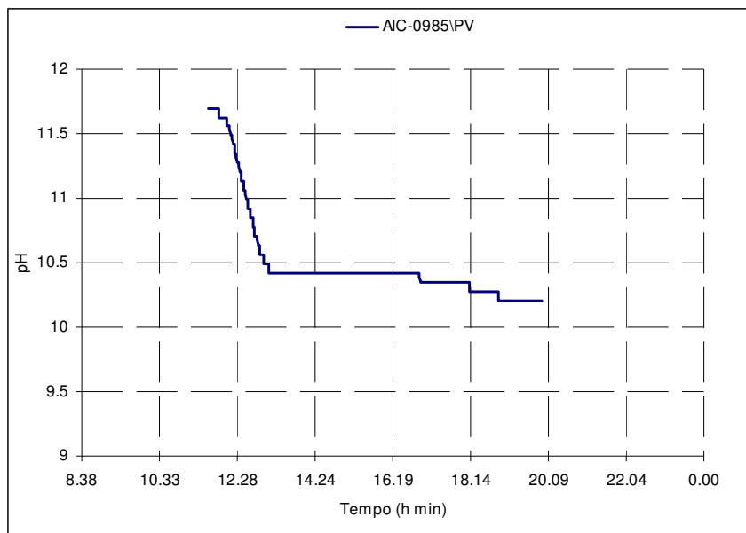
Figura 7.1. Andamento del pH all'interno del II stadio di desolfurazione a freddo.
