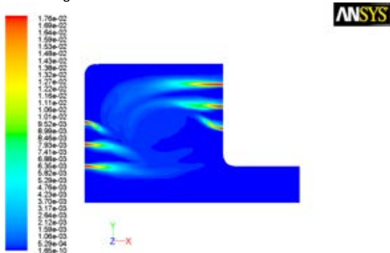
Figura 5.6 – Frazione di massa media di H 2
