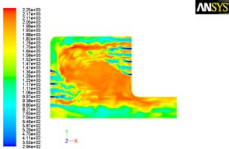
Figura 5.1 – Temperatura istantanea (K)
