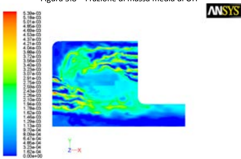
Figura 5.9 – Frazione di massa istantanea di OH
