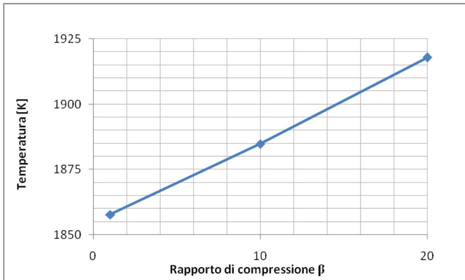
Figura 3.2 - Andamento della temperatura massima all'uscita del combustore al variare del rapporto di compressione
