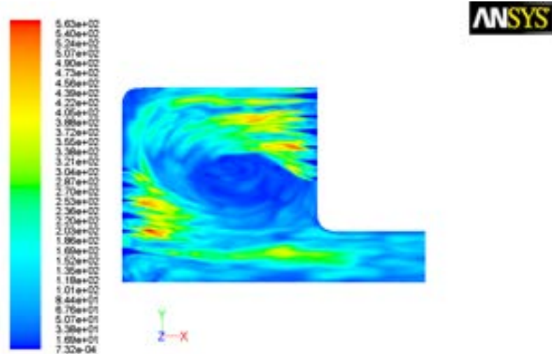
Figura 5.3 – RMS della temperatura (K)
