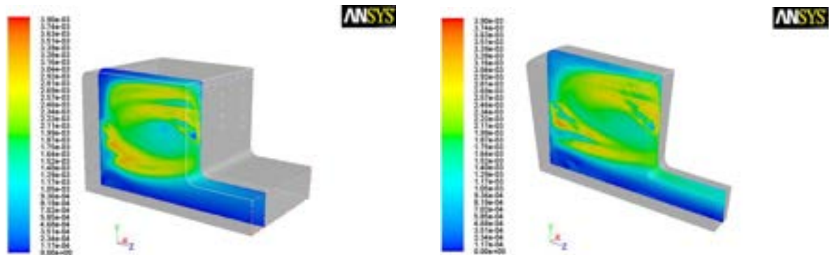
Figura 2.13 - Andamento della frazione di massa di OH nel settore rettificato e nel settore anulare
