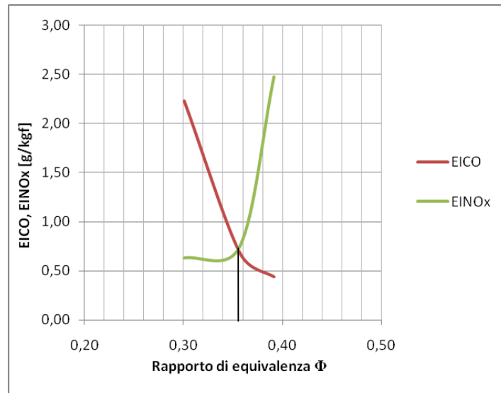
Figura 3.6 - Andamento degli indici EICO e EINO x in funzione del rapporto di equivalenza
