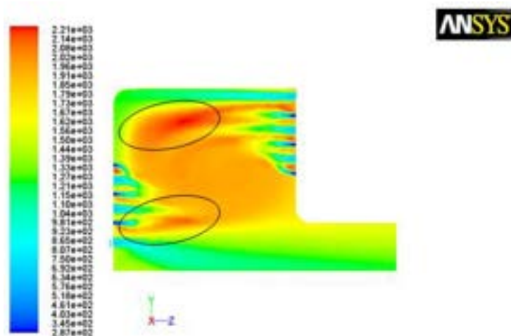
Figura 3.8 – Andamento della temperatura per p=20 bar e A/F=4.34
