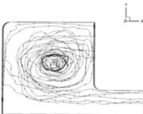
Figura 5.10 – Linee di flusso
