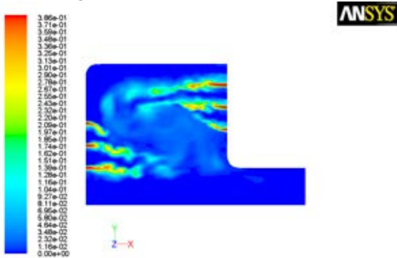
Figura 5.5 – Frazione di massa istantanea di CO
