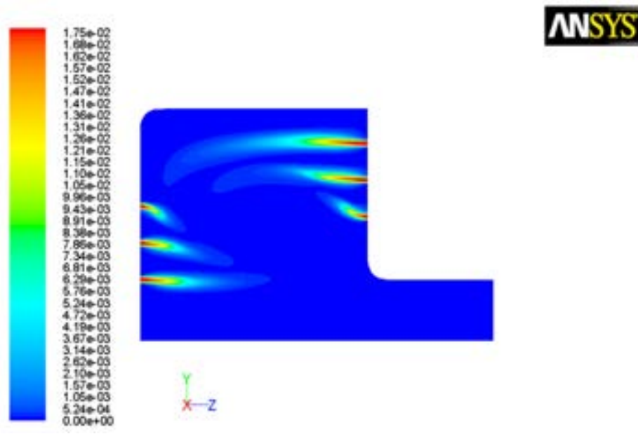
Figura 2.4 – Andamento della frazione massica di H_2 nella sezione centrale
