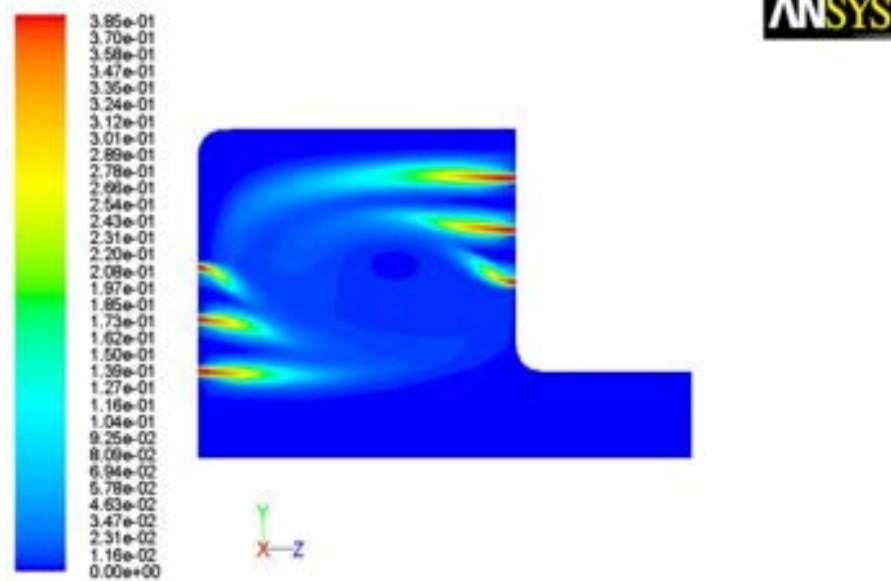
Figura 2.5 – Andamento della frazione massica di CO nella sezione centrale
