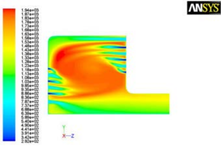
Figura 2.3 – Andamento della temperatura nella sezione centrale
