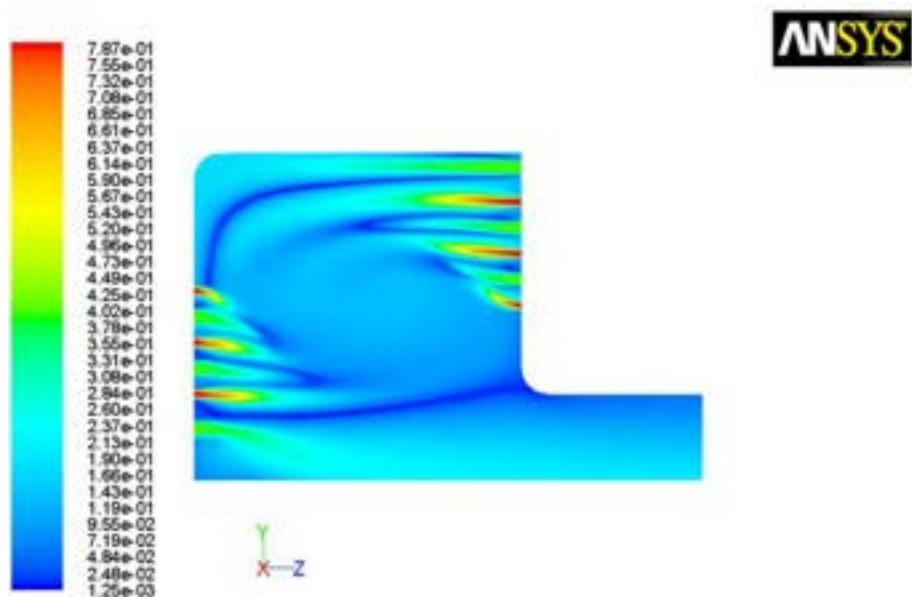
Figura 2.7 – Rappresentazione della grandezza MIX nella sezione centrale
