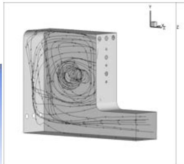
Figura 2.1 - Rappresentazione dei flussi che creano il vortice
