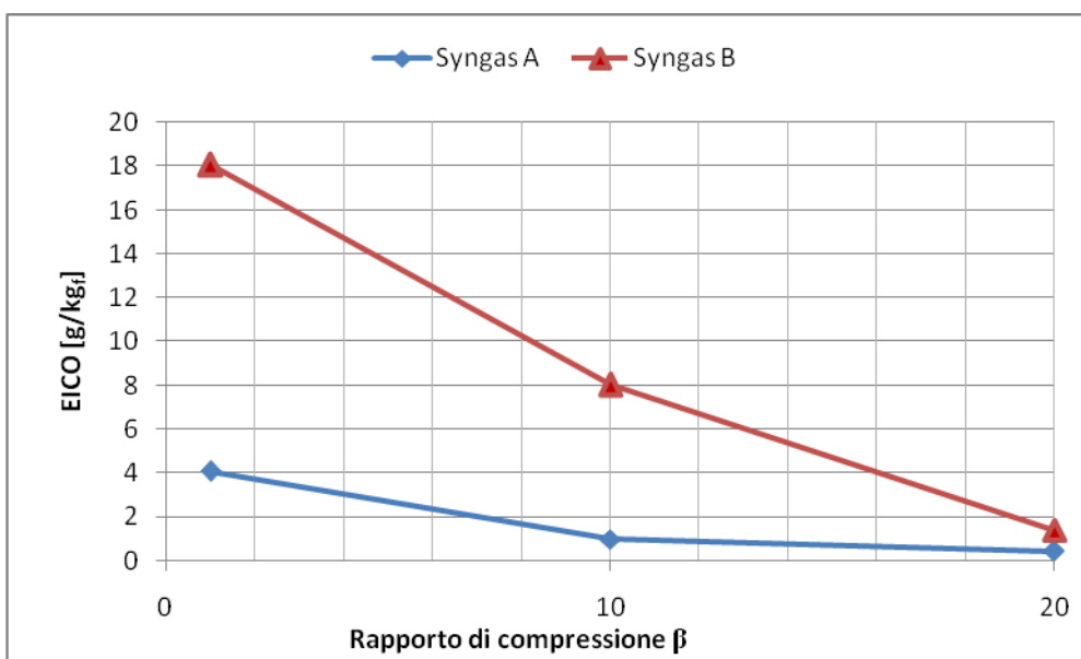
Figura 3.10 - Andamento EICO al variare del rapporto di compressione per i due syngas impiegati.
