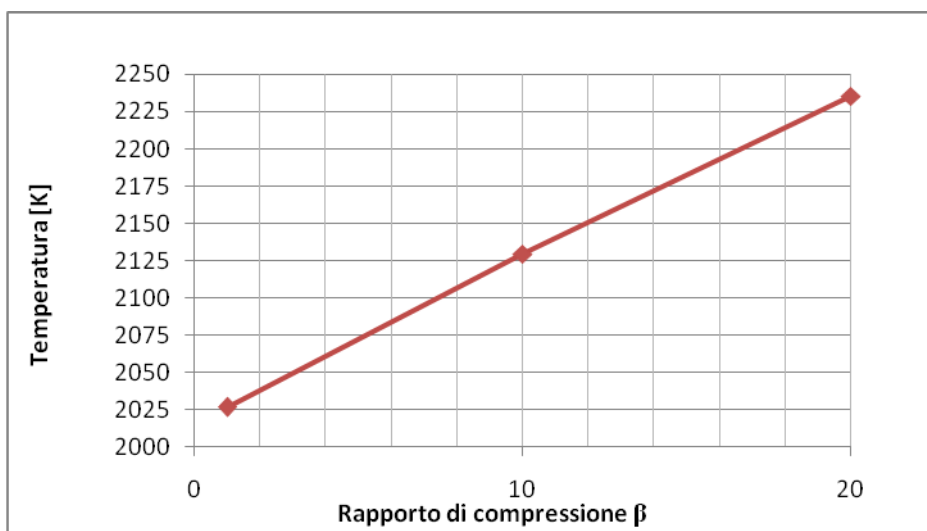
Figura 3.1 - Andamento della temperatura massima nel combustore al variare del rapporto di compressione
