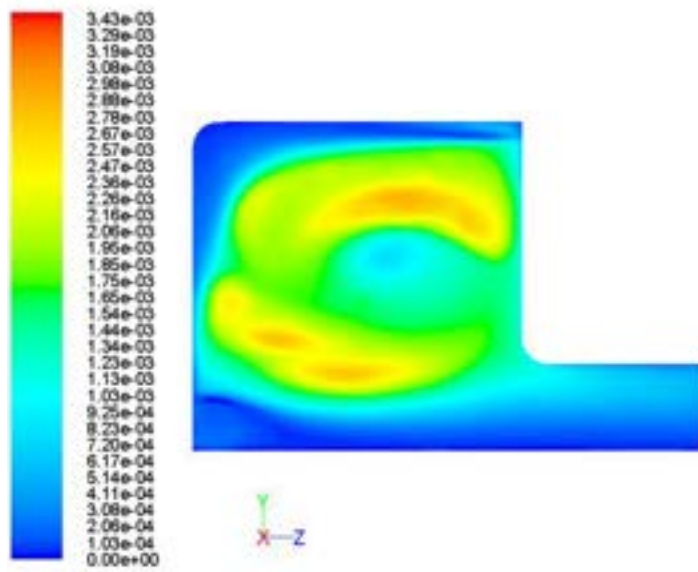
Figura 2.9 – Andamento della frazione massica di OH in una sezione intermedia
