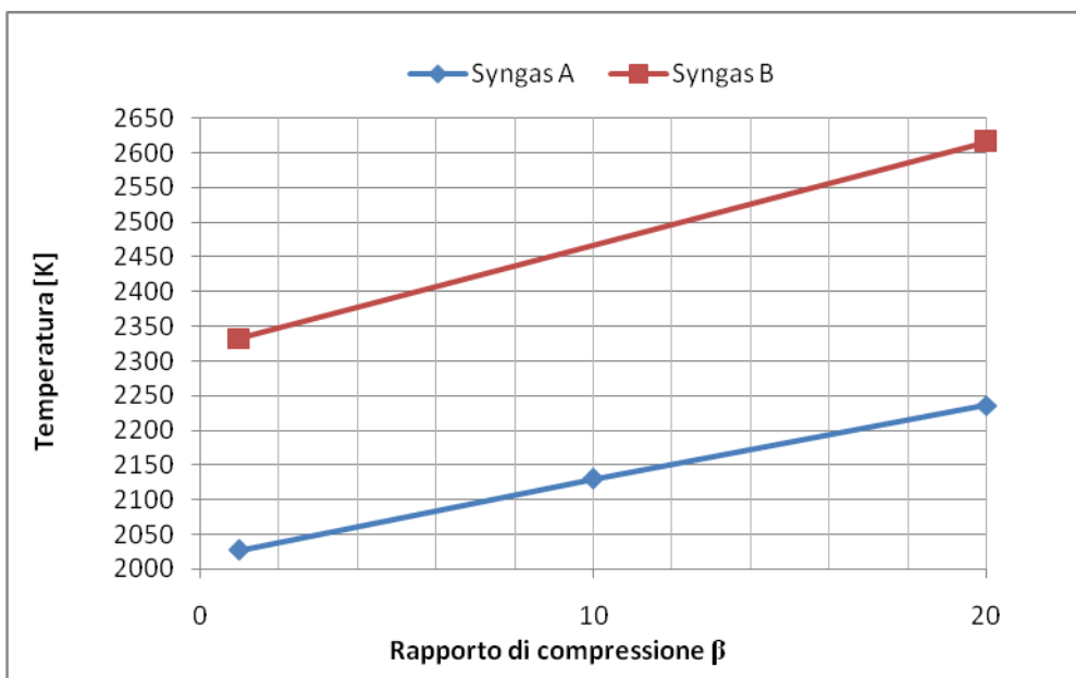
Figura 3.9 - Andamento della temperatura massima nel combustore al variare del rapporto di compressione per i due syngas impiegati
