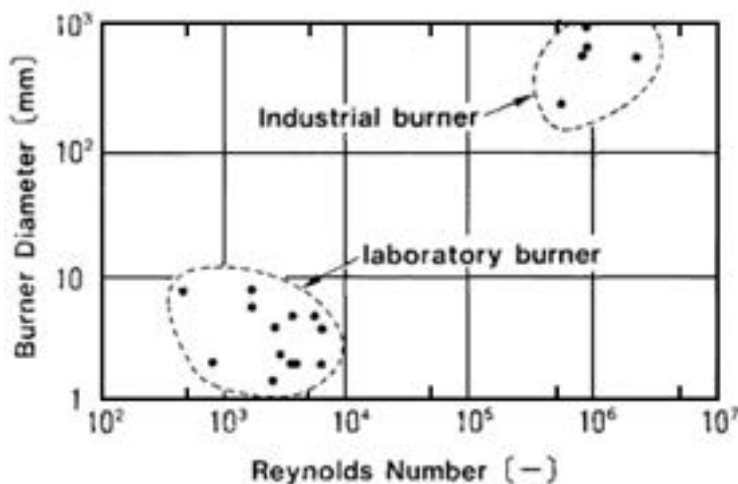
Figura 4.1- Confronto fra combustori da laboratorio e industriali
