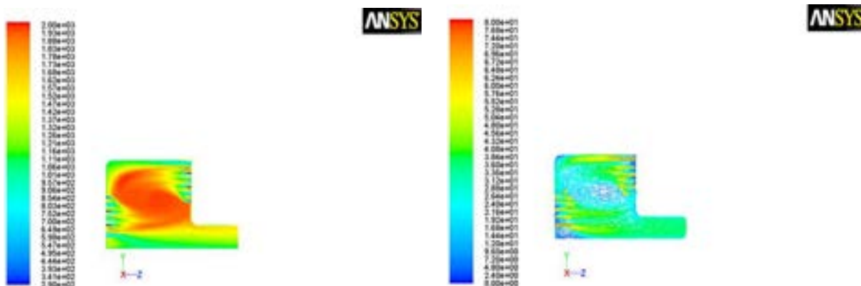
Figura 4.2 - Andamento di temperatura e velocità nel combustore di dimensioni dimezzate
