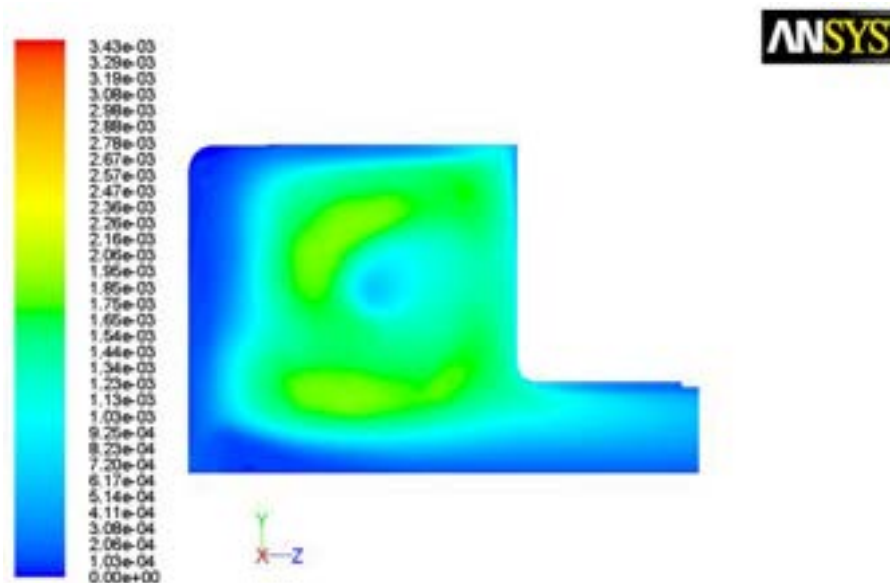
Figura 2.10 – Andamento della frazione massica di OH nella sezione estrema
