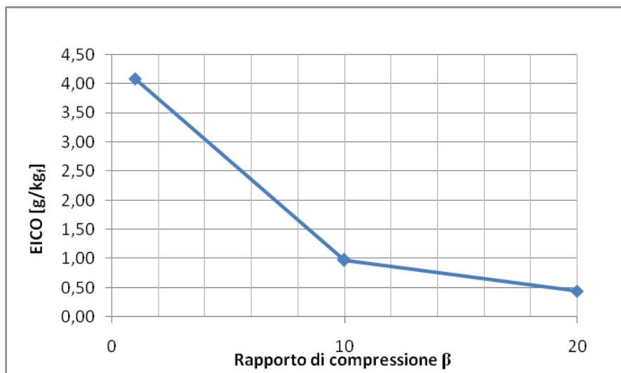
Figura 3.3 - Andamento EICO al variare del rapporto di compressione
