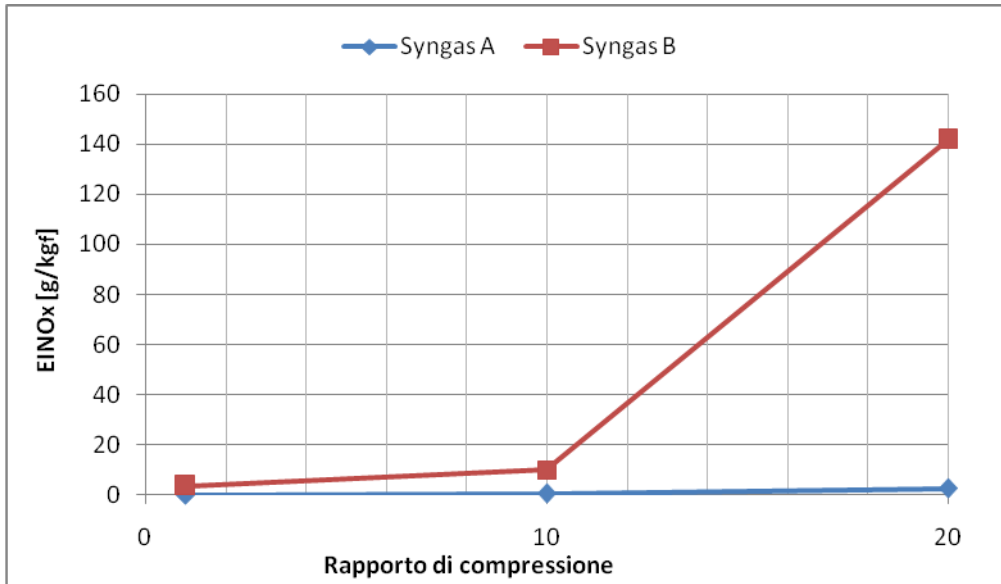
Figura 3.11 - Andamento EINO_x al variare del rapporto di compressione per i due syngas impiegati.
