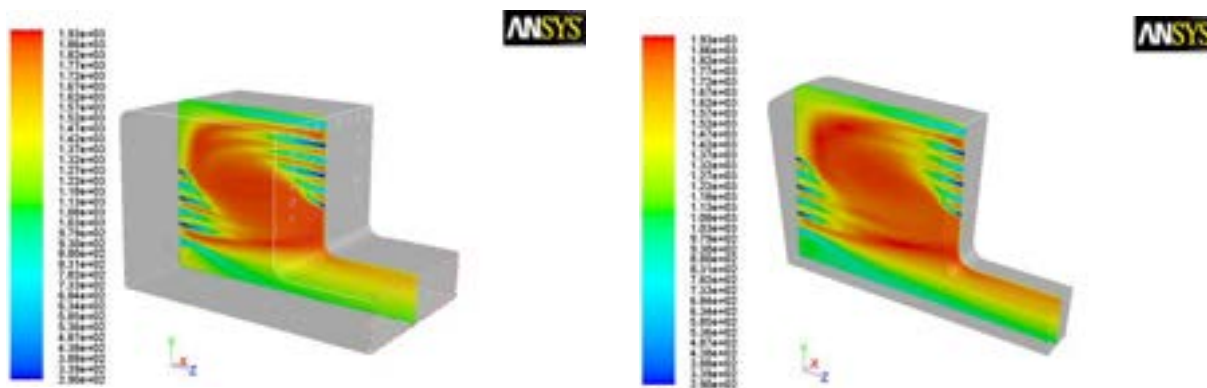
Figura 2.11 - Andamento della temperatura nel settore rettificato e nel settore anulare
