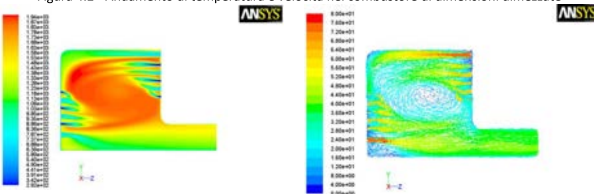
Figura 4.3 - Andamento di temperatura e velocità nel combustore di dimensioni normali
