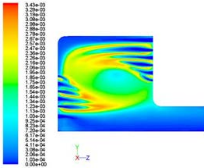
Figura 2.8 – Andamento della frazione massica di OH nella sezione centrale
