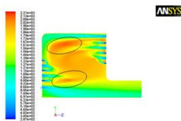
Figura 3.7 – Andamento della temperatura per p=10 bar e A/F=4.34
