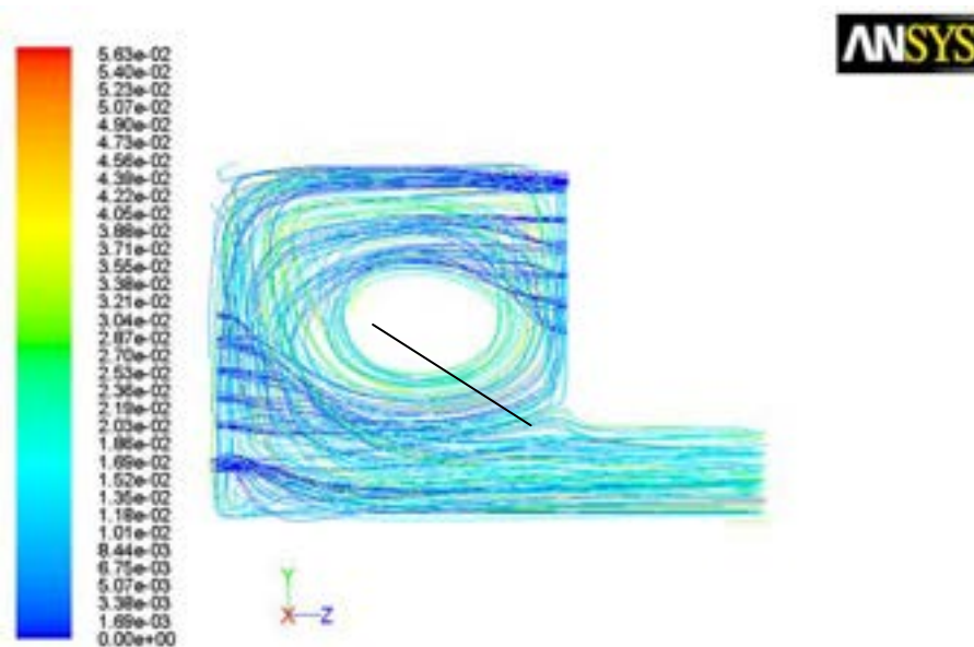
Figura 2.6 – Linee di flusso
