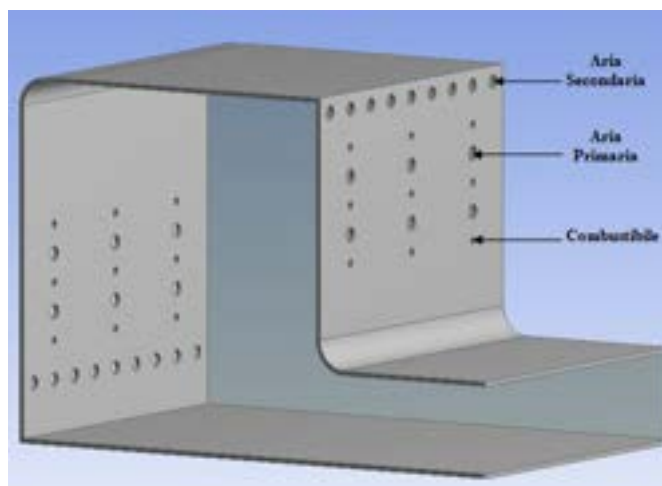
Figura 1.1 - Settore rettificato del bruciatore anulare
