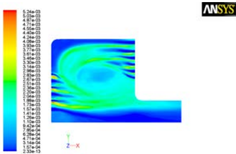
Figura 5.8 – Frazione di massa media di OH
