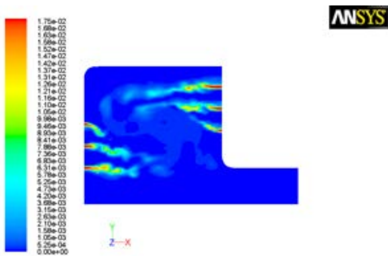
Figura 5.7 – Frazione di massa istantanea di H_2
