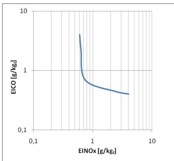
Figura 3.5 - Andamento delle emissioni di CO e NO x al variare delle condizioni operative
