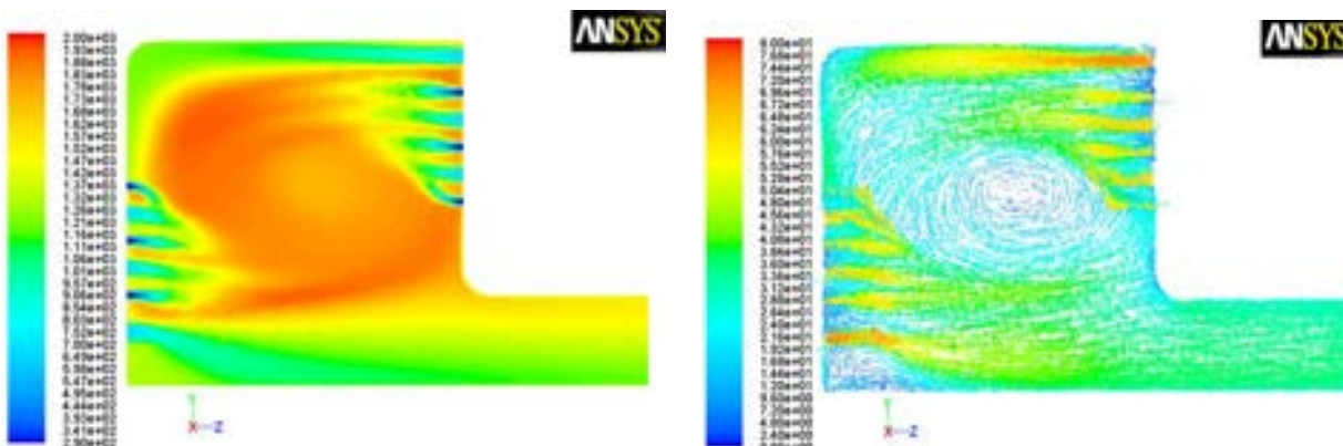
Figura 4.4 - Andamento di temperatura e velocità nel combustore di dimensioni raddoppiate
