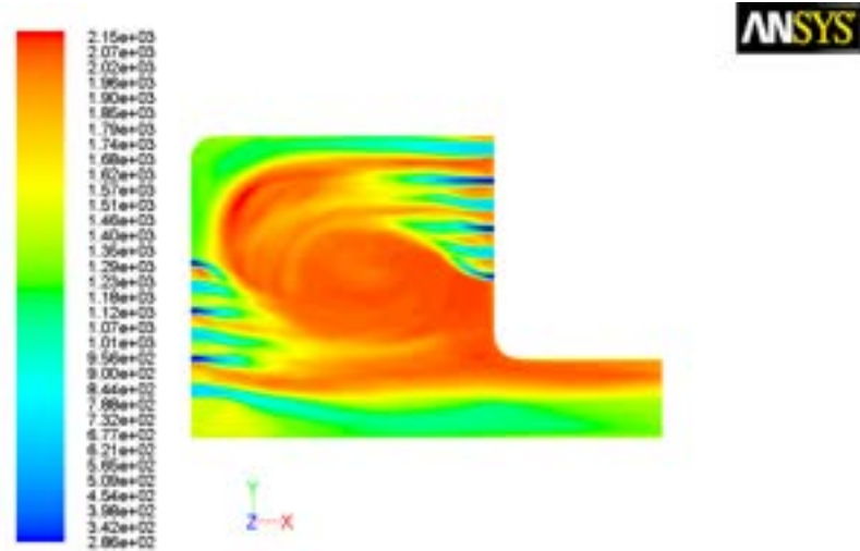
Figura 5.2 – Temperatura media (K)
