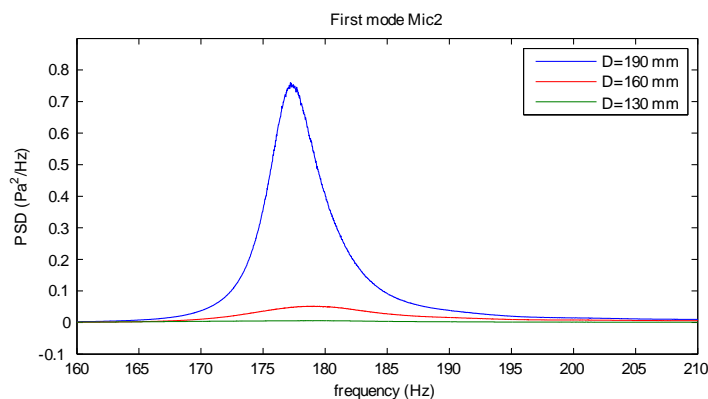
Figura 2.33: confronto delle PSD del primo modo al variare della profondità D.
