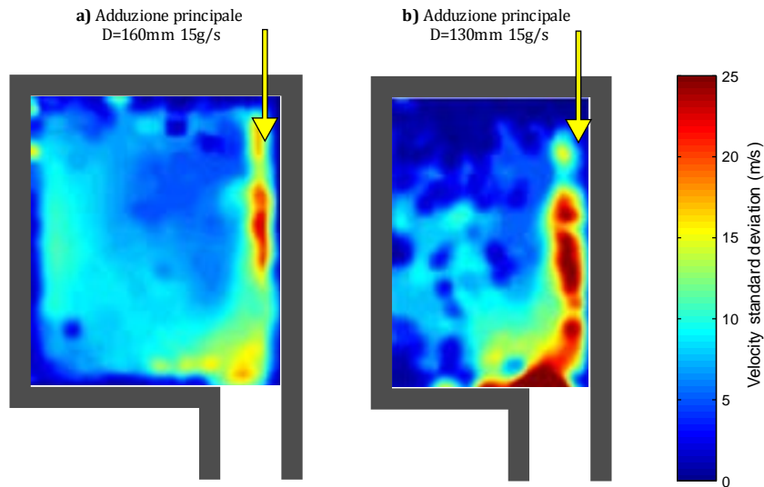
Figura 2.48: deviazione standard della velocità con portata di 15 g/s al variare della profondità della cavità: a) D=160 mm; b) D=130 mm.
