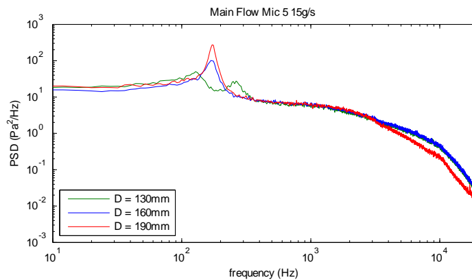
Figura 2.37: Confronto tra gli spettri aeroacustici del TVC alimentato tramite il flusso principale al variare di D.
