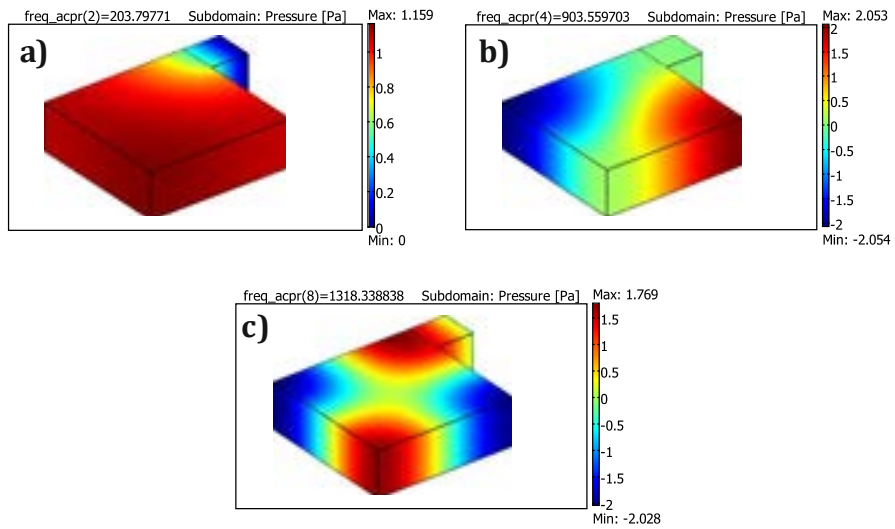
Figura 2.41: Andamento della pressione per i primi tre modi propri con D=190 mm.
