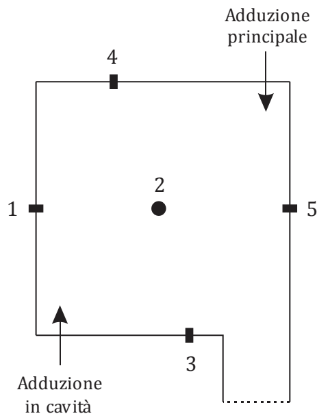
Figura 2.13: Disposizione dei microfoni nel TVC per misure acustiche.
