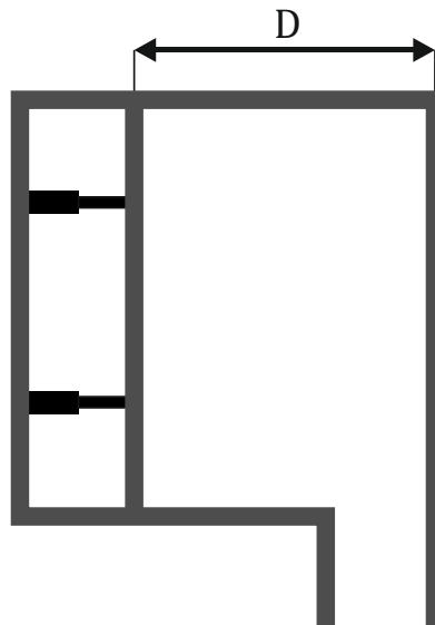
Figura 2.12: Schematizzazione del sistema di movimentazione della paratia per variare la profondità della cavità.
