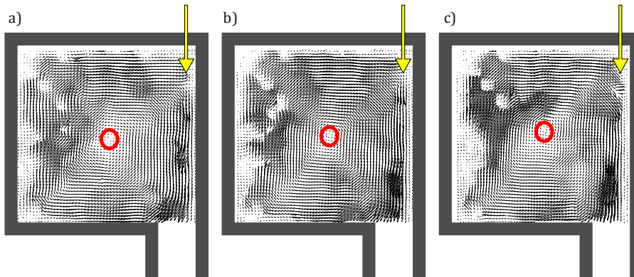
Figura 2.49: Campi vettoriali istantanei della velocità con D=190 mm e portata di 15 g/s. Il cerchio rosso indica la posizione del centro del vortice.
