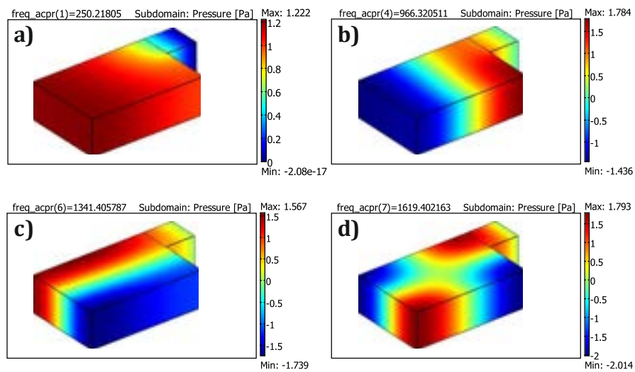
Figura 2.43: andamento della pressione per i primi quattro modi propri con D=130 mm.
