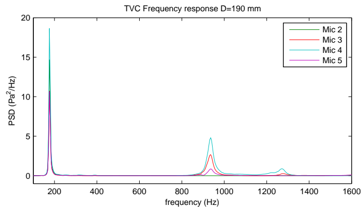
Figura 2.32: risposta in frequenza del TVC per D=190 mm.
