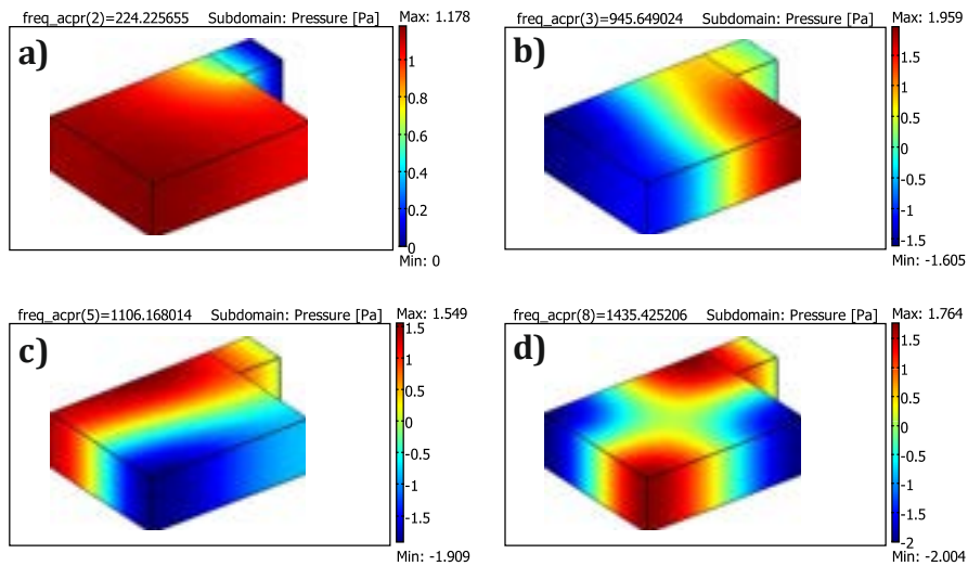
Figura 2.42: andamento della pressione per i primi quattro modi propri con D=160 mm.
