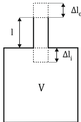
Figura 2.3: Rappresentazione dei fattori correttivi dell'imboccatura.
