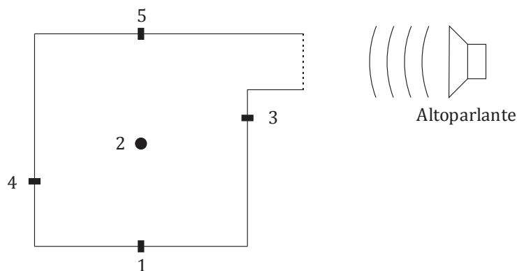
Figura 2.31: Disposizione dell'altoparlante e dei microfoni per il test modale.
