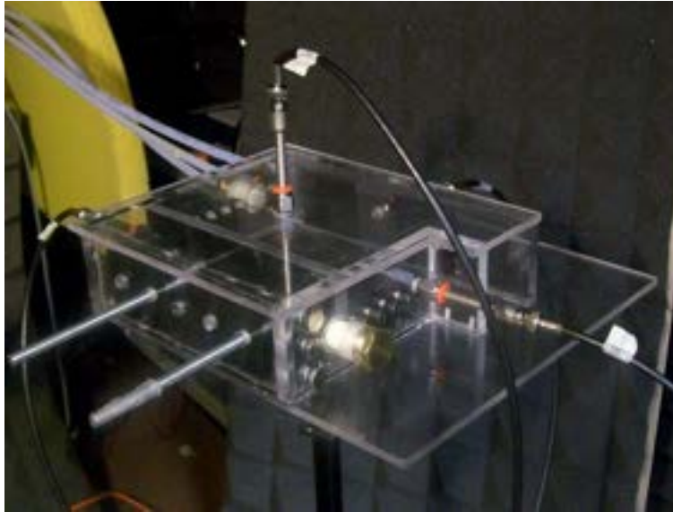
Figura 2.11: Modello di combustore TVC per misure acustiche.
