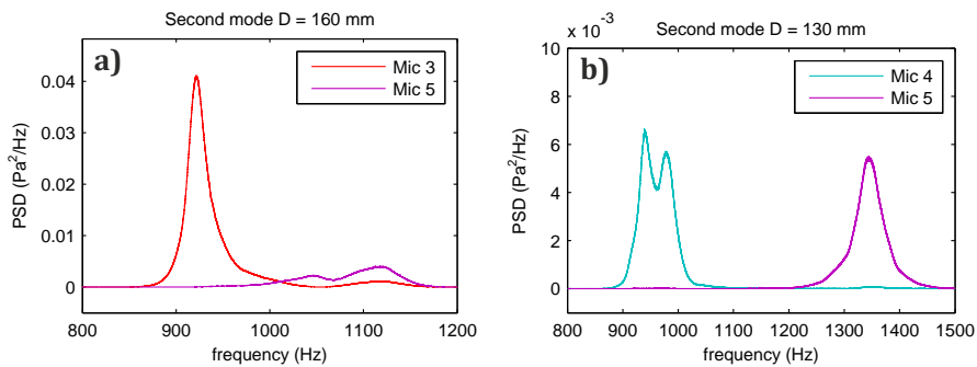
Figura 2.35: separazione dei picchi del secondo modo al diminuire della profondità della cavità: a) D=160 mm, b) D=130 mm.
