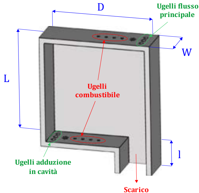
Figura 2.4: Geometria del combustore TVC oggetto di studio.
