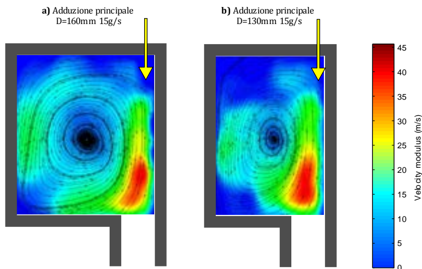
Figura 2.45: campi di velocità con portata di 15 g/s, utilizzando una dimensione della finestra di 32 pixel, al variare della profondità della cavità: a) D=160 mm; b) D=130 mm.
