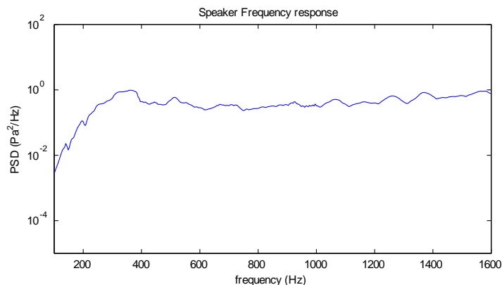
Figura 2.30: Risposta in frequenza dell'altoparlante nell'intervallo 100-1600 Hz.
