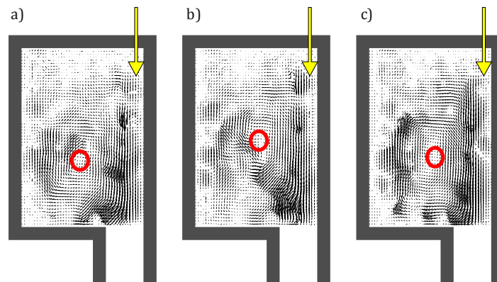
Figura 2.50: Campi vettoriali istantanei della velocità con D=130 mm e portata di 15 g/s. Il cerchio rosso indica la posizione del centro del vortice.
