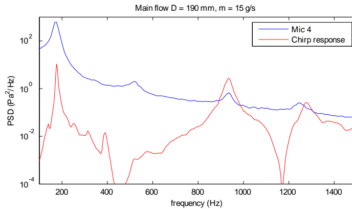
Figura 2.36: Sovrapposizione tra risposta in frequenza del TVC con D=190 mm e spettro aeroacustico con adduzione principale e portata 15 g/s.
