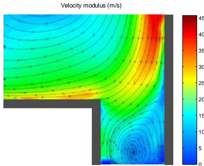
Figura 2.46: particolare del campo di velocità del condotto di scarico. Si noti la bolla di ricircolo in corrispondenza della sezione di uscita.
