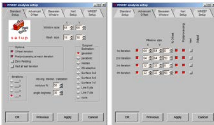
Figura 2.24: Schermate delle impostazioni del software PIVDEF.
