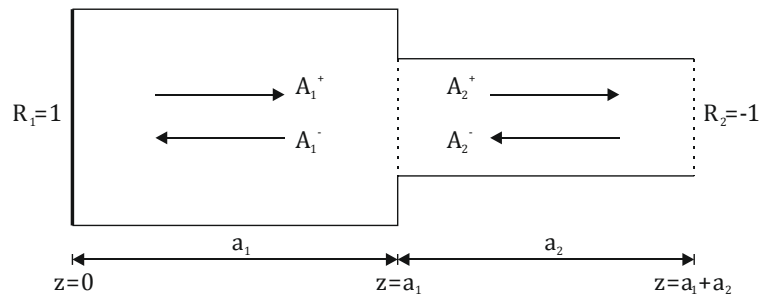
Figura 2.1: configurazione double duct.
