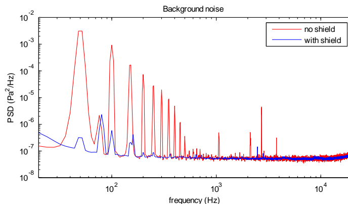
Figura 2.26: Confronto degli spettri del background acustico con e senza gabbia di Faraday.
