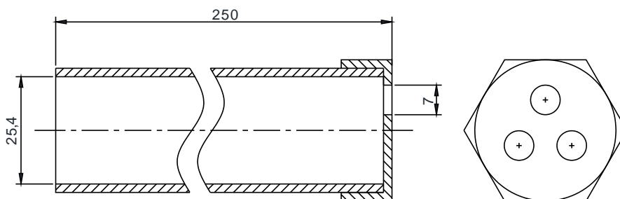
Figura 2.9: Collettore cilindrico.
