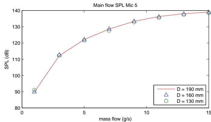
Figura 2.38: Confronto dei SPL con adduzione principale al variare della profondità D.
