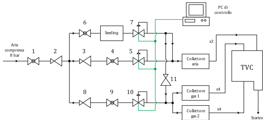
Figura 2.5: Schema dell'impianto di adduzione del combustore.
