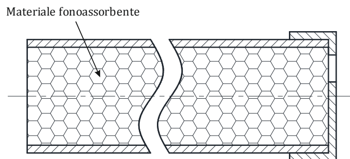
Figura 2.27: Disposizione del materiale fonoassorbente all'interno del collettore cilindrico della linea di adduzione dell'aria.
