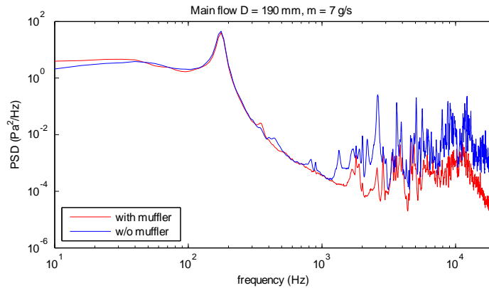
Figura 2.28: Confronto tra le PSD del microfono 2 nel caso di TVC con adduzione principale, portata 7 g/s e profondità D=190 mm, con e senza muffler.
