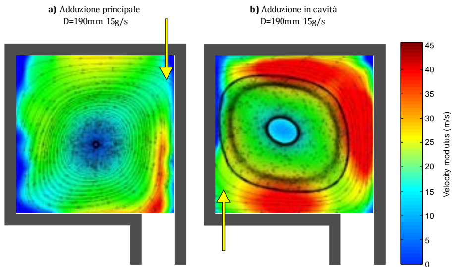
Figura 2.44: campi di velocità con D=190 mm e portata di 15 g/s, utilizzando una dimensione della finestra di 32 pixel, al variare del tipo di adduzione: a) adduzione principale; b) adduzione in cavità.
