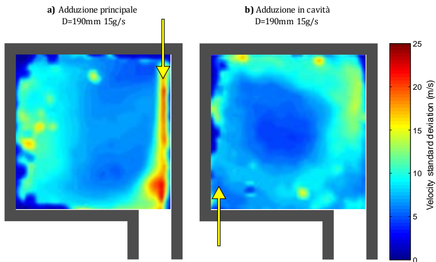
Figura 2.47: deviazione standard della velocità con D=190 mm e portata di 15 g/s al variare del tipo di adduzione: a) adduzione principale; b) adduzione in cavità.
