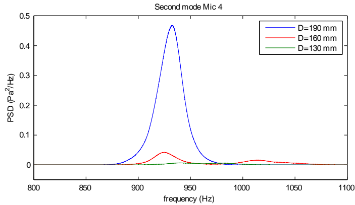
Figura 2.34: confronto delle PSD del secondo modo al variare della profondità D.
