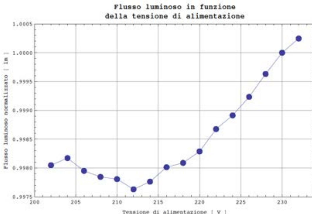
Figura 39 Variazione del flusso luminoso (normalizzato) emesso dall'apparecchio di illuminazione in funzione della tensione di alimentazione.
