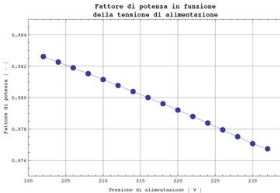
Figura 41 Variazione del fattore di potenza elettrica dell'apparecchio di illuminazione in funzione della tensione di alimentazione.
