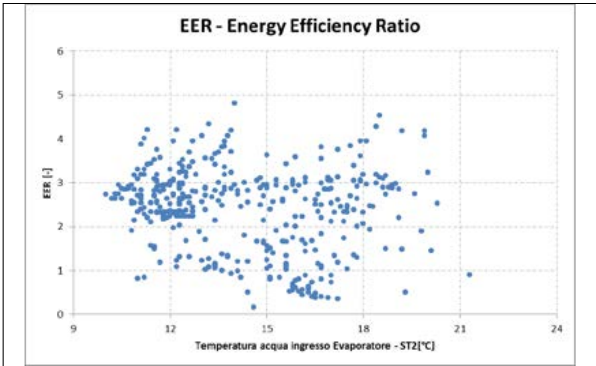
FIGURA 2.22 b): Andamento delle prestazioni della pompa di calore in funzione di ST2
