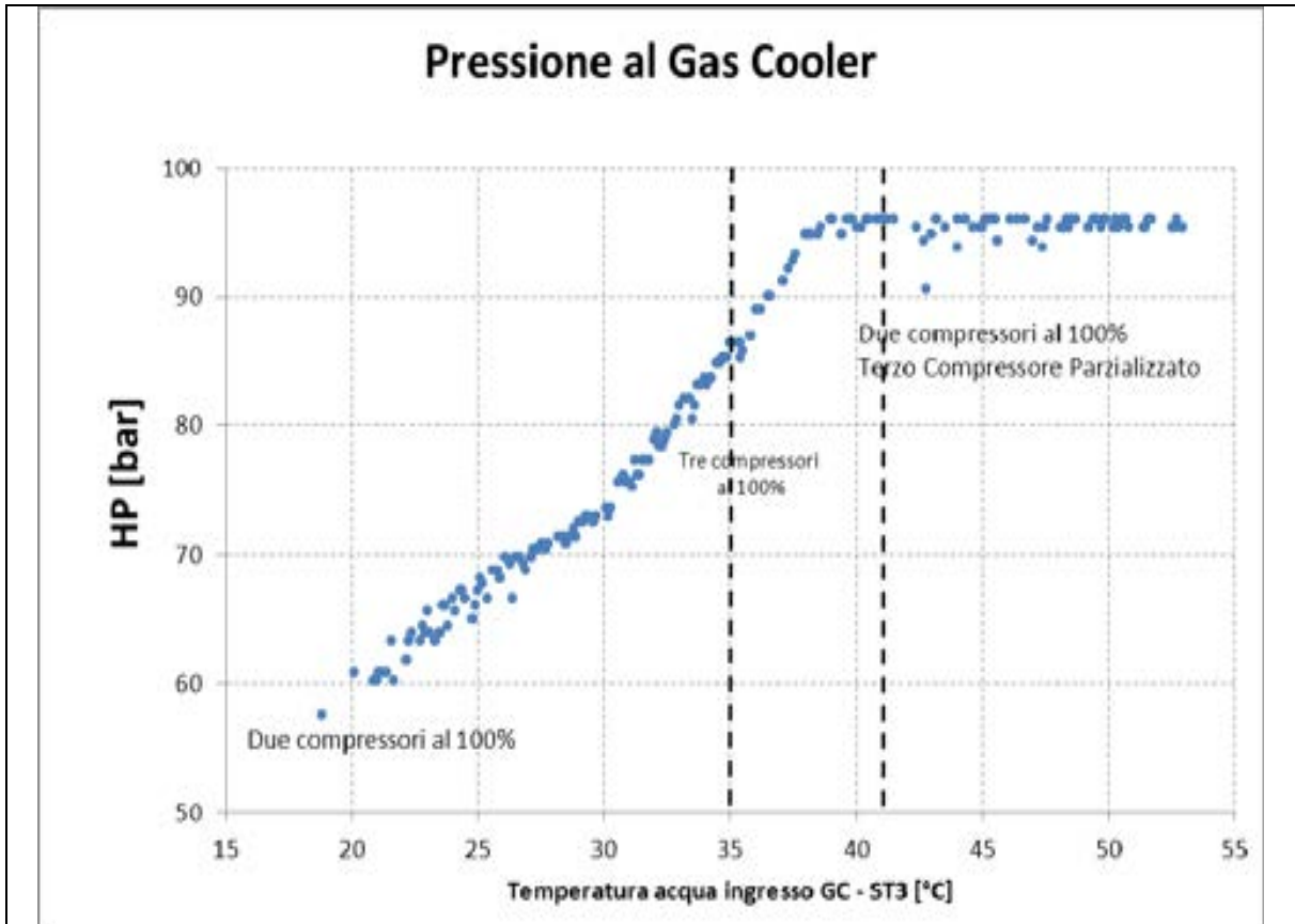
FIGURA 2.3: Andamento della pressione al gas cooler in funzione della temperatura dell'acqua in ingresso al GC
