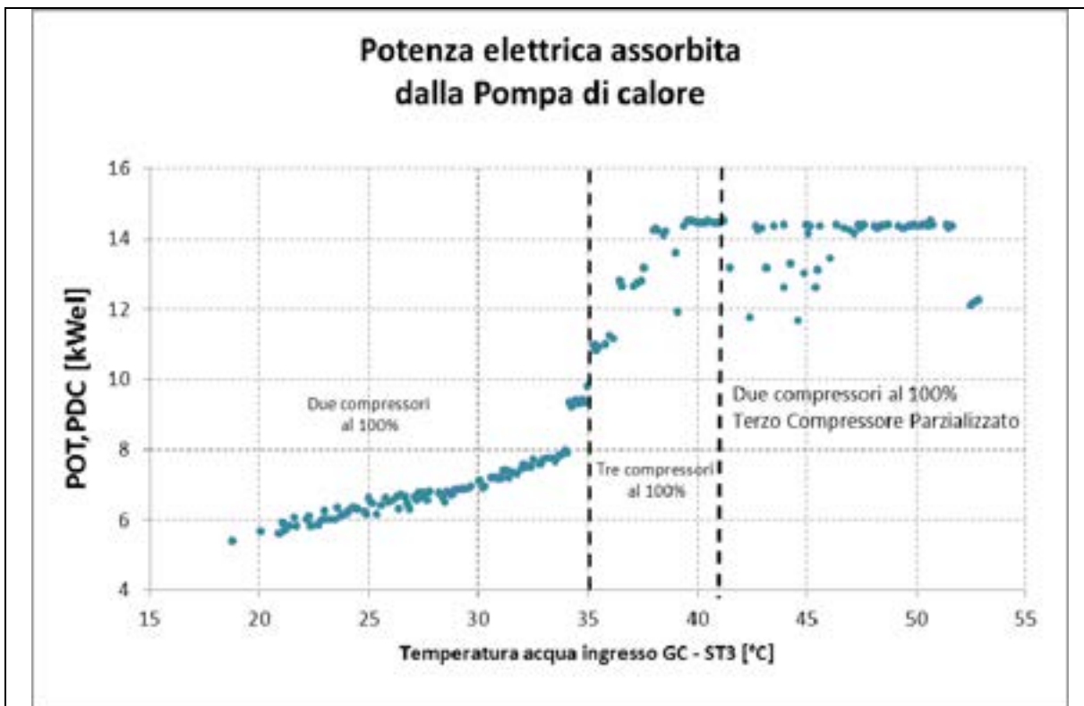
FIGURA 2.7: Andamento della potenza elettrica assorbita dalla Pompa di calore in funzione della temperatura dell'acqua in ingresso al GC
