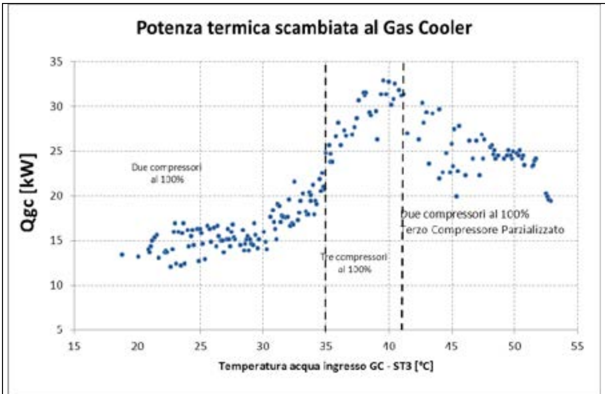
FIGURA 2.8: Andamento della potenza termica scambiata al GC in funzione della temperatura dell'acqua in ingresso al Gas cooler
