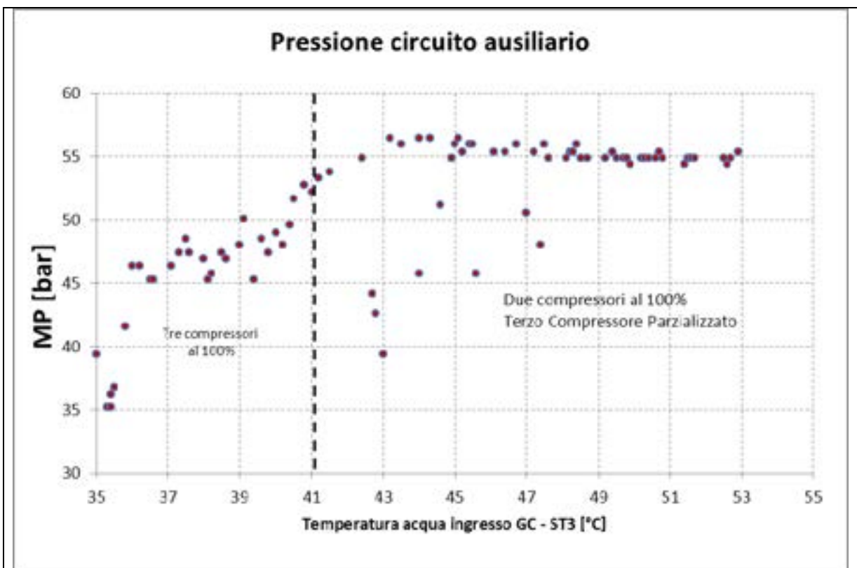
FIGURA 2.4: Andamento della pressione del circuito ausiliario in funzione della temperatura dell'acqua in ingresso al gas cooler
