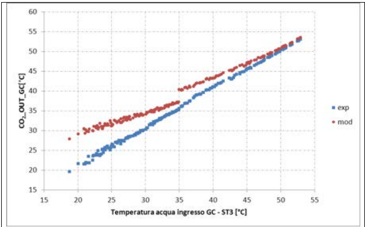
FIGURA 4.9: Confronto tra i valori forniti dal modello e i valori sperimentali per la temperatura della CO 2 in uscita dal gas cooler al variare di ST3
