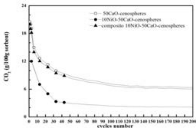
Figura 2. Cicli di carbonatazione/ciclazione di CaO-cenosfera (50-50), CSCM, e un composito di CSCM.
