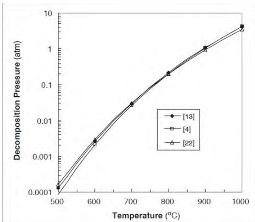
Figura 3 Andamento della pressione della CO_2 di equilibrio [6]
