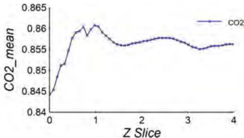
Figura 12 Concentrazione molare media della CO 2 lungo il reattore dopo 60 s
