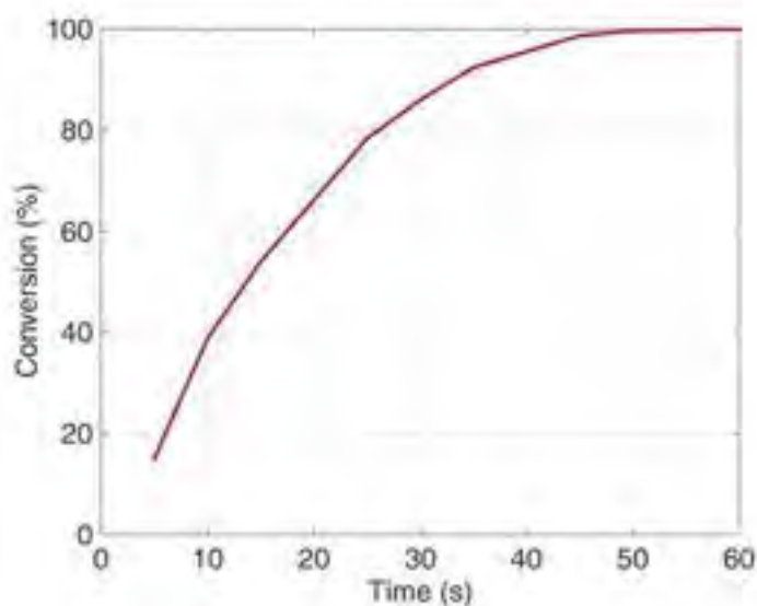
Figura 7 Andamento della conversione ottenuta dalla simulazione CPFD
