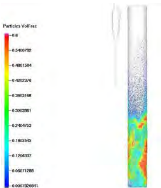
Figura 9 Frazione di volume della fase solida dopo 60 s
