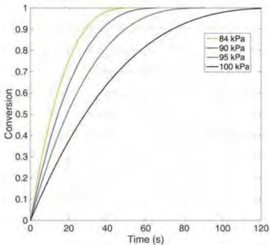
Figura 4 Andamento della conversione a 900 °C
