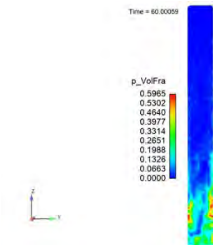
Figura 10 Frazione volumetrica della fase solida
