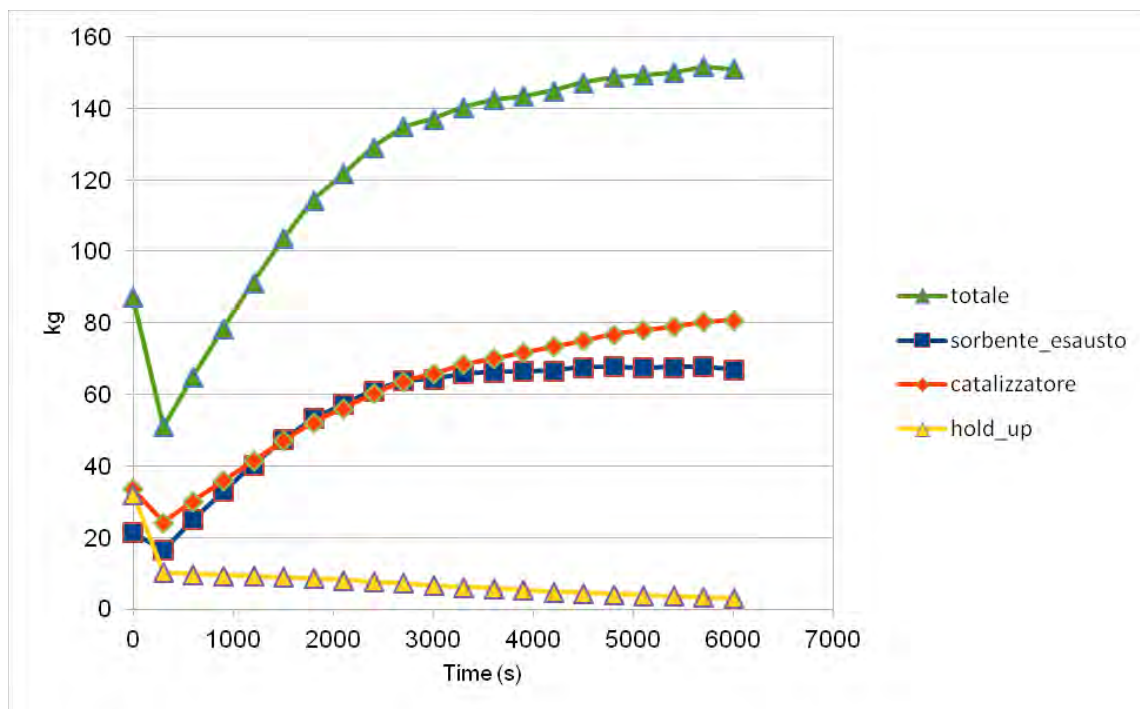
Figura 14 Andamento della massa del letto in funzione del tempo
