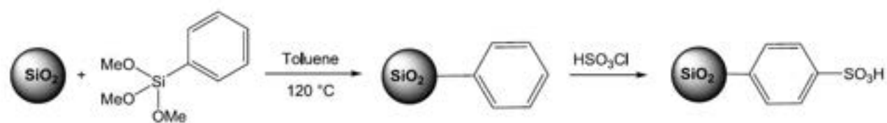
Schema 2. Procedura di sintesi del catalizzatore SiO 2 -C 6 H 4 -SO 3 H
