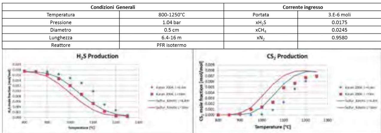
Figura 2 Condizioni operative di un reattore PFR isotermo con reagenti H 2 S e CH 4 e confronto fra dati sperimentali e previsione del modello cinetico
