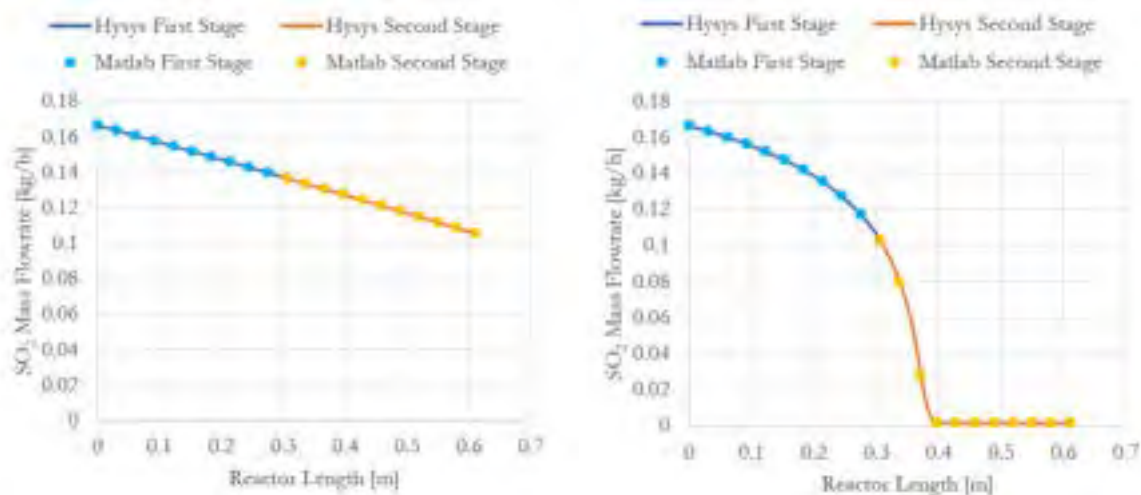
Figura 4. Confronto tra le portate massiche di SO 2 tra Aspen e Matlab - caso isoterma e adiabatico.
