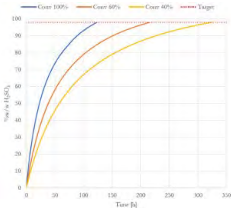
Figura 8.3. Profilo temporale di concentrazione dell'acido solforico vs tempo e conversione di \text{SO}_2 .
