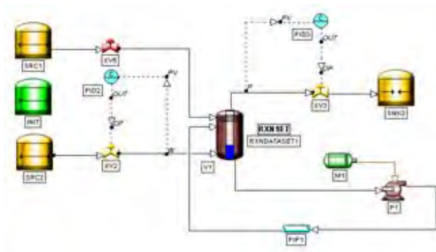
Figura 8.1. Modello della colonna sviluppato con SimSci DYNsim.
