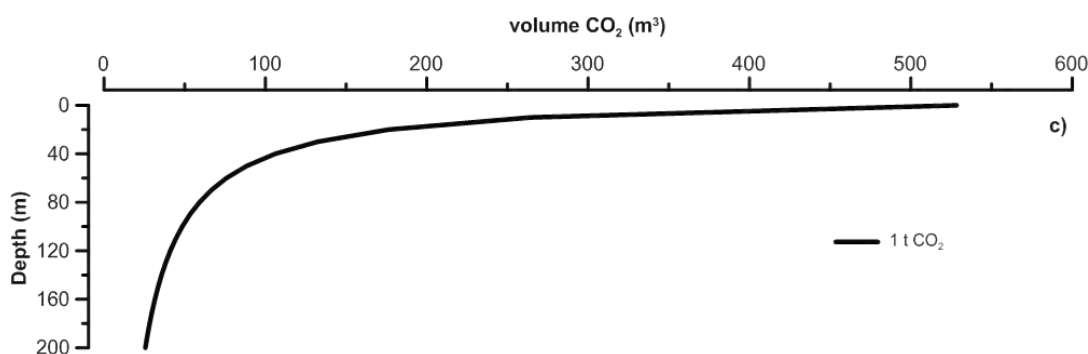
Figura 20 Variazione di volume di 1 t di CO 2 con la profondità, assumendo un gradiente costante di pressione idrostatica.
