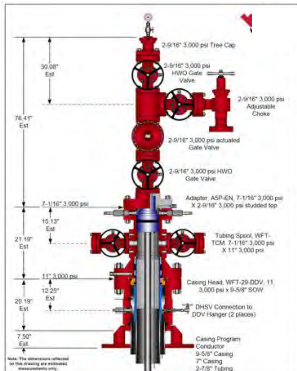
Figura 18 Testa pozzo con X-Mas Tree. Per i diametri del casing, si veda la sezione 7.1.1.
