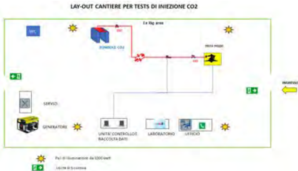
Figura 26 Layout di cantiere.
