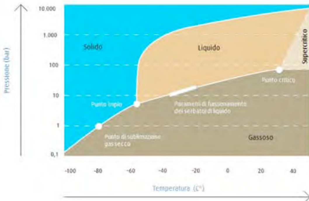
Figura 1: Stati di aggregazione in funzione della temperatura e della pressione della CO 2 .
