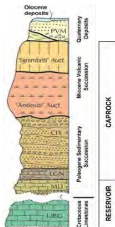
Figura 1. Stratigrafia del Bacino carbonifero del Sulcis (modificato da ISPRA, 2012).
