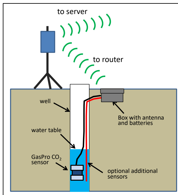
Figura 18. Disegno schematico che mostra il layout e l'implementazione di un sistema GasPro Network 3 in un pozzo.
