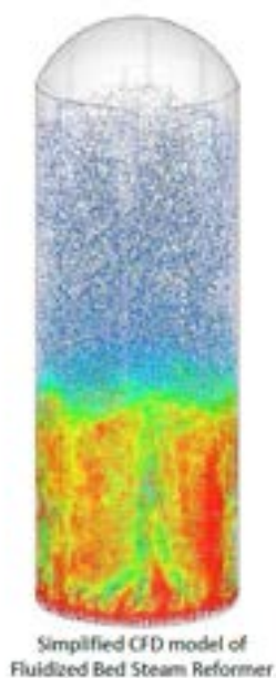
Figura 4 Modello semplificato della distribuzione del calore in letto fluido a vapore
