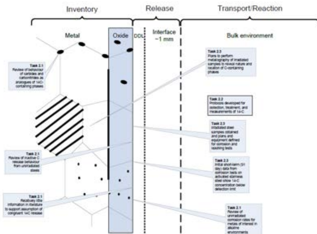
Figura 12 Schema di sintesi dei progressi relativi al termine sorgente di c14 negli acciai
