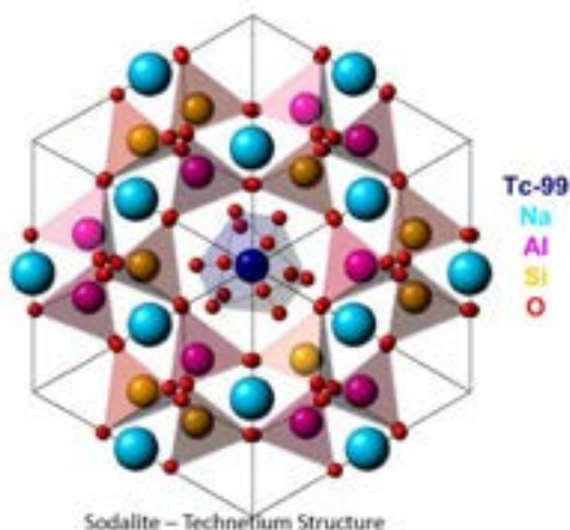
Figura 6 Schema della struttura minerale sodalite che incapsula il tecnezio
