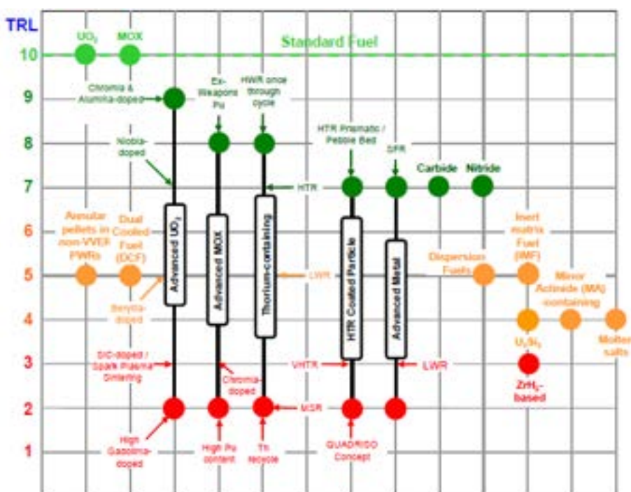
Figura 11 Evoluzione delle nuove tipologie di combustibile ed il loro Technology Readiness Level (TRL) – David Hambley SNTEP Meeting 2014
