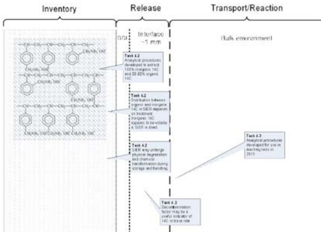
Figura 14 - Schema di sintesi dei progressi relativi al termine sorgente di C14 nelle resine a scambio ionico
