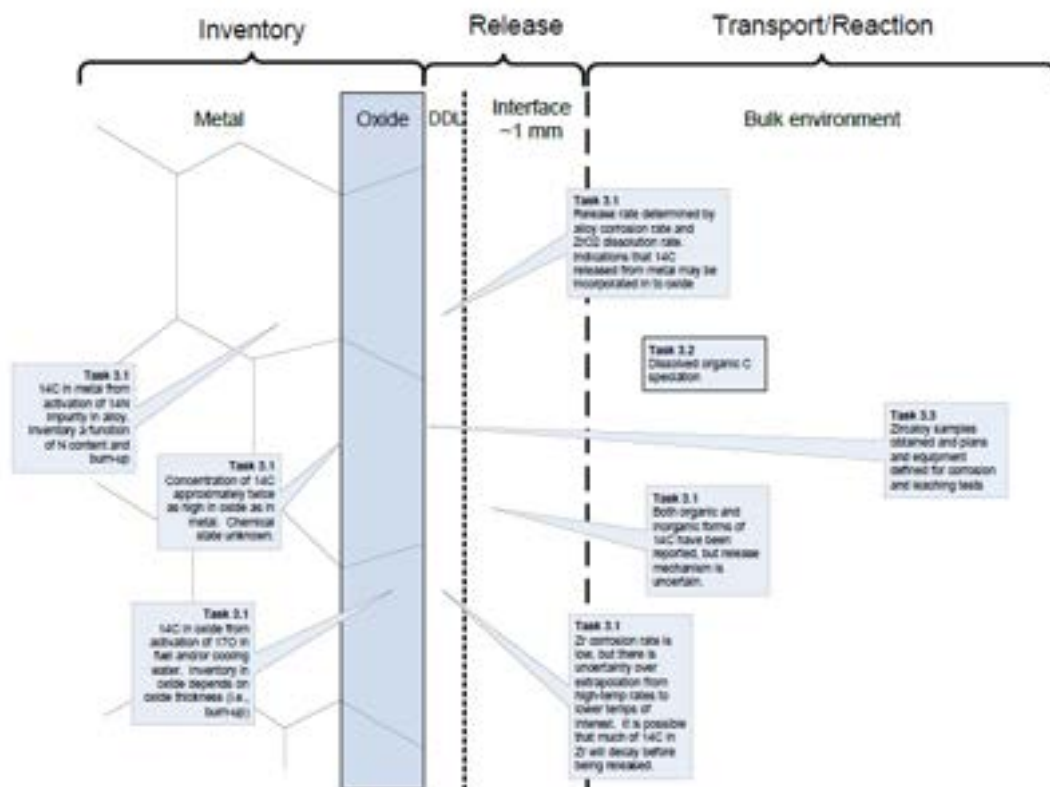
Figura 13 - Schema di sintesi dei progressi relativi al termine sorgente di C14 nelle zircalloy
