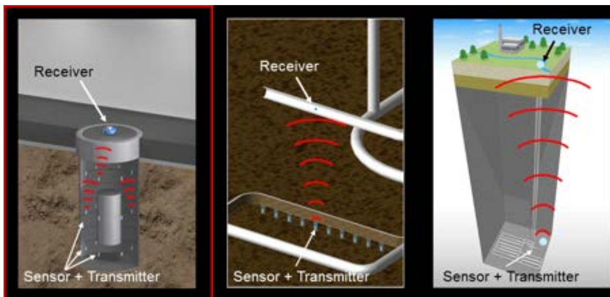
Figura 17 - Esempi di progettazione di sistemi di trasmissione wireless per MODERN2020
