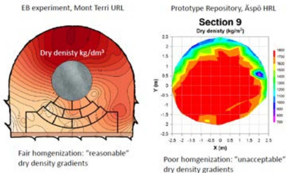
Figura 8 Evoluzione temporale del sistema di riempimento a bentonite dopo la saturazione, in due diversi esperimenti (Mont Terri e Äspö) – SKB Patrick Sellin
