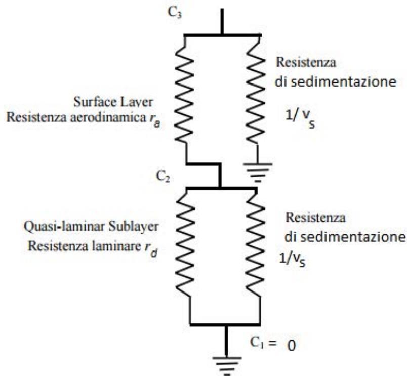
Figura 3. – Analogia elettrica per la deposizione secca nel caso di particella. Per diametri della particella d_p > 1 \text{ }\mu\text{m} il parametro C_c tende al valore unitario. eq. (18) il parametro \alpha_{air}
