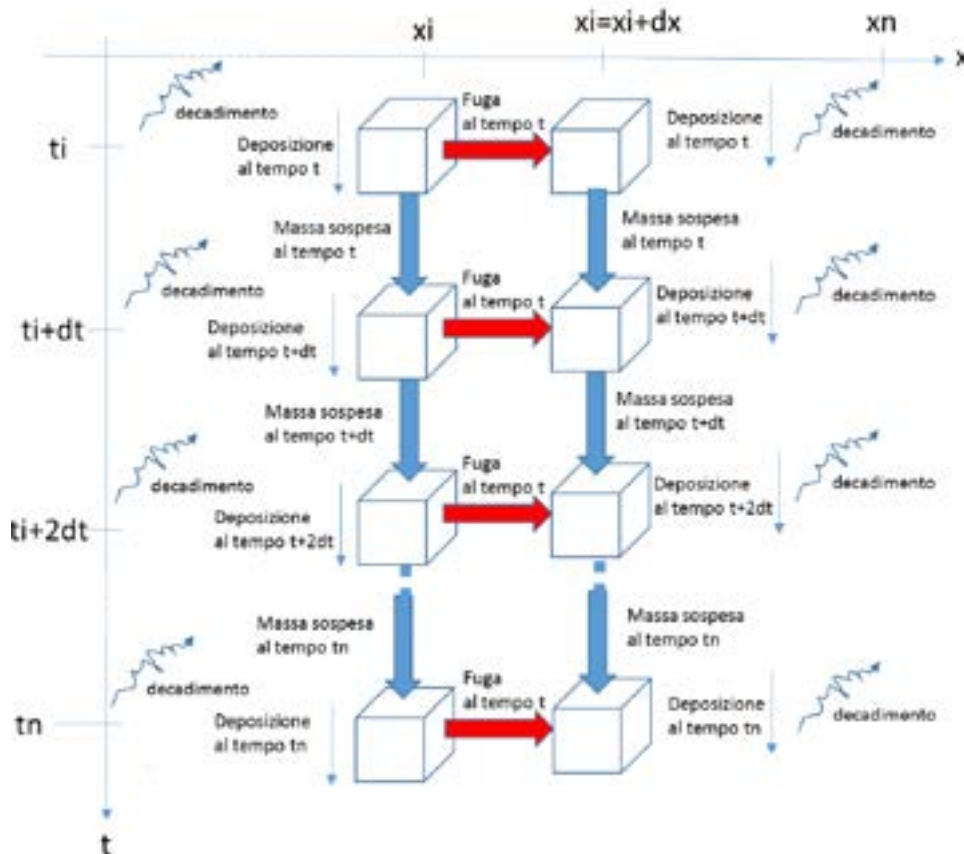
Fig. 1- Schematizzazione del calcolo della concentrazione di inquinante effettuata dal codice RADCAL nel volume di riferimento al variare del tempo e dello spazio.
