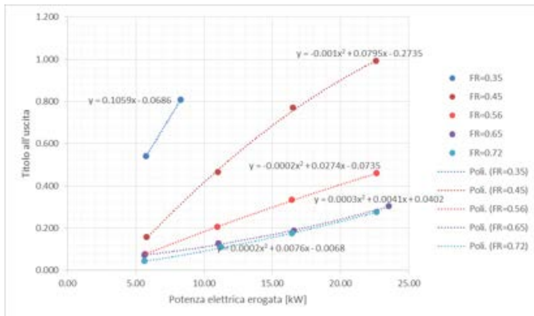
Figura 26 – Titolo all'uscita del GV in funzione della potenza elettrica e del Filling Ratio.
