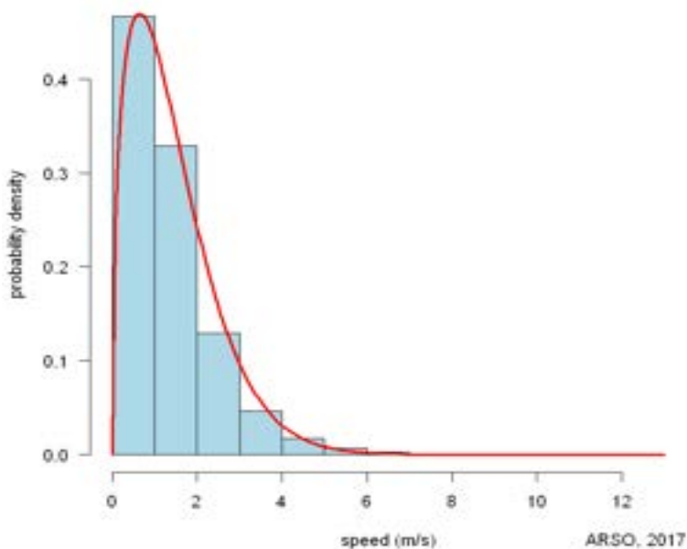
Figura 11: Distribuzione di probabilità della velocità del vento – Krško
