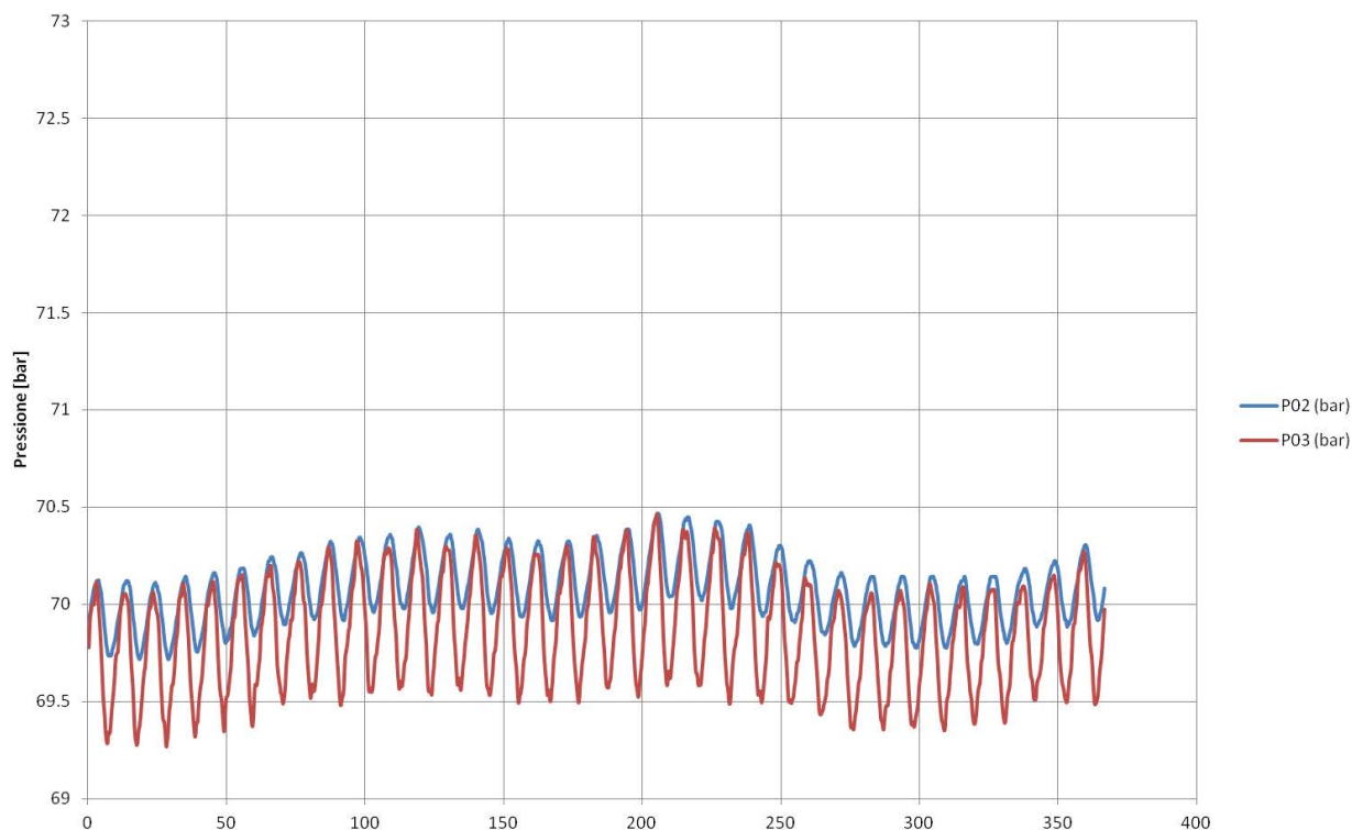
Pressioni in/out vs. tempo - Test 2015
