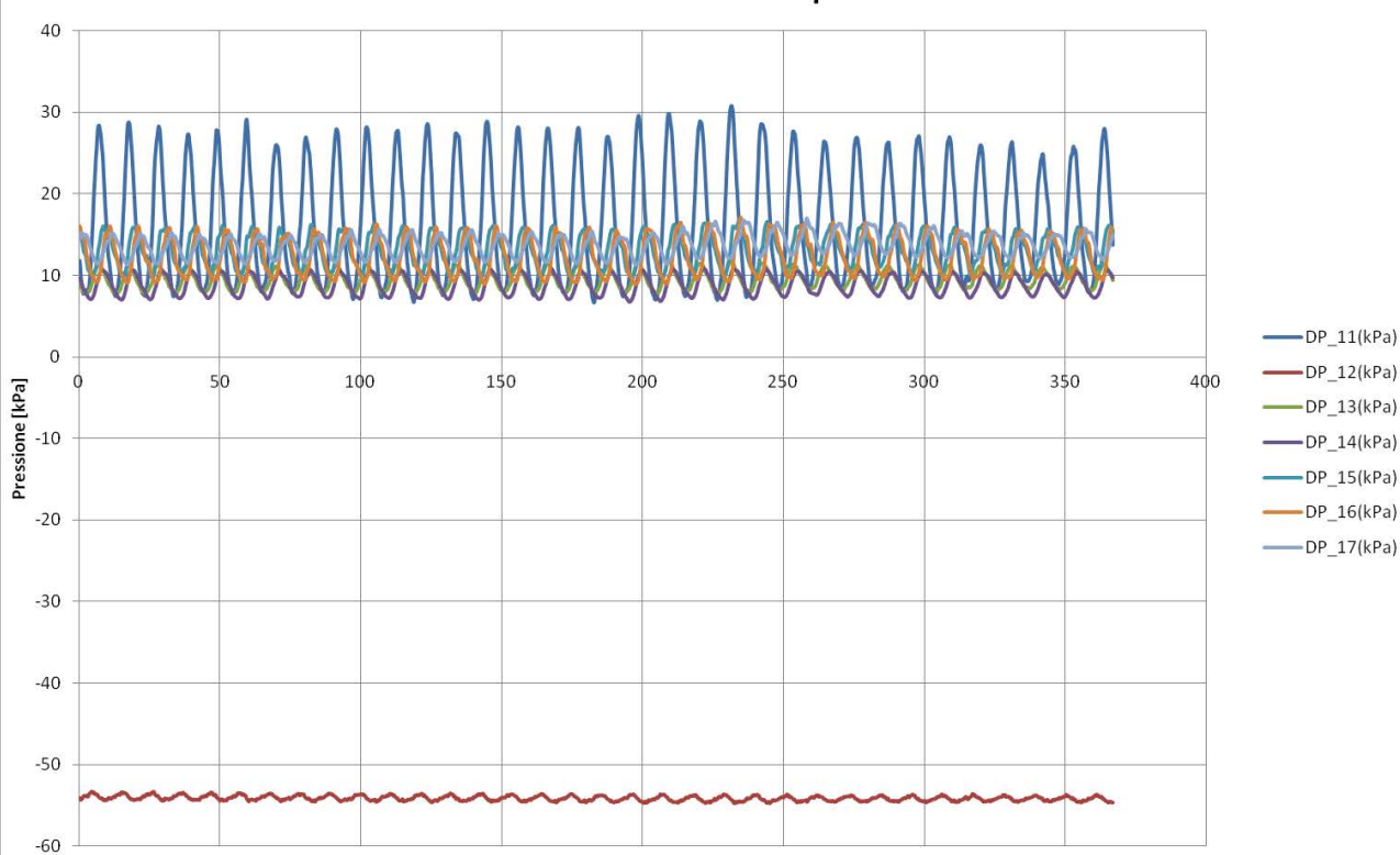
Pressione differenziale vs tempo - Prove 2015
