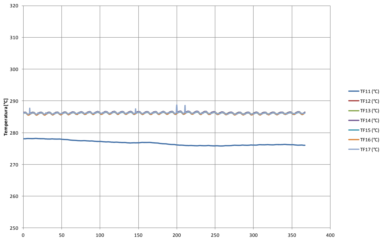
Temperature di fluido vs. tempo - Prove 2015
