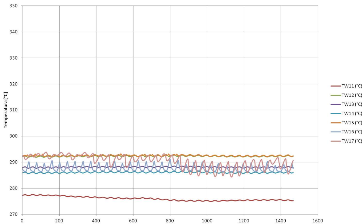
Temperature di parete vs tempo - Prove 2015
