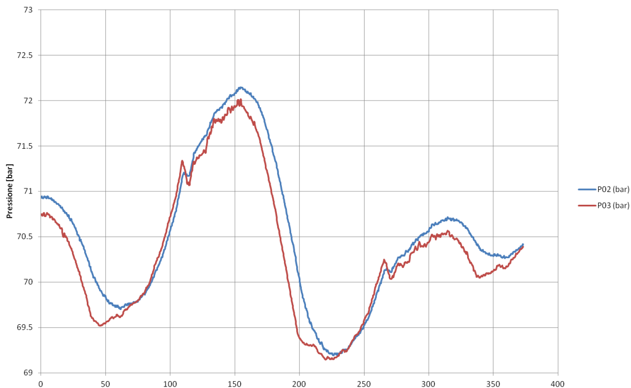
Pressioni in/out vs. tempo - Test 2017
