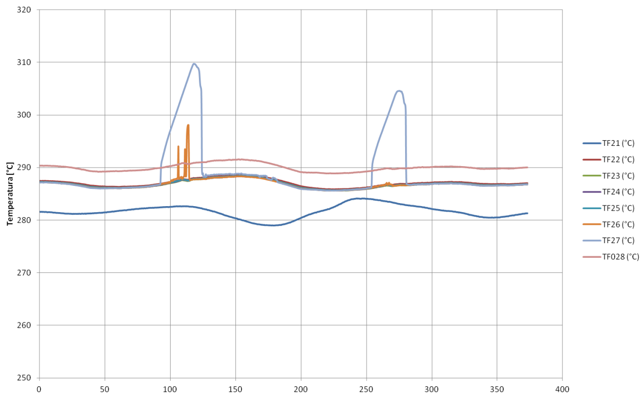
Temperature di fluido vs. tempo - Prove 2017
