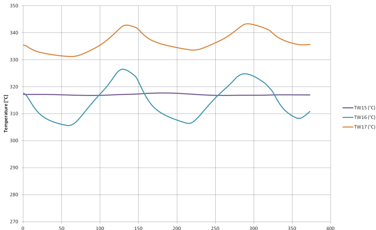
Temperature di parete vs tempo - Prove 2017
