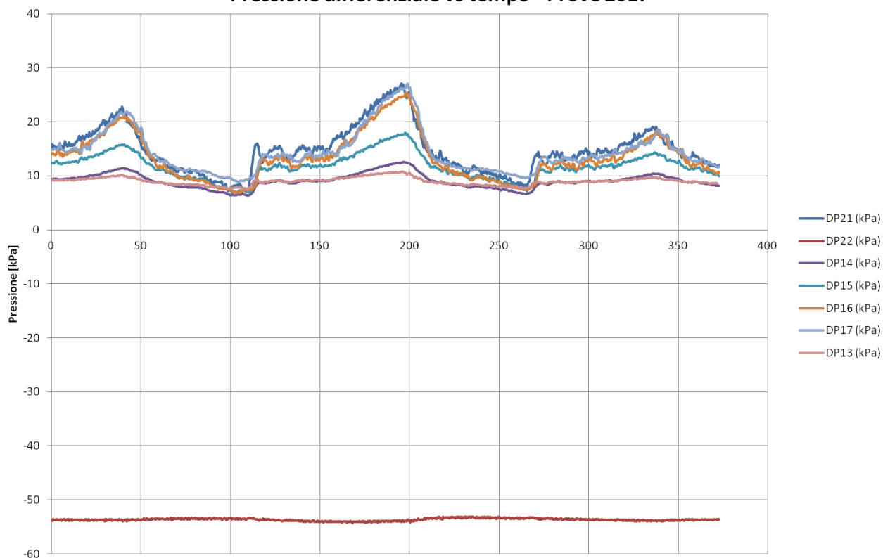
Pressione differenziale vs tempo - Prove 2017
