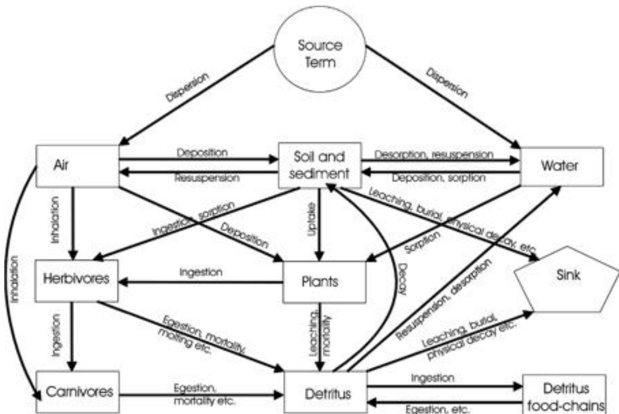
Figura 2. Processi che influenzano il comportamento dei radionuclidi negli ecosistemi (Whicker and Schultz, 1982).
