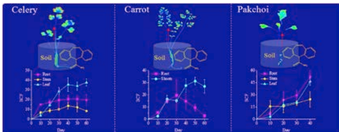
Figura 4. Esempio di trasferimento del C-14 dal suolo ad alcuni tipi di piante (Li et al., 2018).
