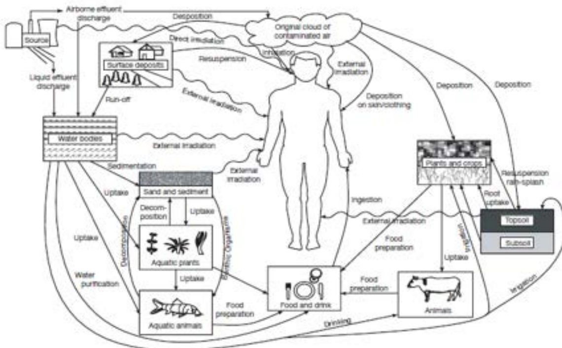
Figura 1. Possibili vie di esposizione della popolazione ai rilasci di radioattività nell'ambiente (IAEA, 2005).
