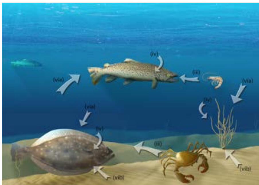
Figura 8. Percorsi di esposizione acquatica per pesci e alghe: (iii) Ingestione di animali con livelli trofici inferiori; (iv) Assorbimento diretto dall'acqua; (vi) Esposizione esterna da (a) acqua e (b) sedimento (ICRP, 2009).
