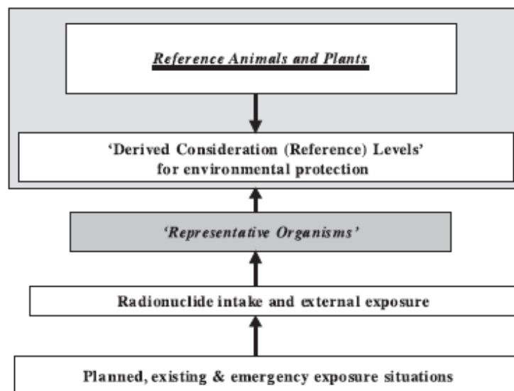
Figura 6. Relazioni tra i vari punti di riferimento per la protezione dell'ambiente (ICRP, 2008).
