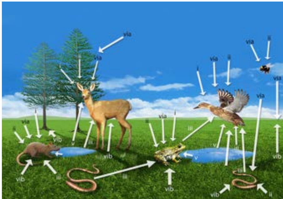
Figura 7. Percorsi di esposizione terrestre: (i) Inalazione di particelle o gas; (ii) Contaminazione di pellicce / piume / pelle; (iii) Ingestione di animali con livelli trofici inferiori; (v) Bere acqua contaminata; (vi) Esposizione esterna attraverso (a) aria o (b) suolo (ICRP, 2009).
