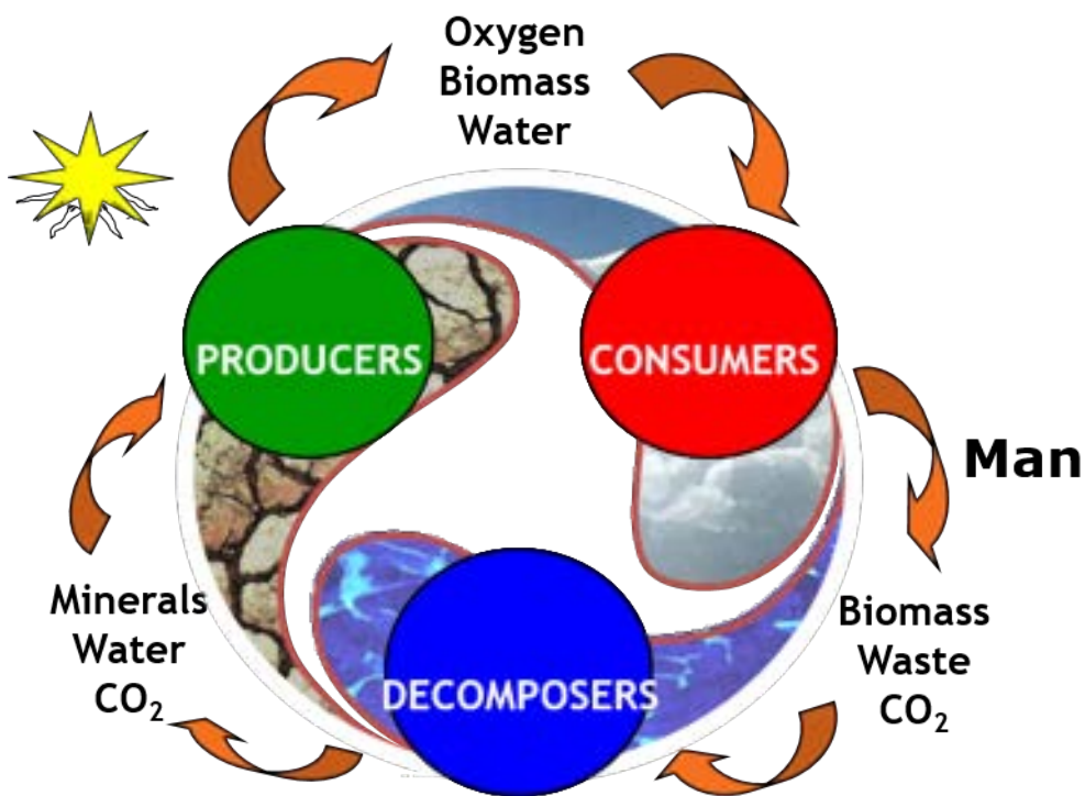
Figura 3. Ciclo della radioecologia.
